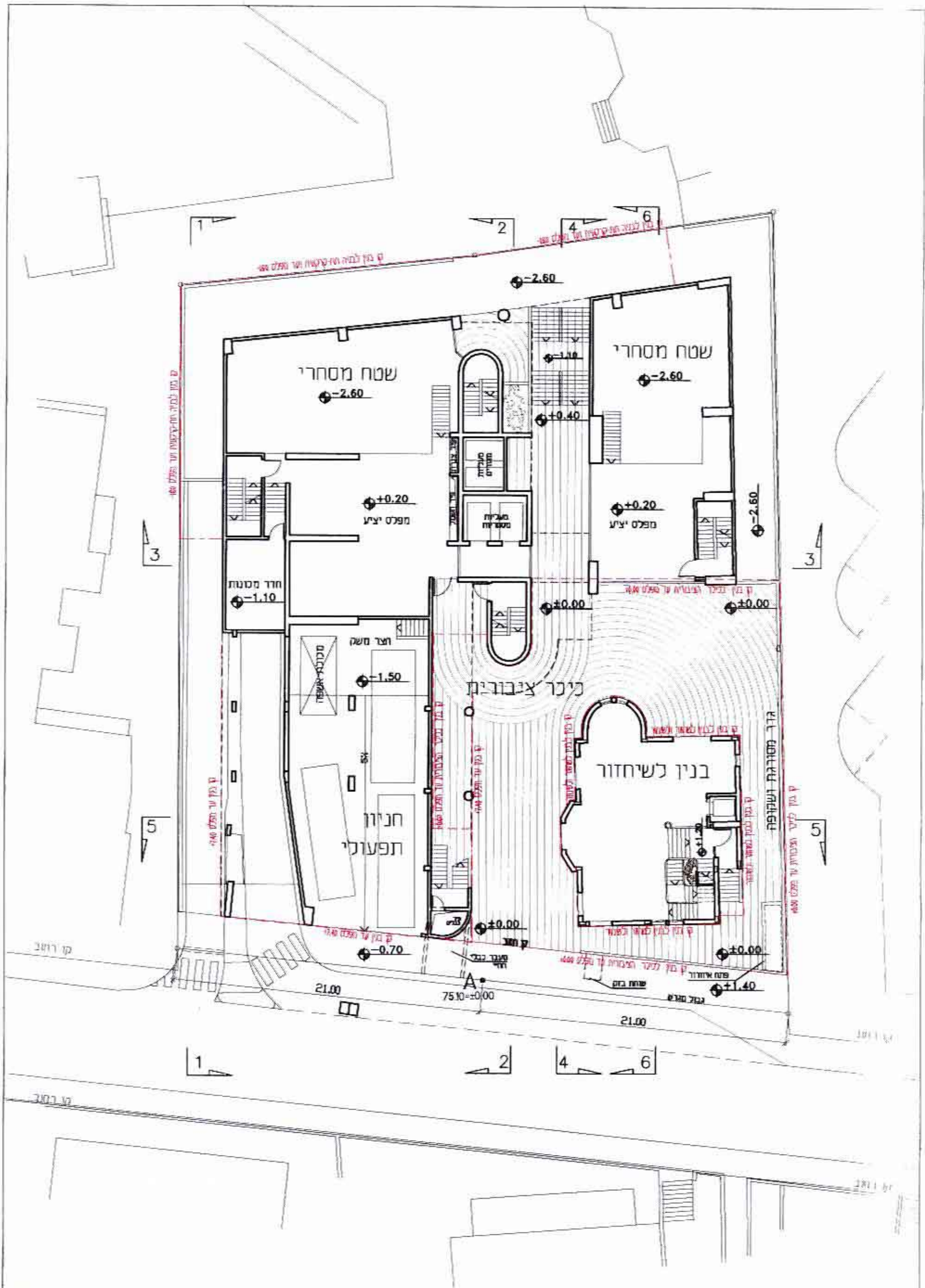
1 : 250 תכנית קומה מסחרית יציע - רח' אחד העם (מפלס +0.20) 7
