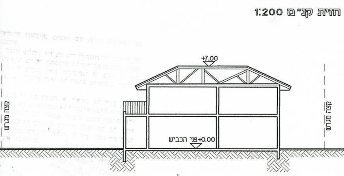
חתך עקרוני קני"מ 1:200
