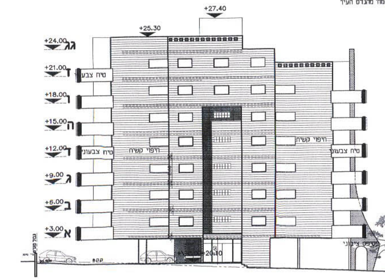
חזית דרומית
