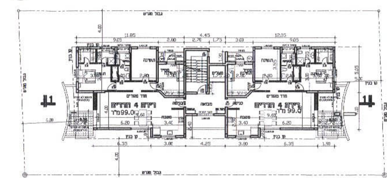
קומה ג'-ה
