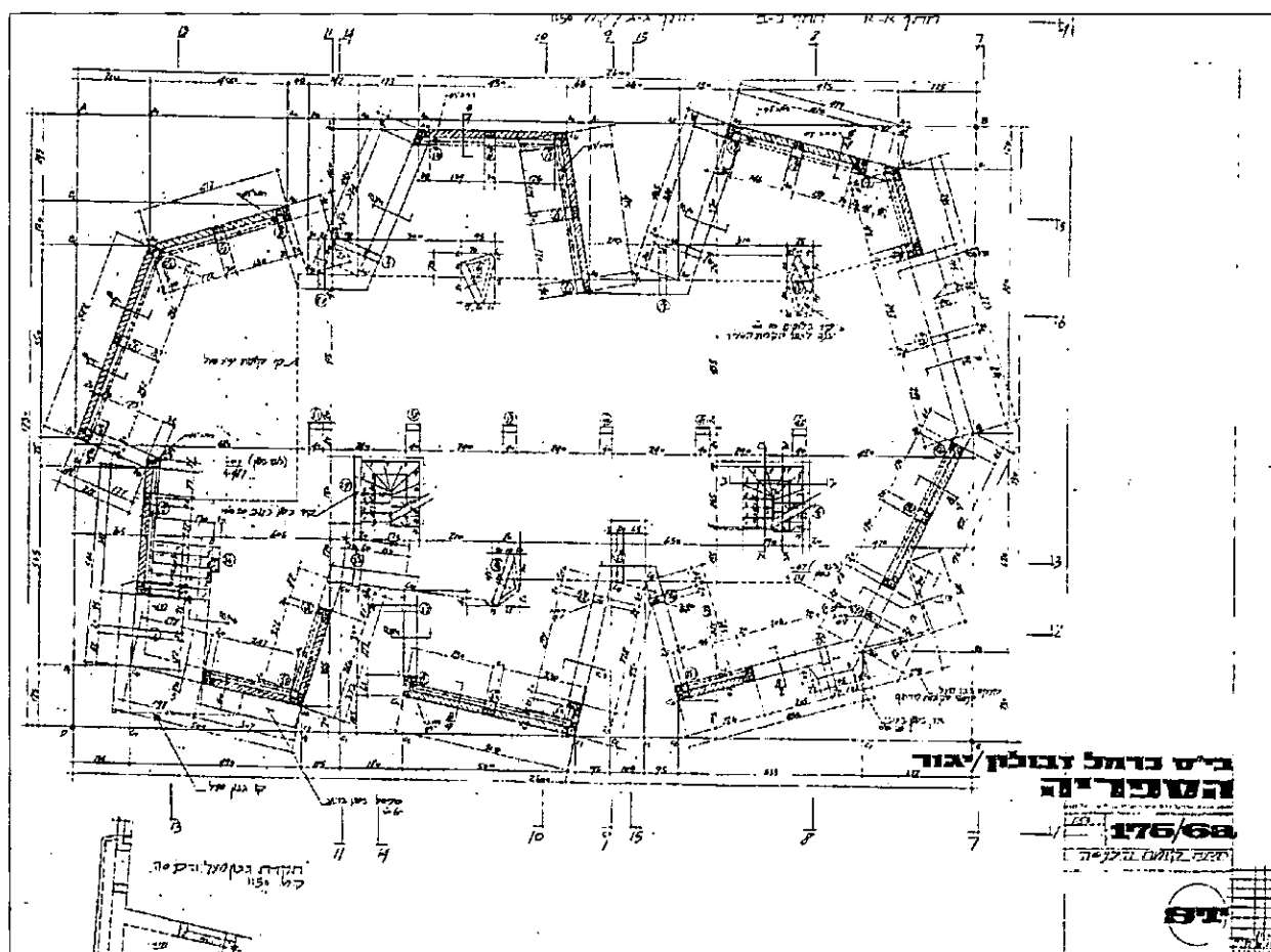
מבנה הספרייה, תוכנית קומת הכניסה, אדריכל שמעון שפירא, 1977
