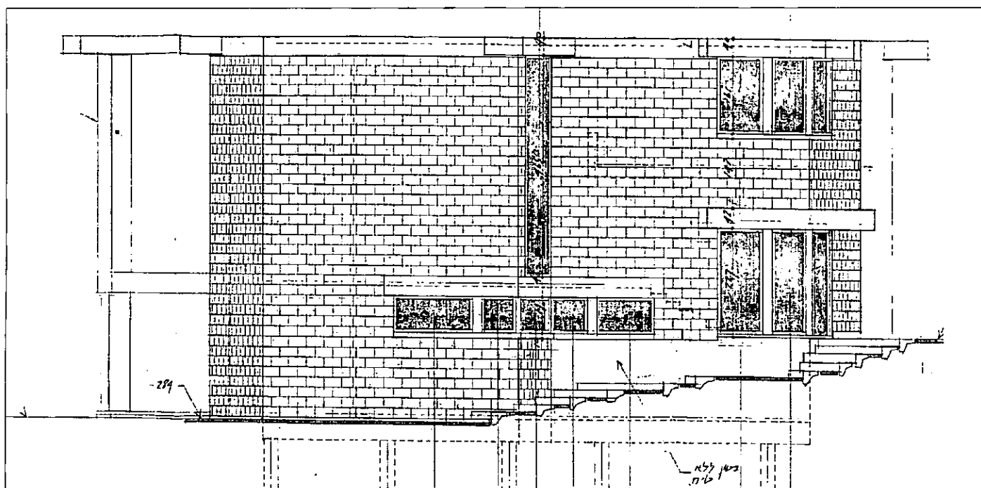
מבנה הספרייה, חזית מערבית, אדריכל שמעון שפירא, 1977
