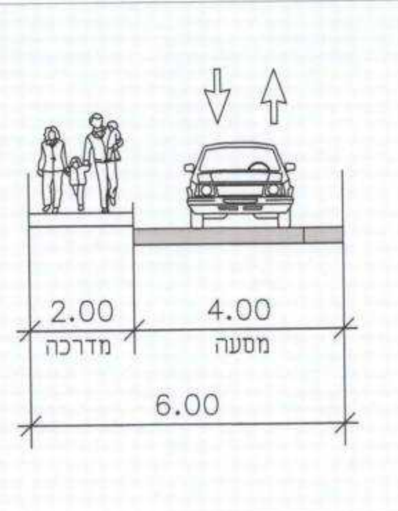
חתך אופייני למעבר כלי רכב קנ"מ 1:100
