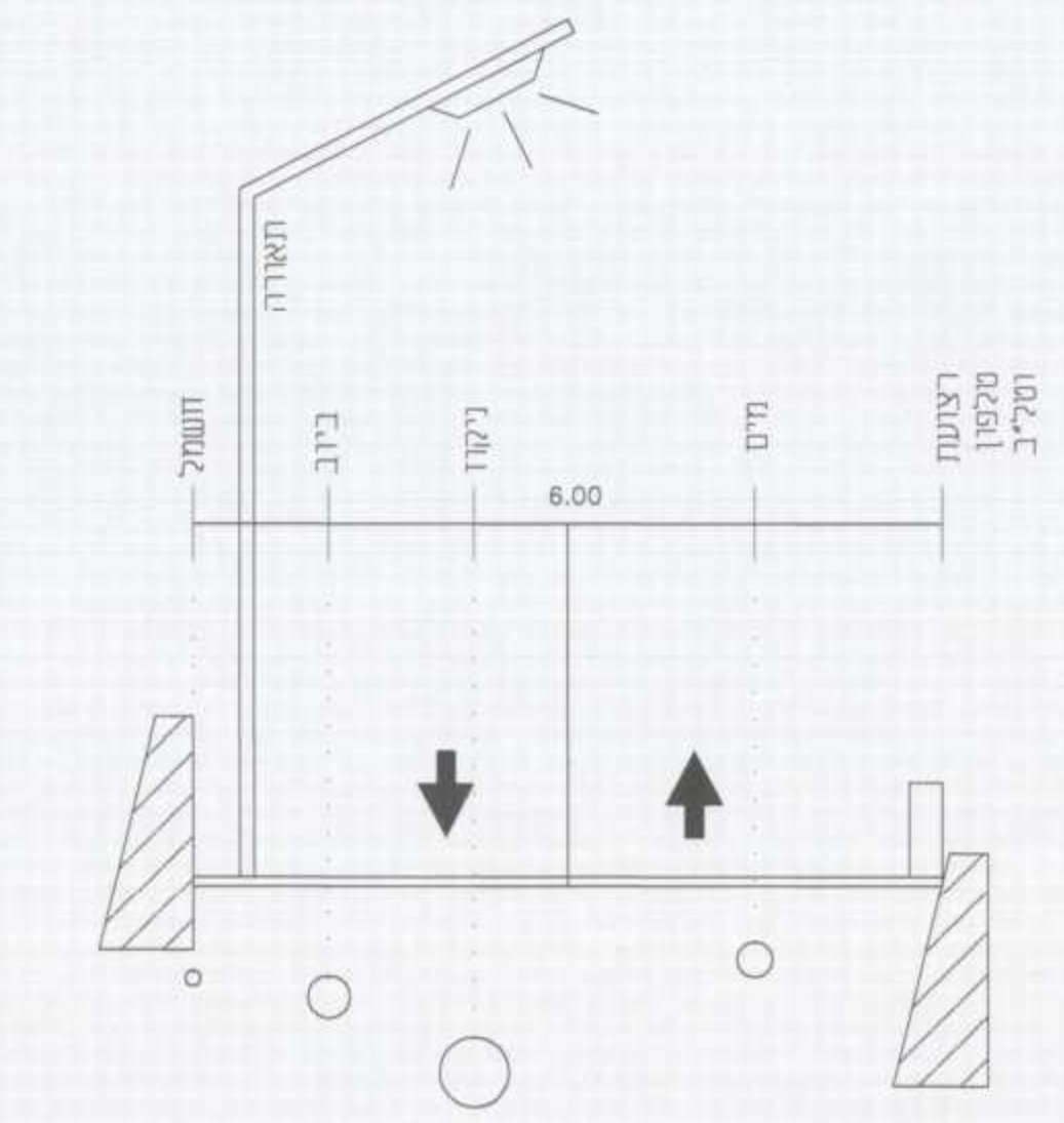
חתך טיפוסי לכביש ברוחב רצועה 6 מטר
