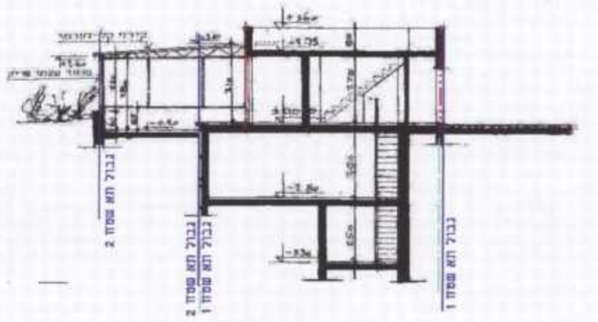
חתך ב-ב 1:200
