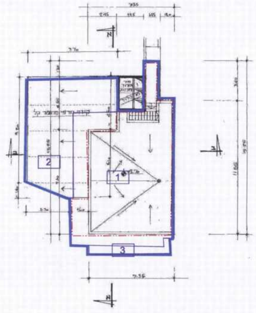
תכנית גג 1:200
