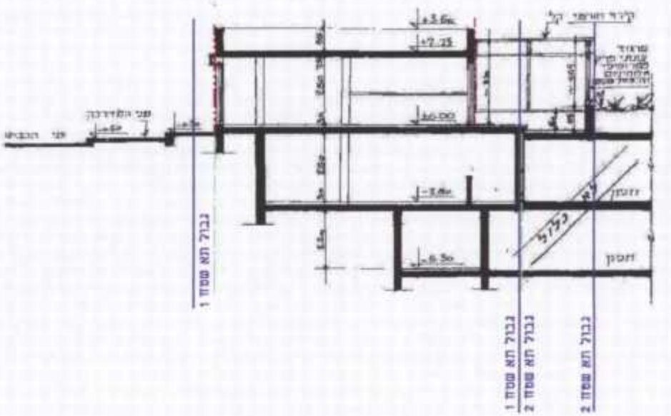
חתך א-א 1:200
