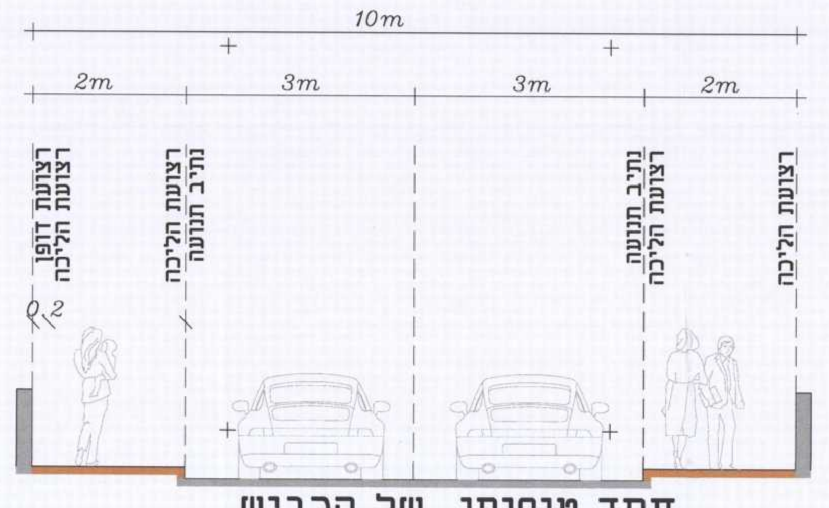
חתך טיפוסי של הכביש קני"מ 1:50 חתך A-A
