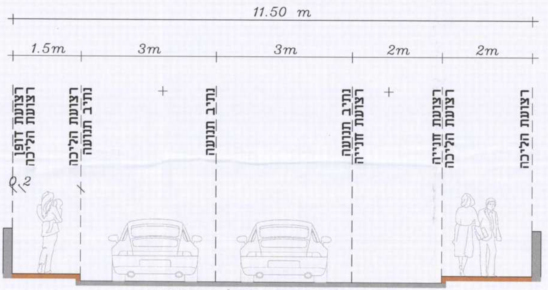
חתך טיפוסי של הכביש קני"מ 1:50 חתך B-B
