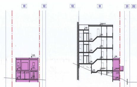
חתך ב-ב - קנ"ח 1:200
