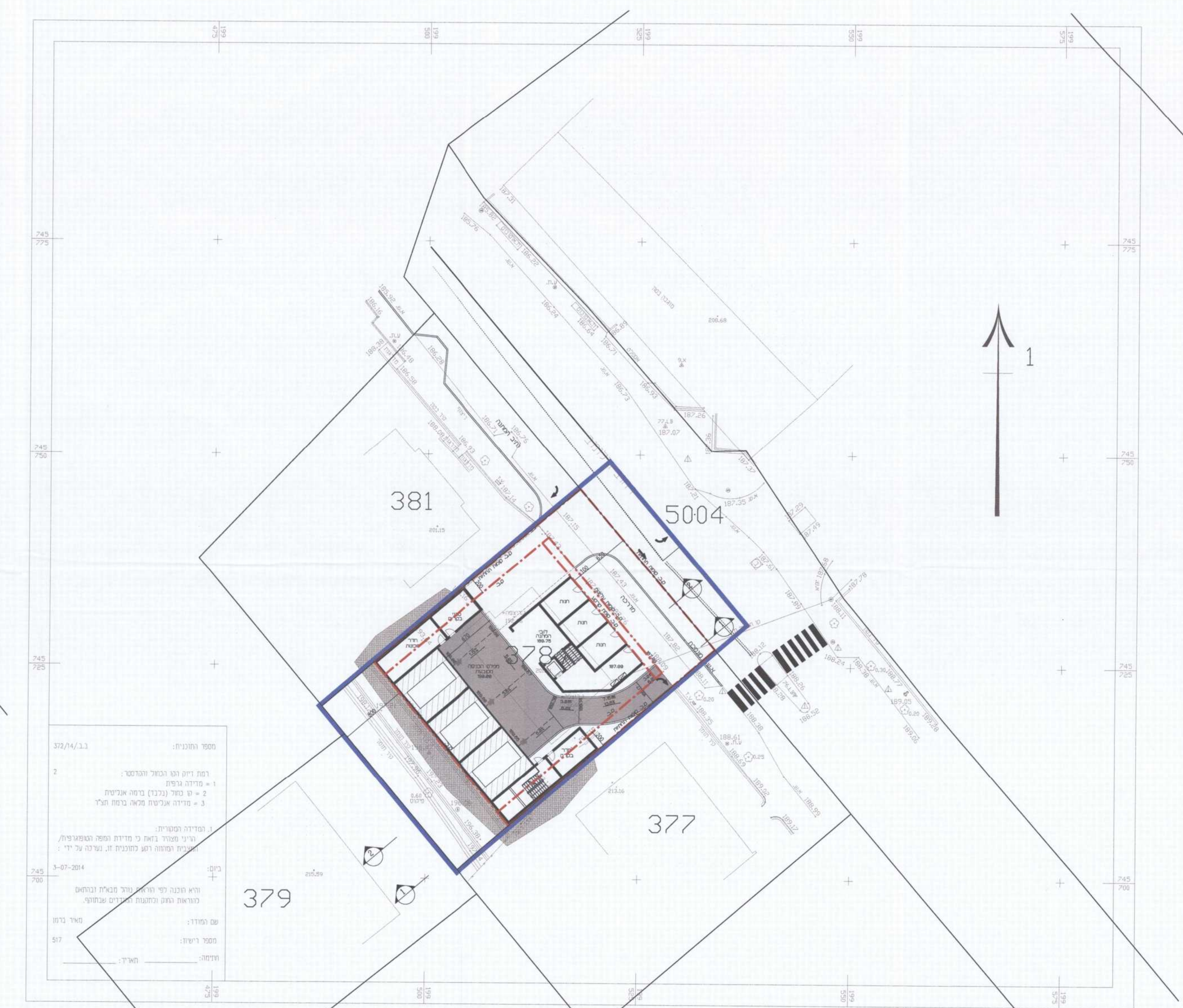
תוכנית קומת כניסה - מפלס יציאת רכבים קנ"מ 1:250
