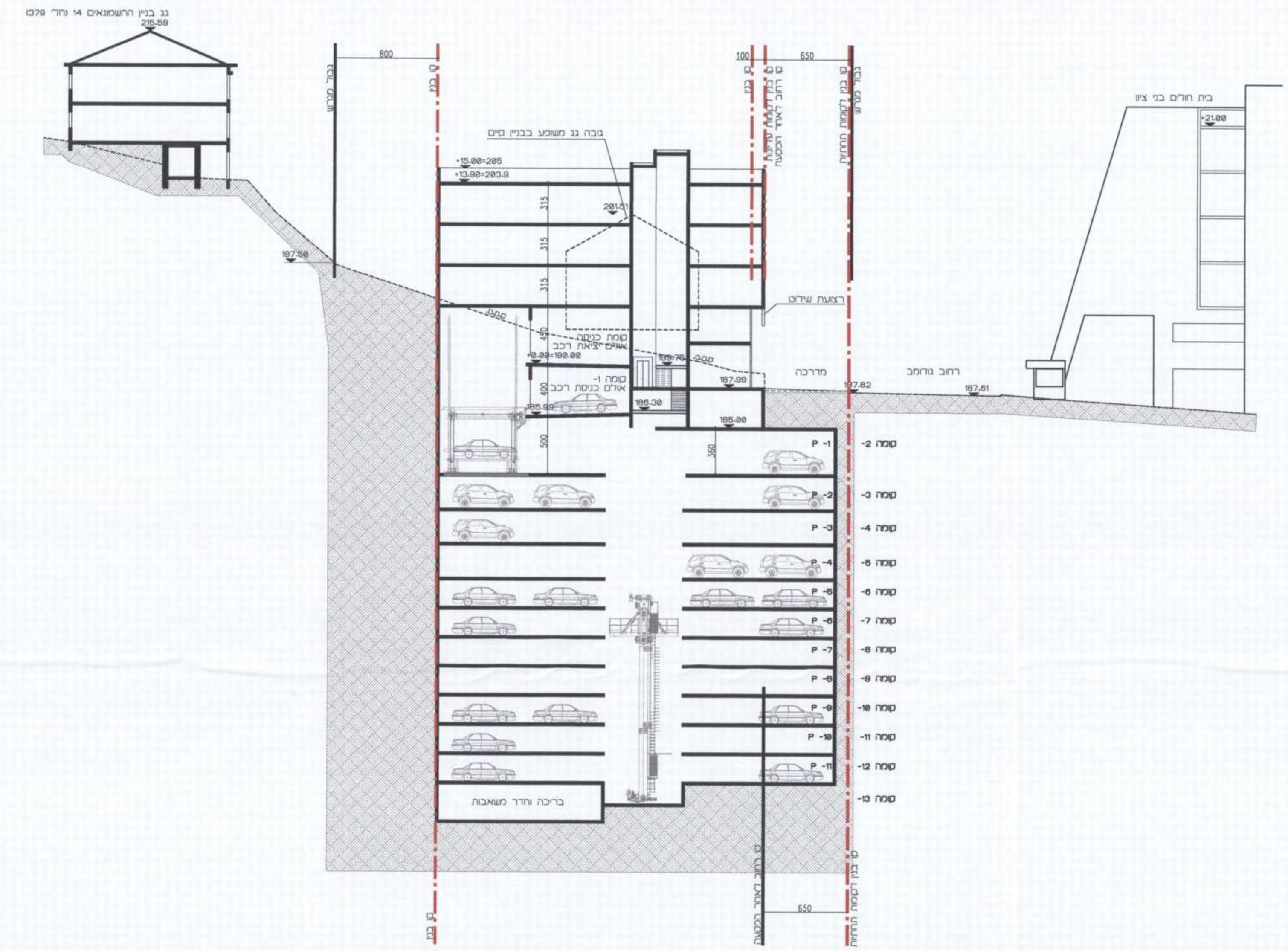
חלופה ב': חלופה ב': מבנה למסחר/מרפאות/ משרדים חתך 2-2 קנ"מ 1:250
