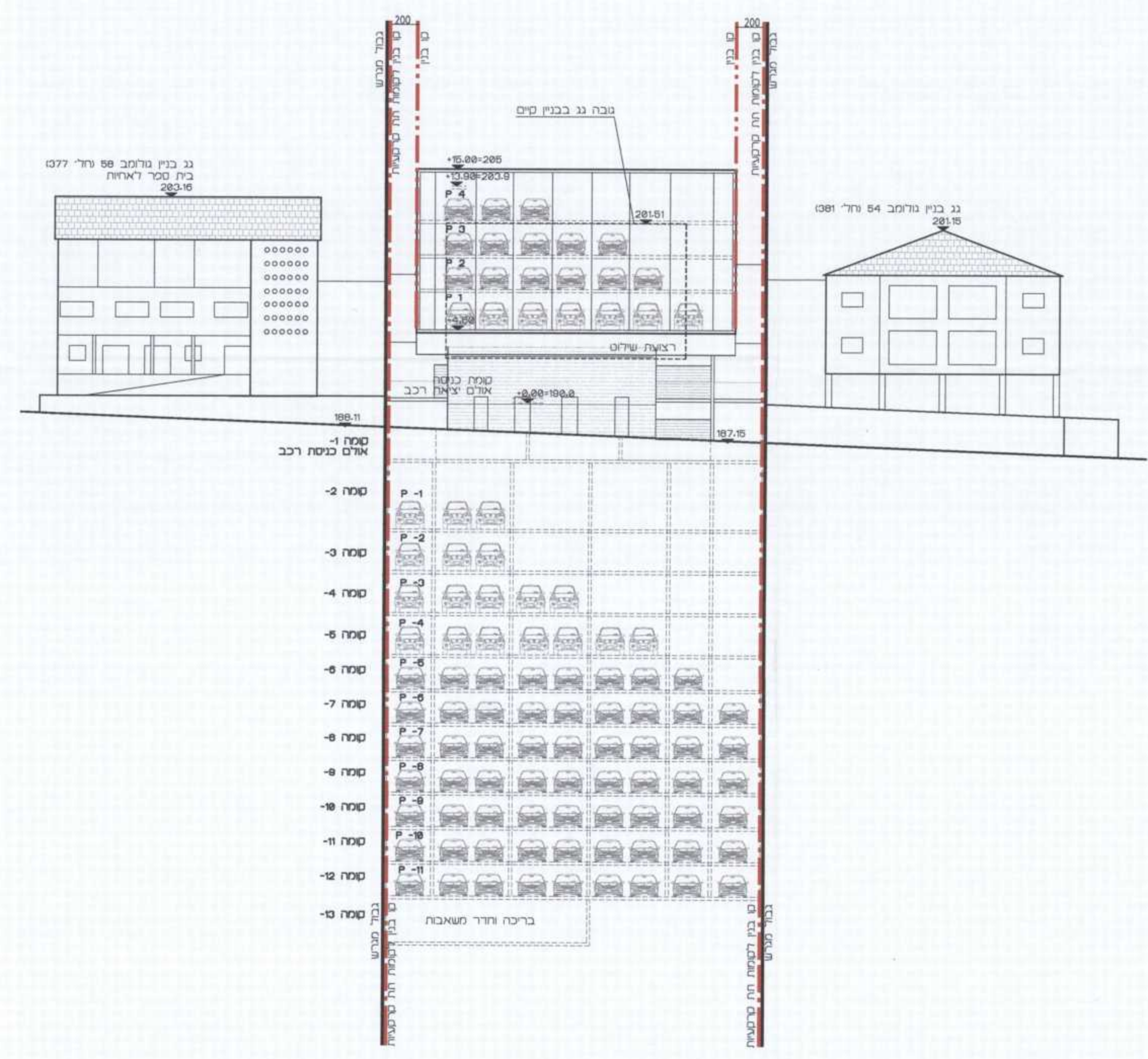
חלופה א': חניון רבובטי חזית צפונית לרח' גולומב קנ"מ 1:250
