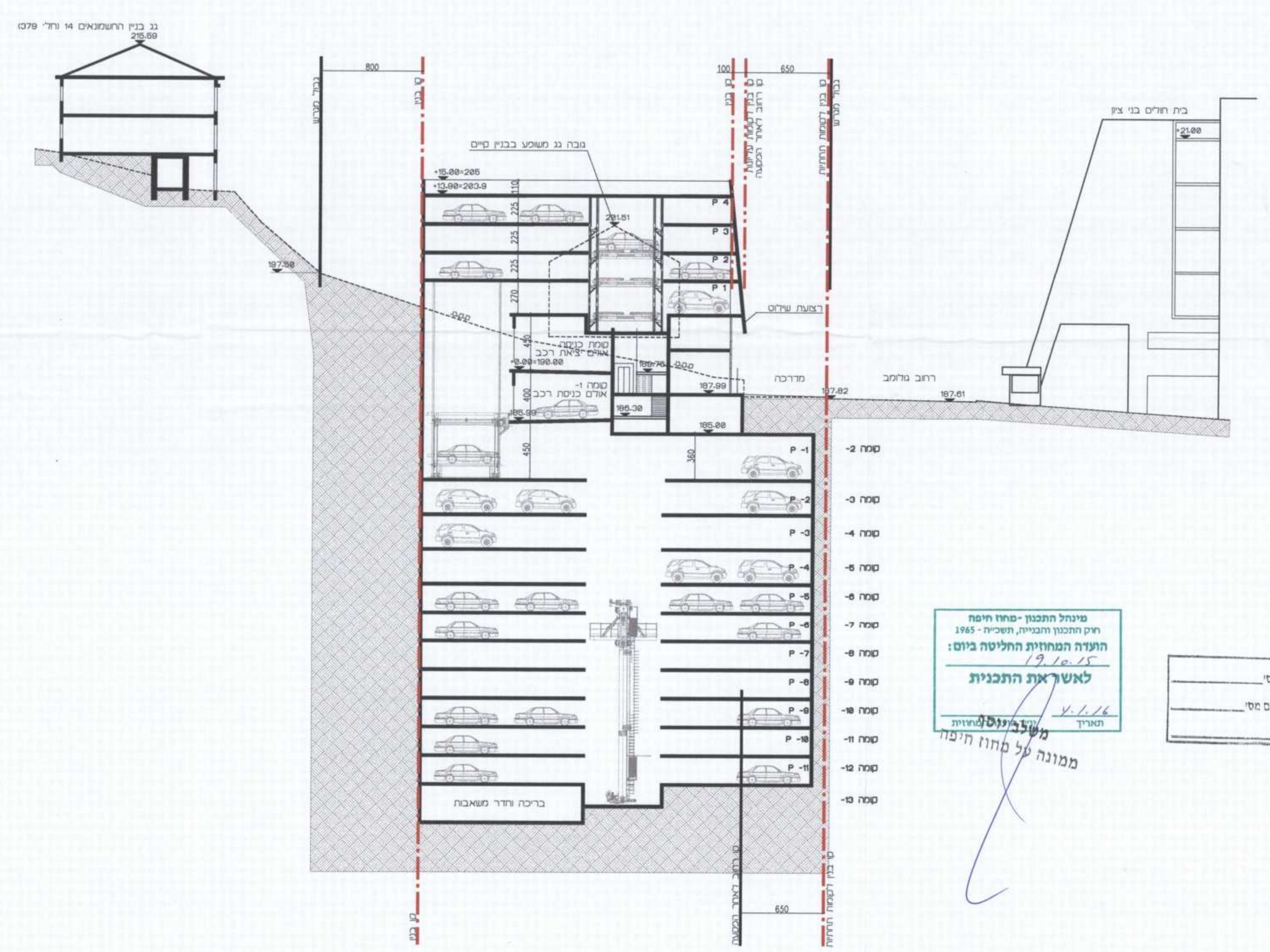
חלופה א': חניון רבובטי חתך 2-2 קנ"מ 1:250
