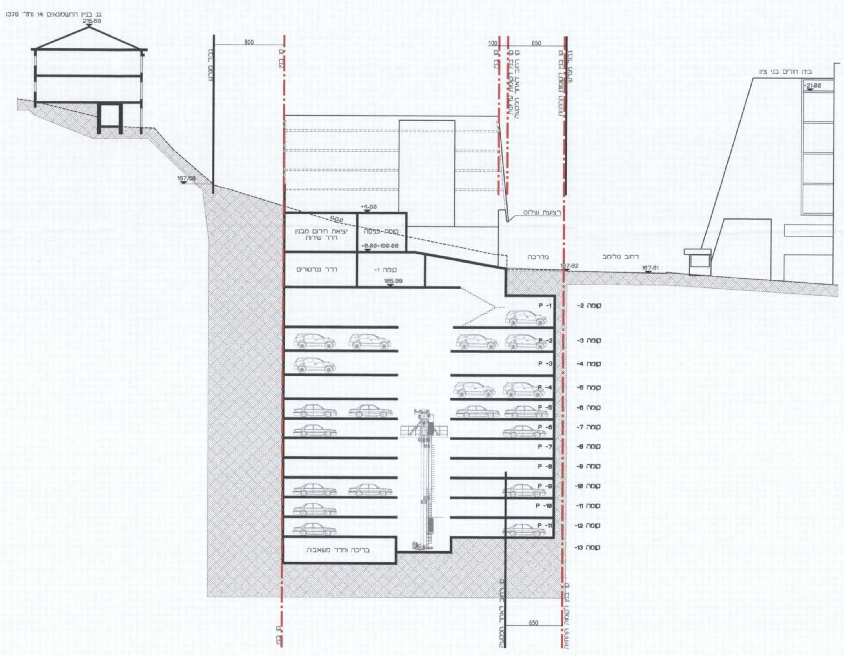
חלופה א': חניון רבובטי חתך 1-1 קנ"מ 1:250
