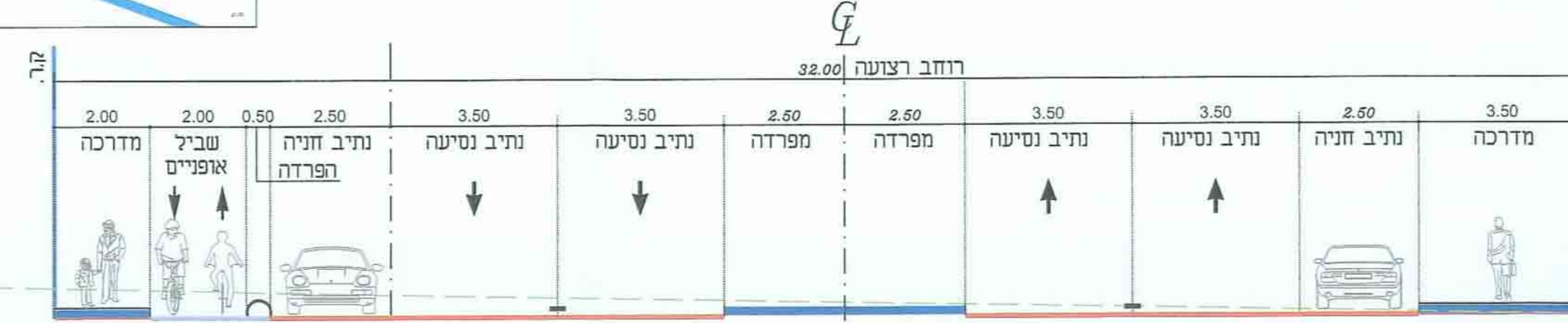
חתך טיפוס ג-ג רוחב כביש 32 מ' כולל שביל אופניים קני"מ 1:100
