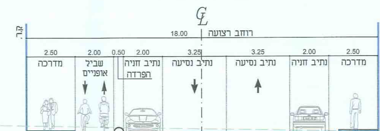
חתך טיפוס א-א רוחב כביש 18 מ' כולל שביל אופניים קני"מ 1:100
