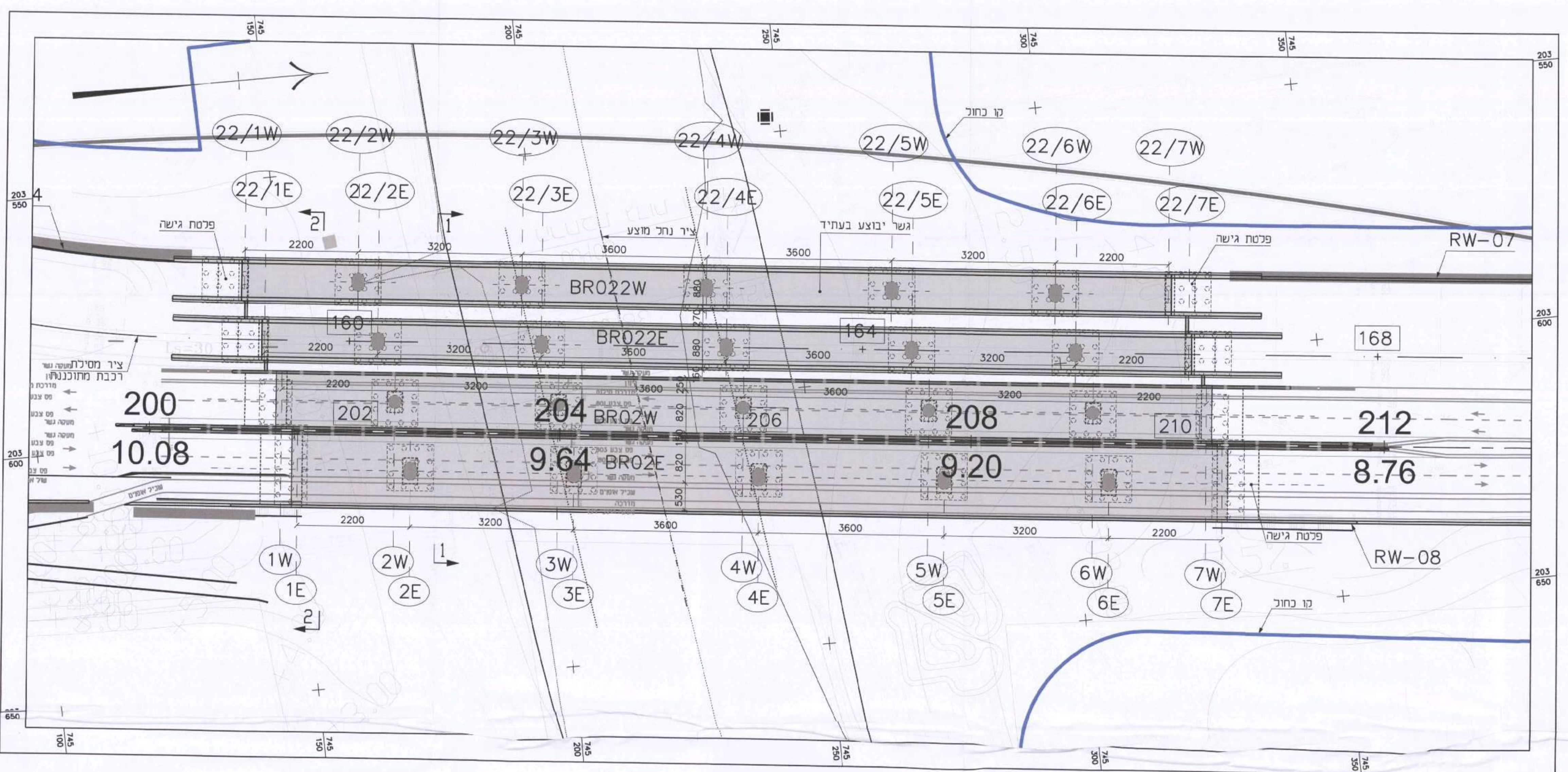
תנוחה 1:500
