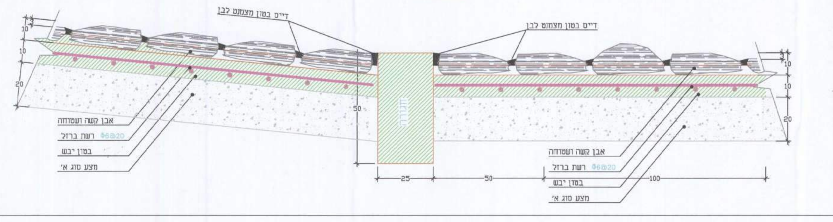
פרט חתך בריח קני"מ 1:10
