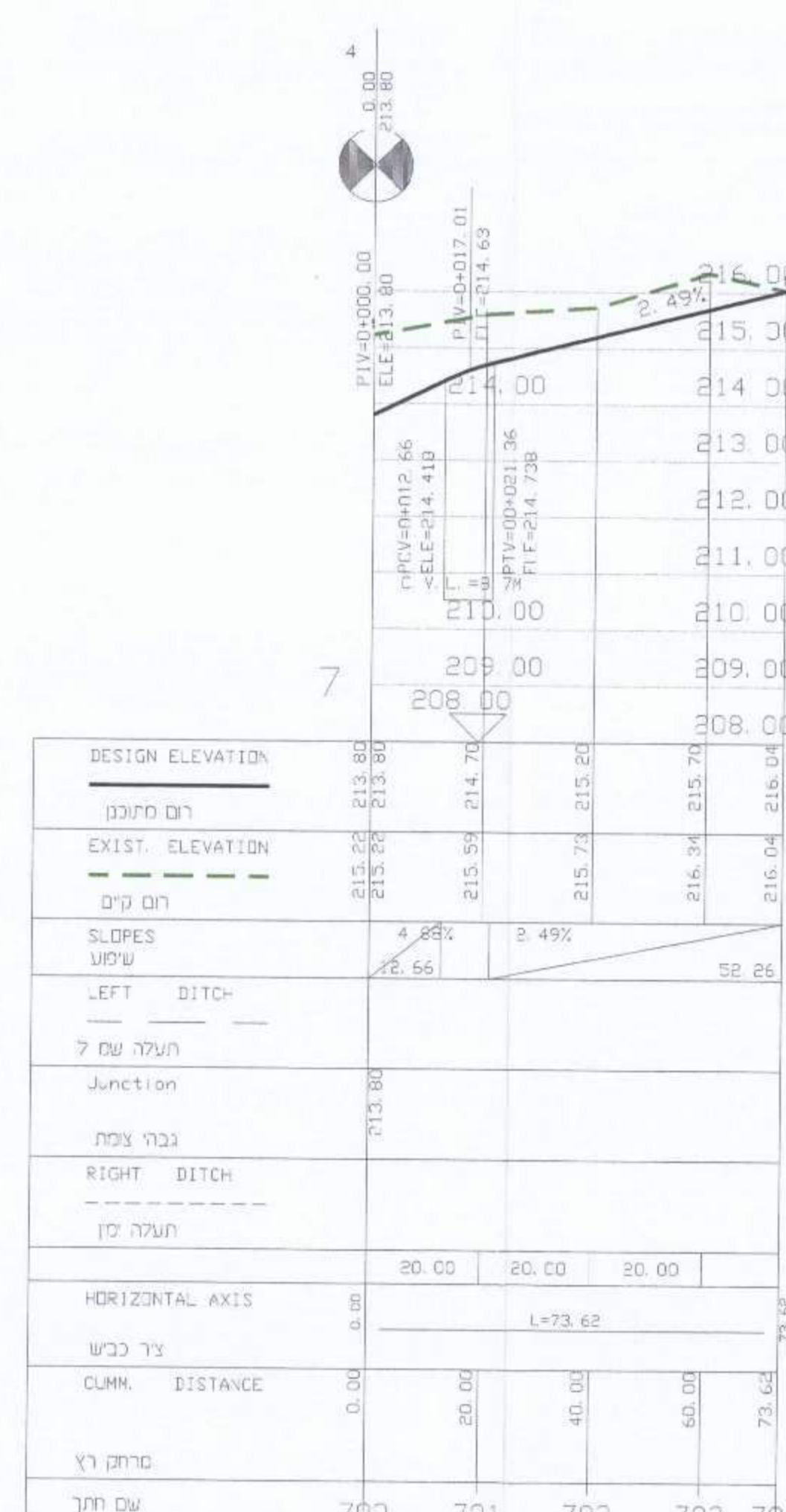
חתך לאורך כביש מס' 13 1:100 / 1:1000
