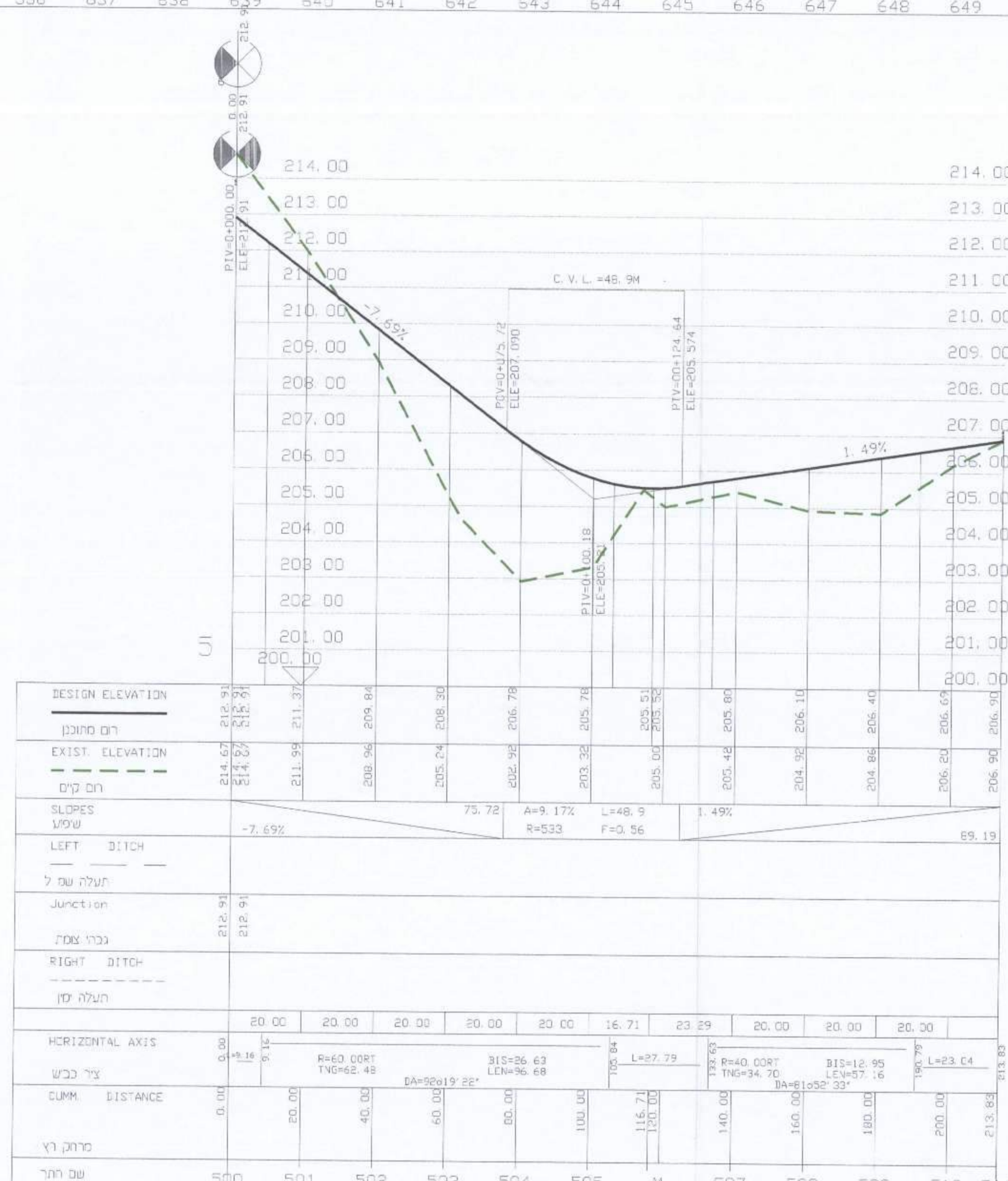
חתך לאורך כביש מס' 10 1:100 / 1:1000
