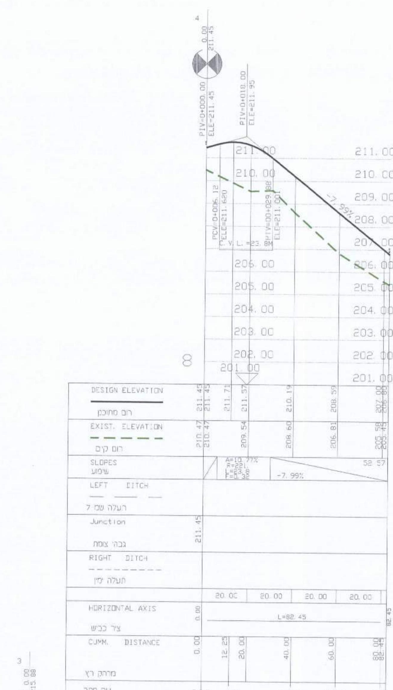
חתך לאורך כביש מס' 14 1:100 / 1:1000
