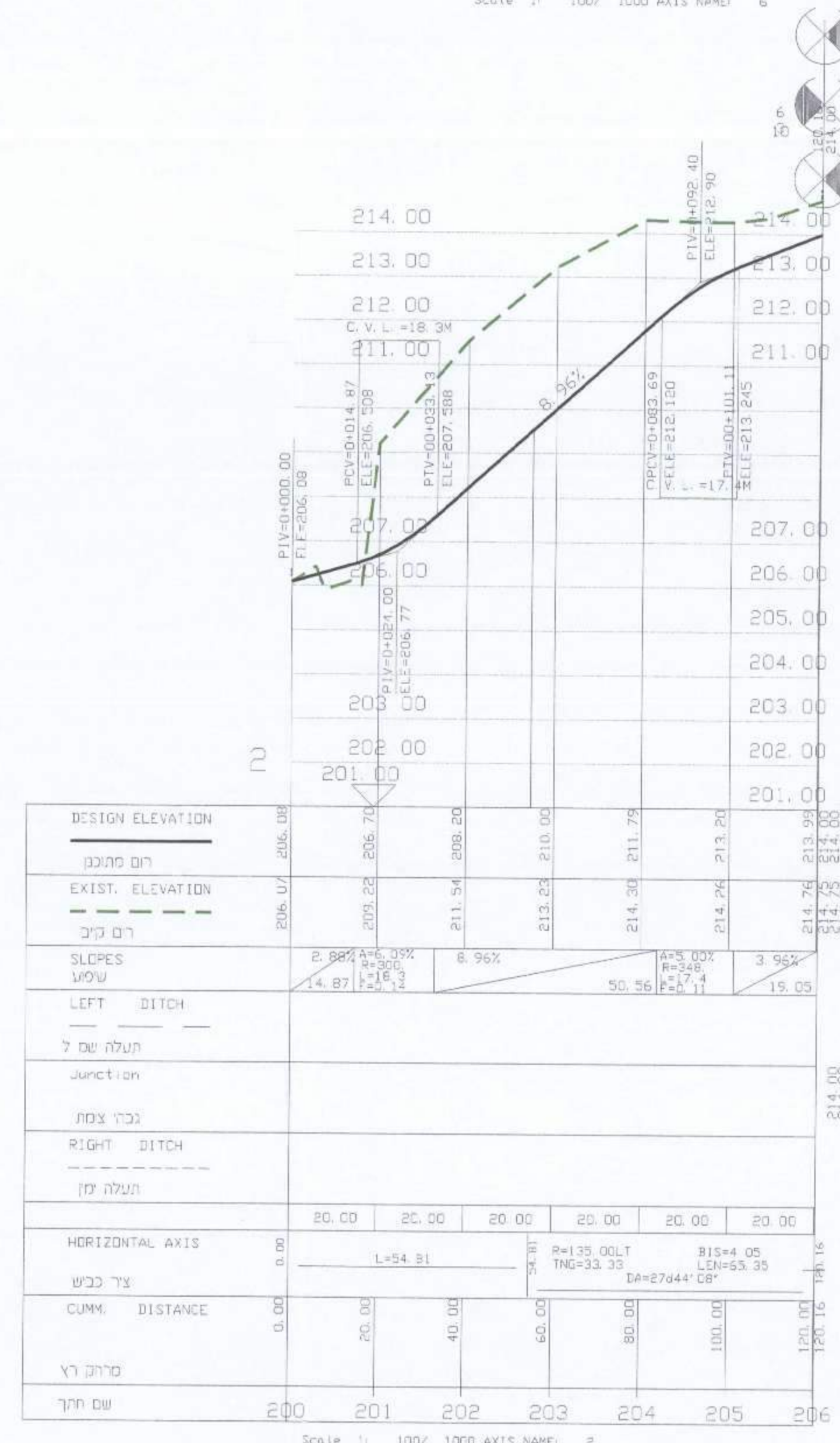
חתך לאורך כביש מס' 7 1:100 / 1:1000
