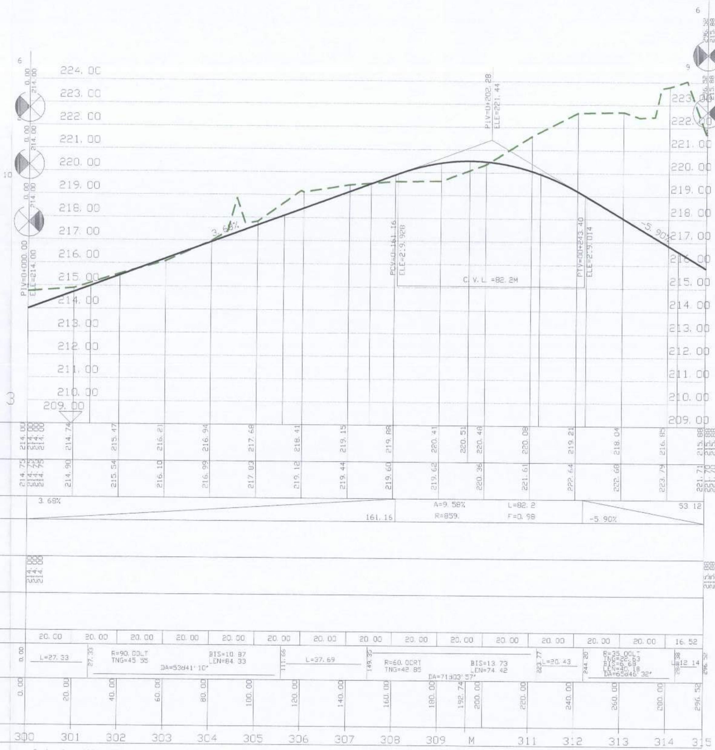
חתך לאורך כביש מס' 8 1:100 / 1:1000
