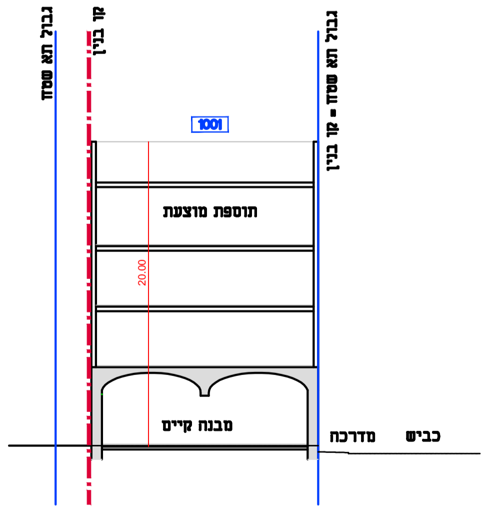
חתך 1-1 מבנה קיים
