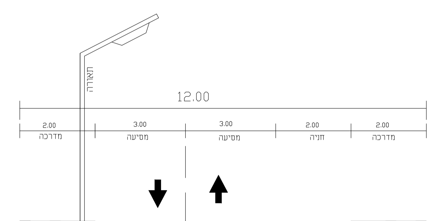
חתך טיפוסי לכביש ברוחב רצועה 12 מטר עם הרחבה
