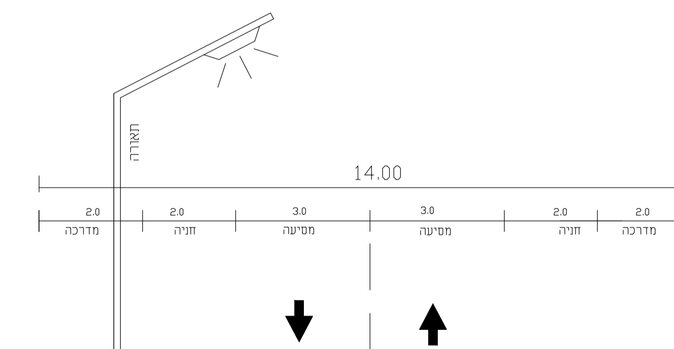
חתך טיפוסי לכביש ברוחב רצועה 14 מטר
