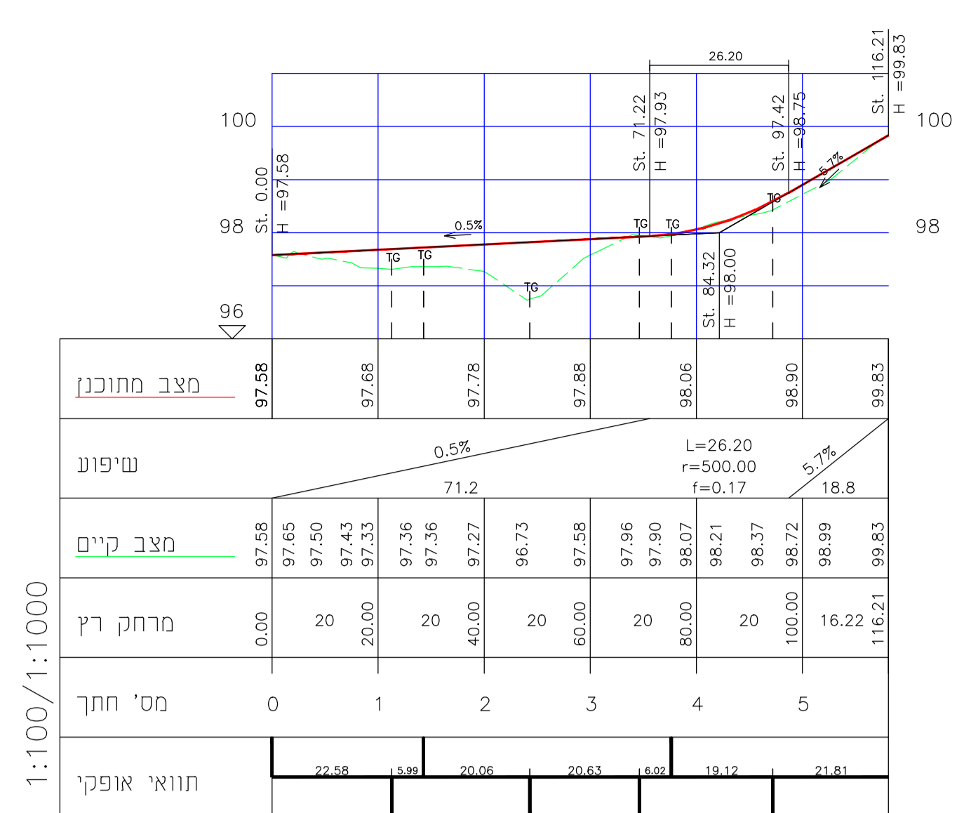
חתך לאורך-קנ"מ 1:100:1000
