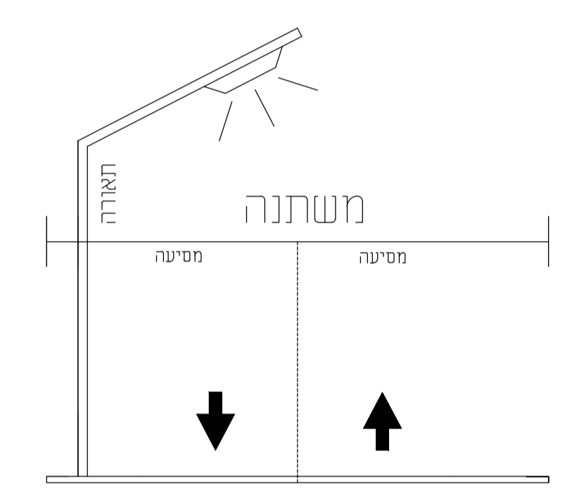
חתך טיפוסי לכביש ברוחב משתנה בלי חזיה למסעה מאבן משתלבת
