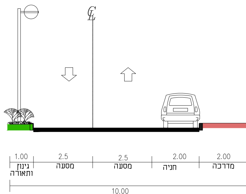
חתך טיפוסי 10 מ' קנ"מ 1:100
