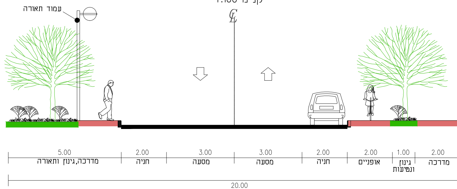
חתך טיפוסי 20 מ' קנ"מ 1:100
