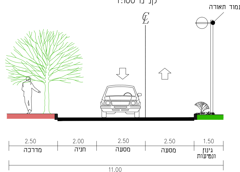
חתך טיפוסי 11 מ' קנ"מ 1:100
