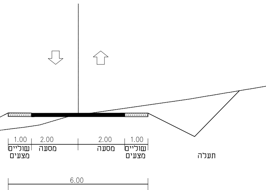
חתך טיפוסי 6 מ' דרכי גישה לת.שאיבה קנ"מ 1:100
