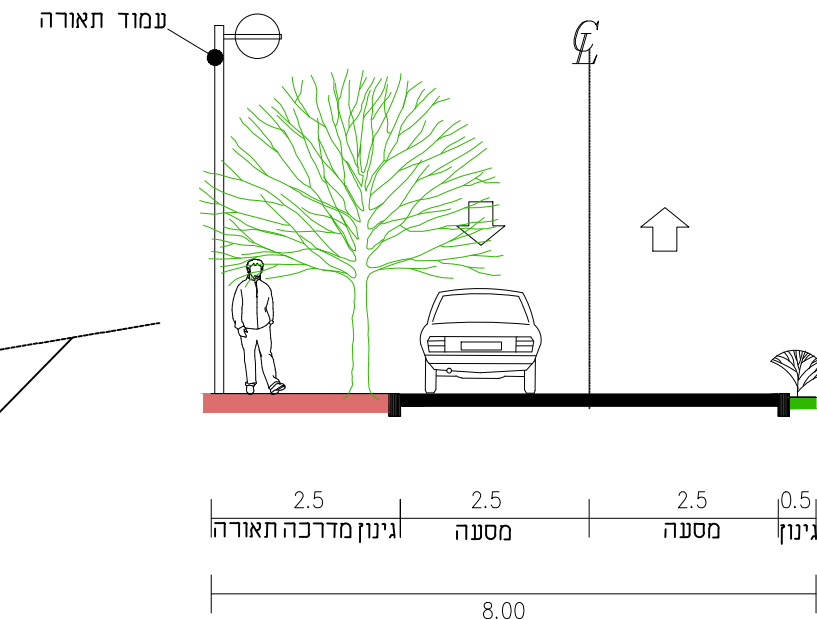
חתך טיפוסי 8 מ' קנ"מ 1:100
