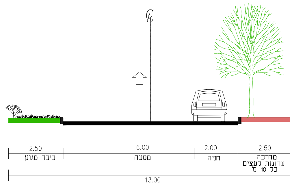
חתך טיפוסי-חד סיפרי 13 מ' קנ"מ 1:100
