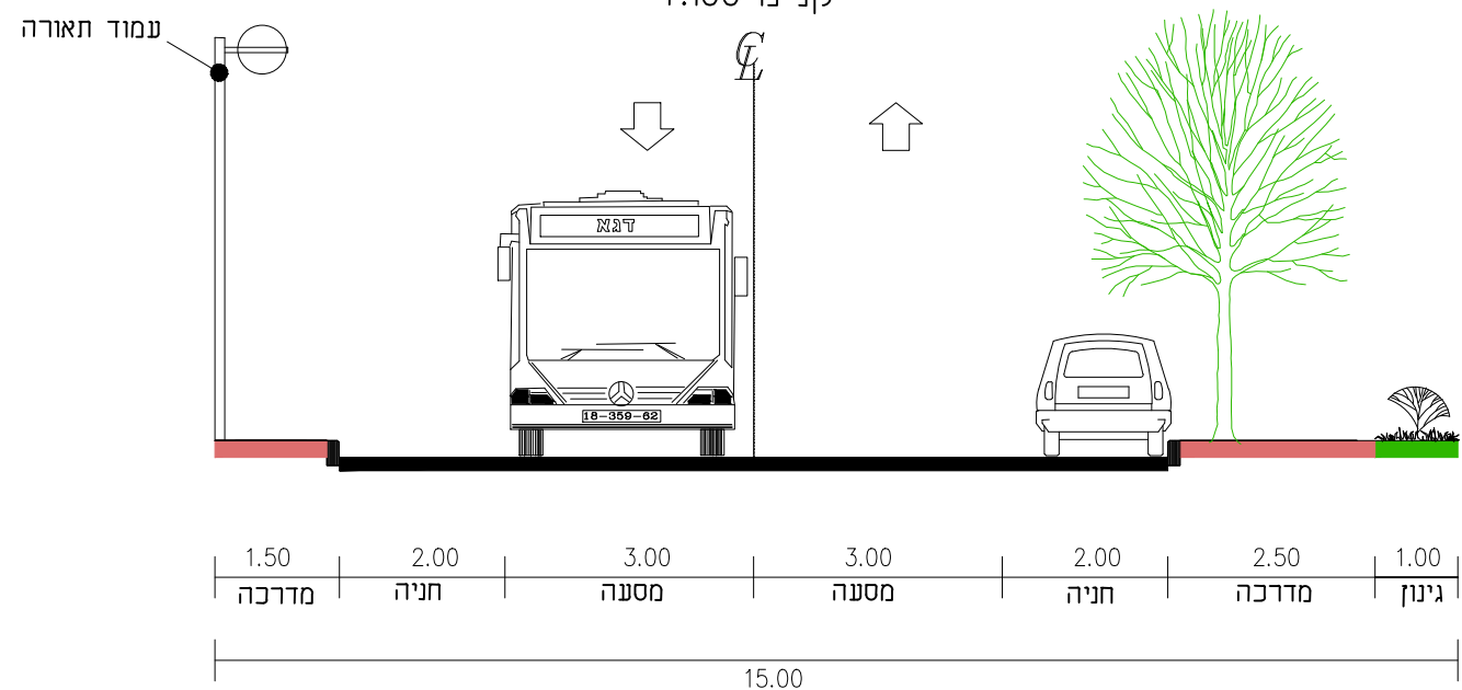
חתך טיפוסי 15 מ' קנ"מ 1:100
