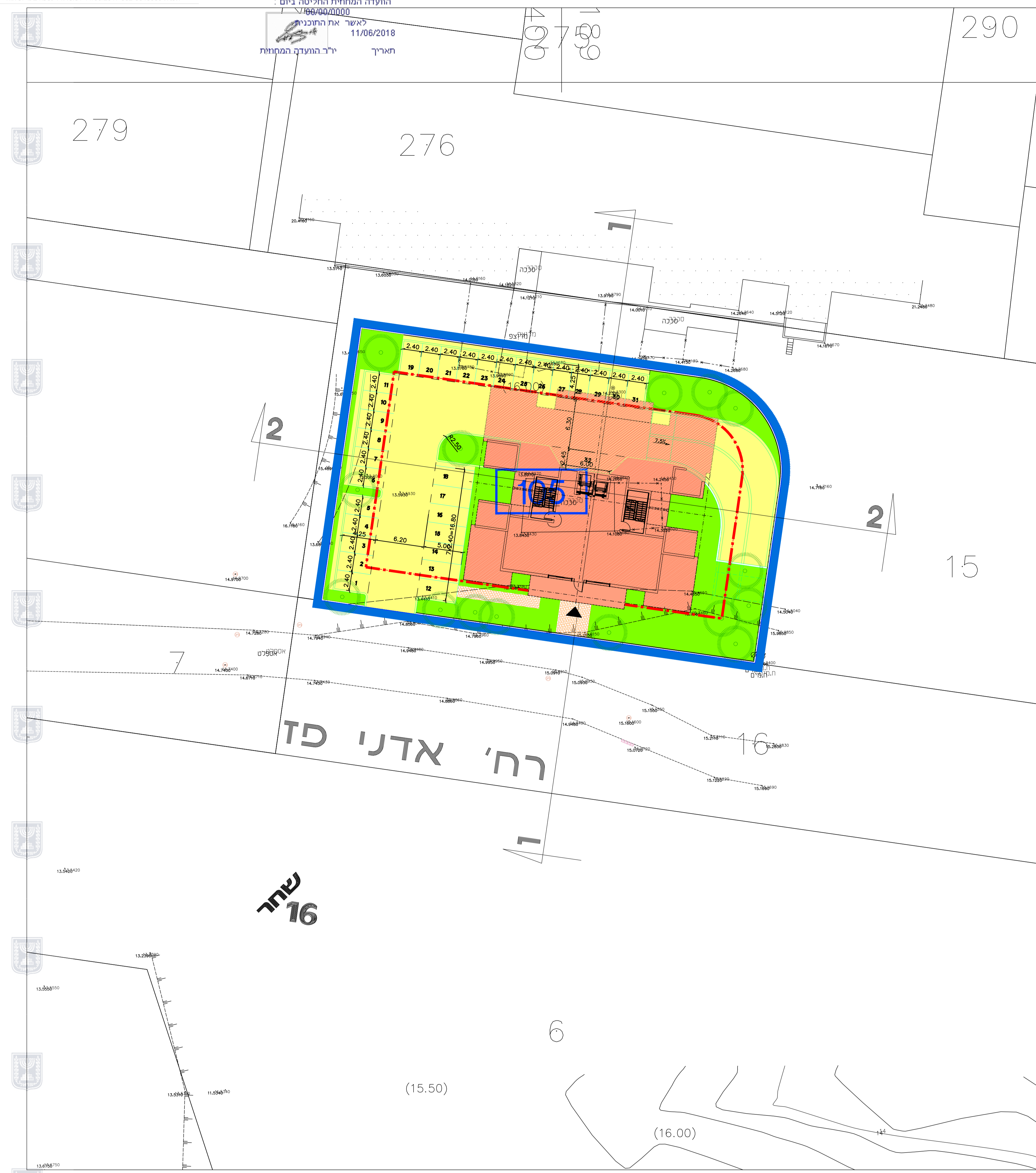
בנין ק.מ. 1:250
