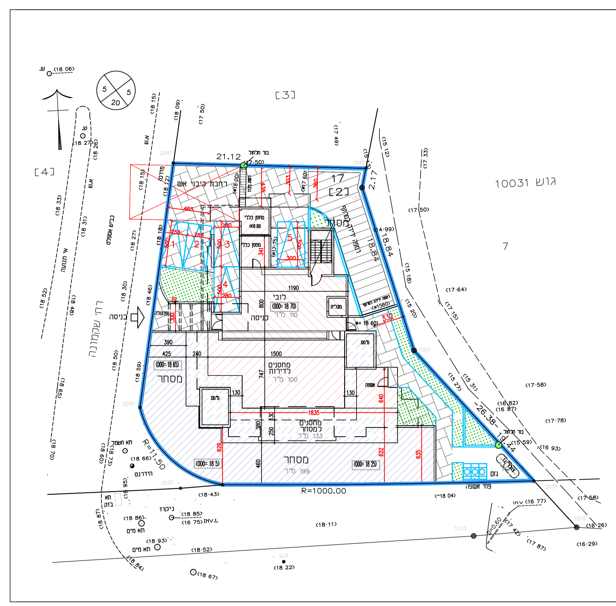
תכנית קומת קרקע 1 : 250 לובי כניסה לבנין מחסנים ואזור מסחר
