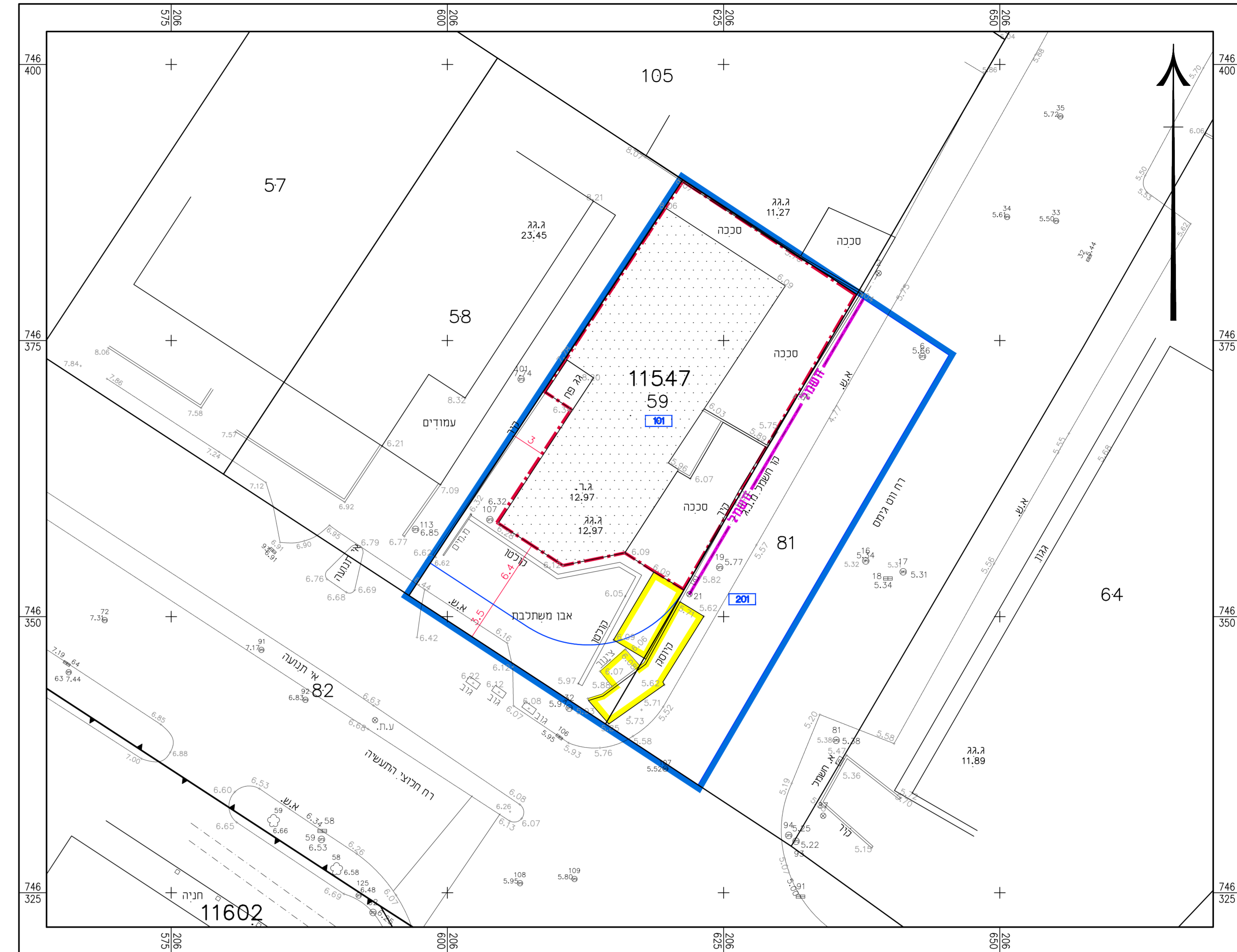
תכנית החלקה - קני"מ 1:250
