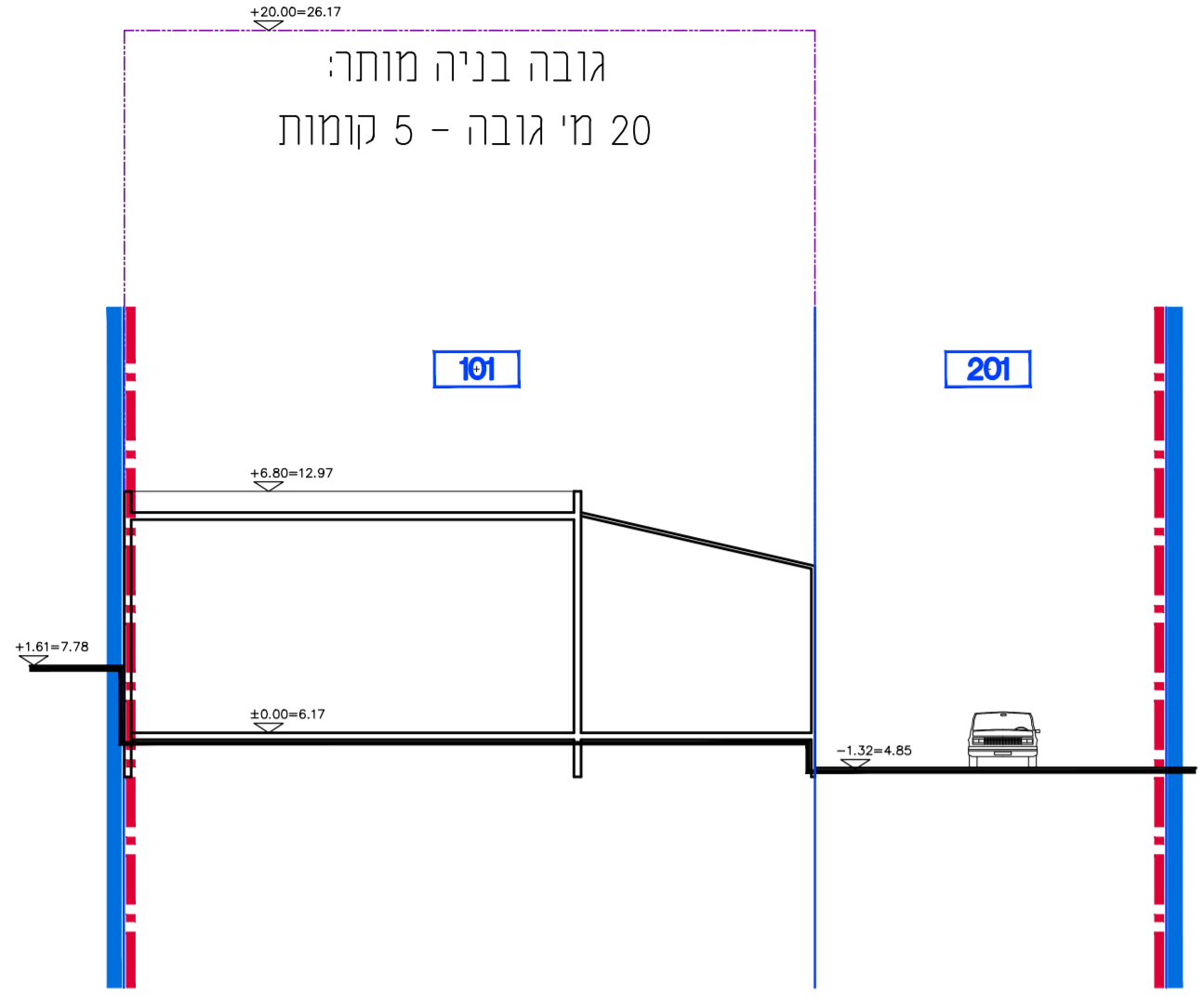
חתך א-א - קני"מ 1:200
