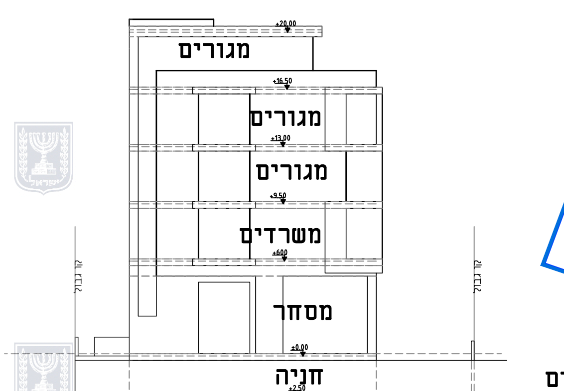
חזית צפונית
