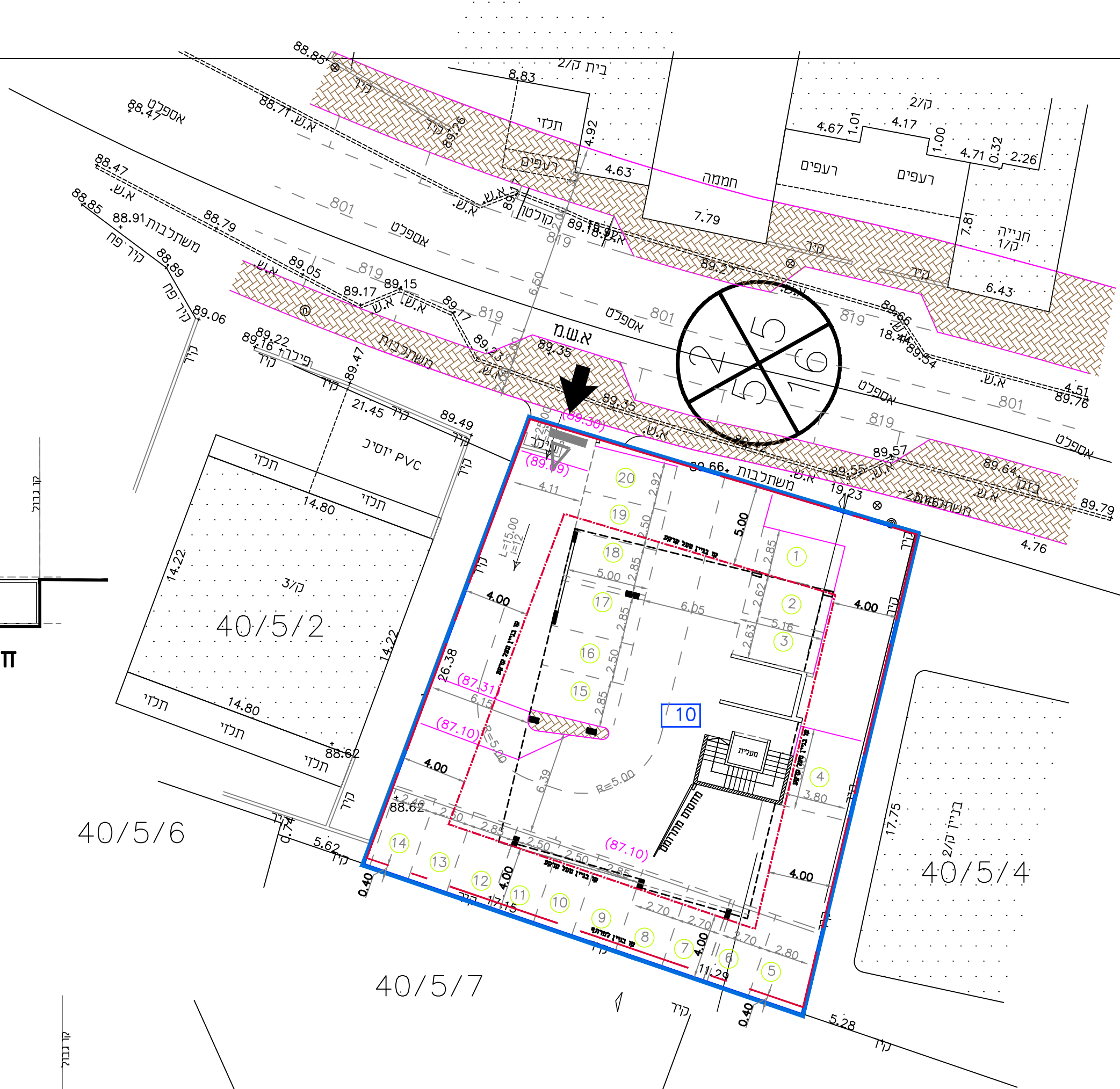
קומת מרתף-חניה
