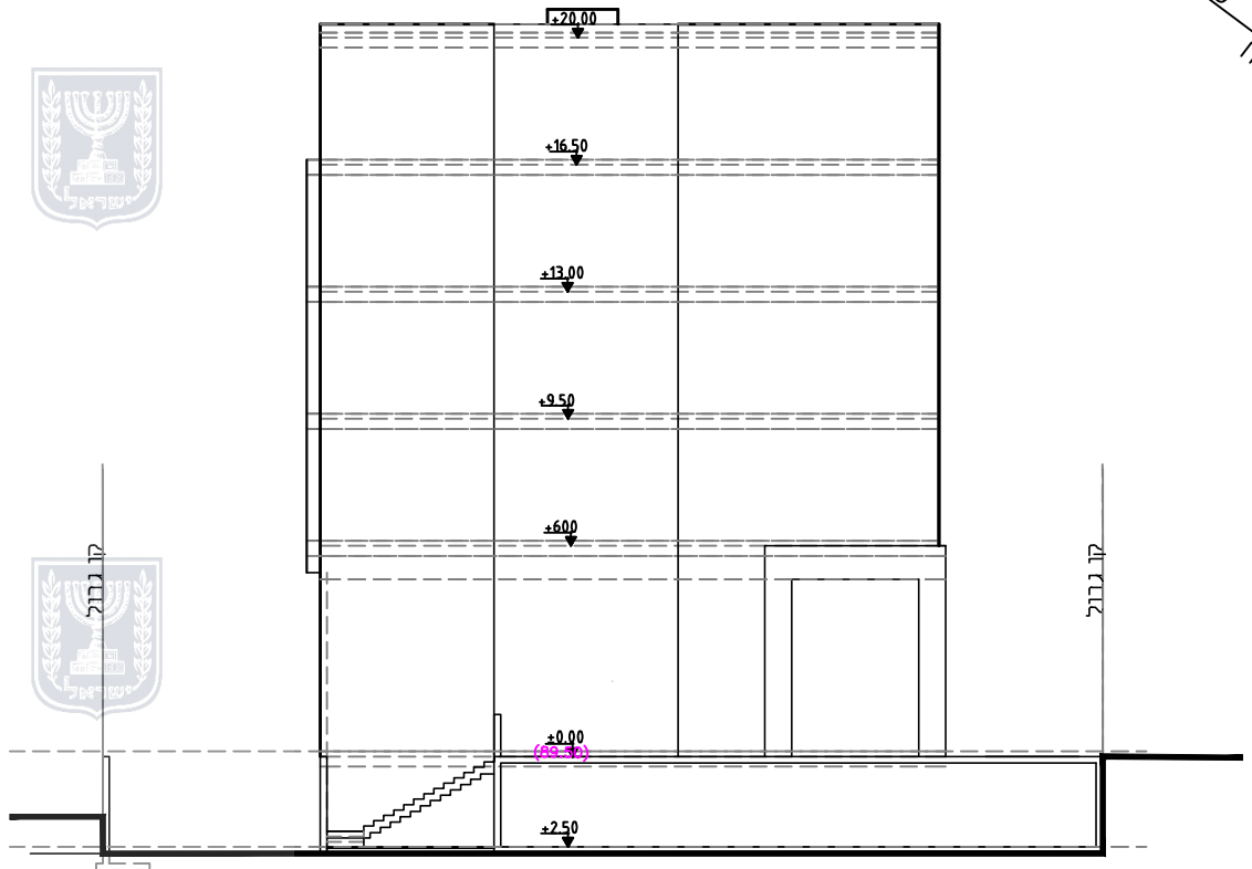
חזית מזרחית
