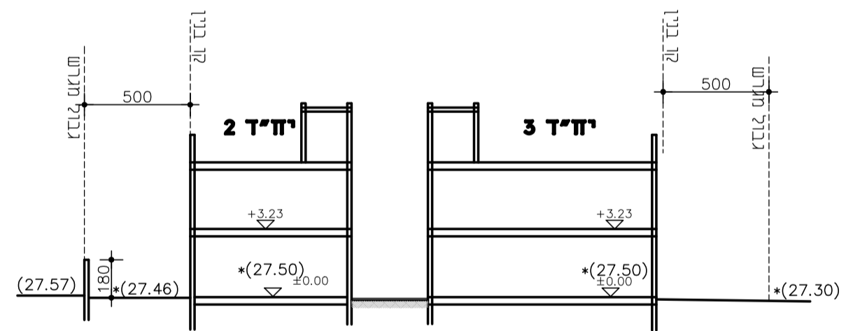
חתך א-א קנים 1:250
