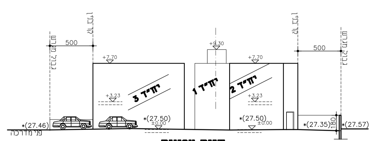
חזית צפונית קנים 1:250
