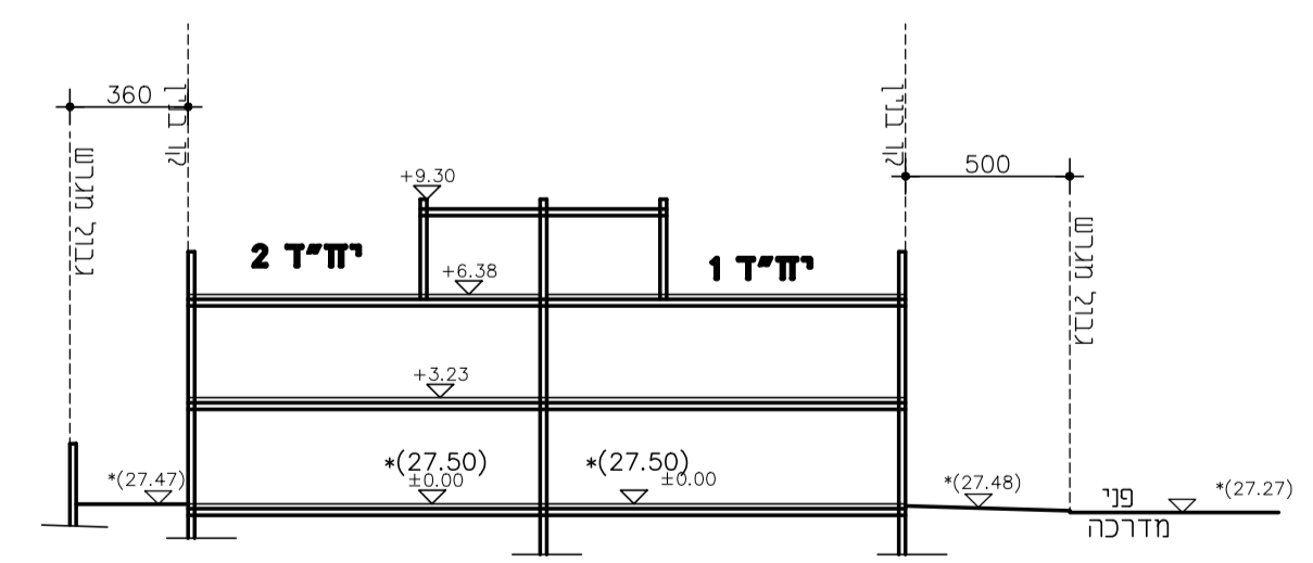
חתך ב-ב קנים 1:250
