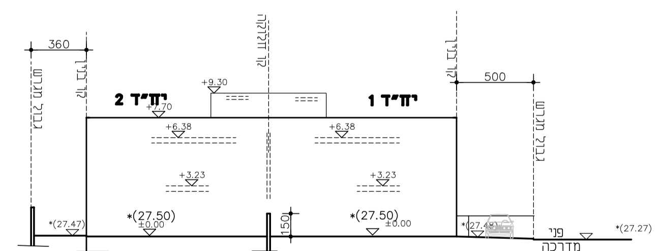
חזית דרום מעבית קנים 1:250
