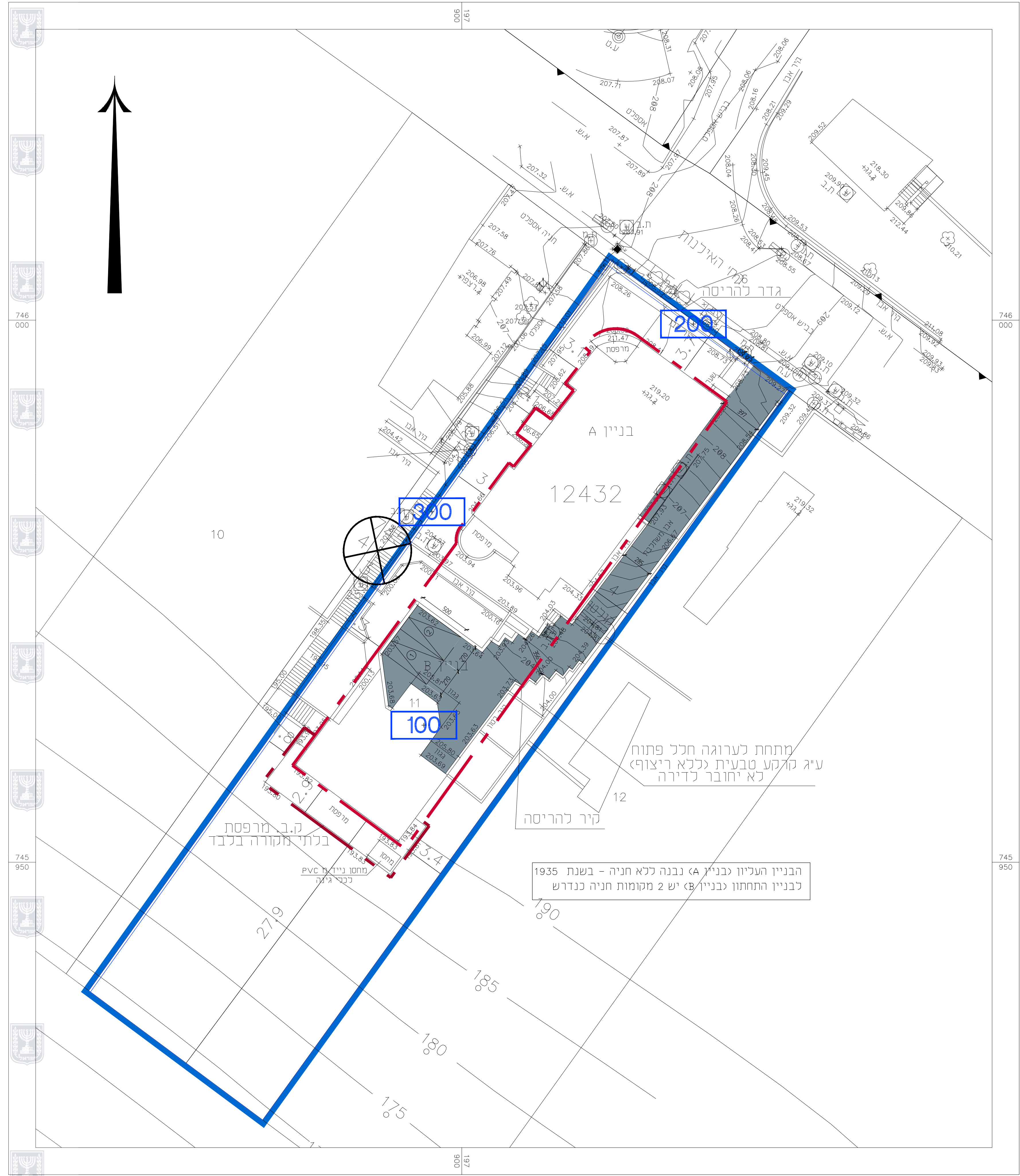
תכנית חנייה 1:200
