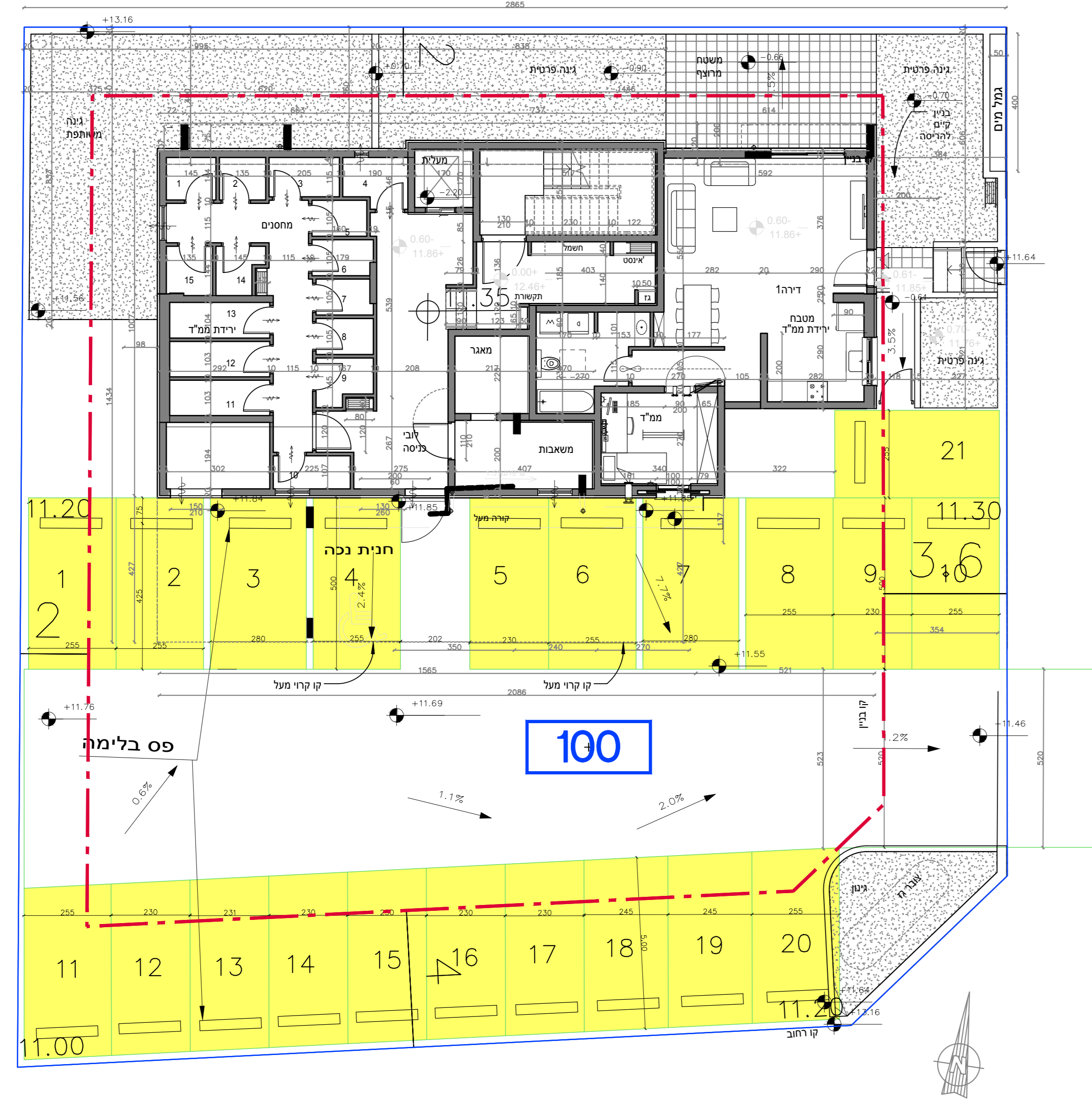
תכנית קומת ארבע קניים 1:100
