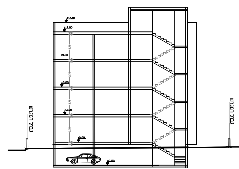
חזית טיפוסי קני"מ 1:250
