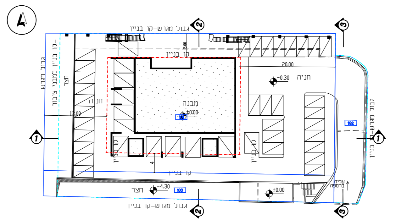
רחבת חניה וכניסה קנ"מ 1:500
