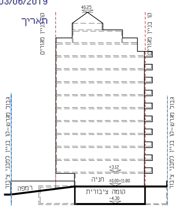
חזית 3-3 קנ"מ 1:500
