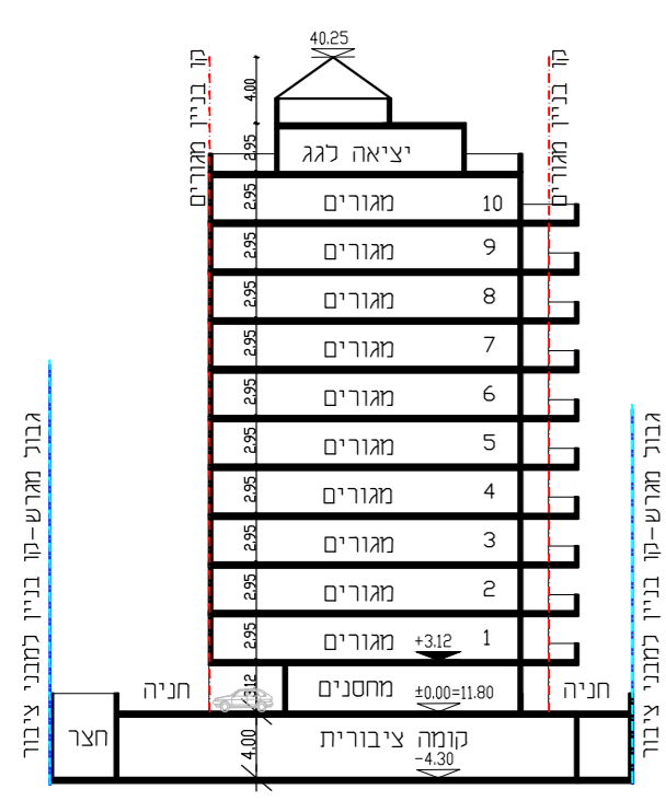
חזית 2-2 קנ"מ 1:500
