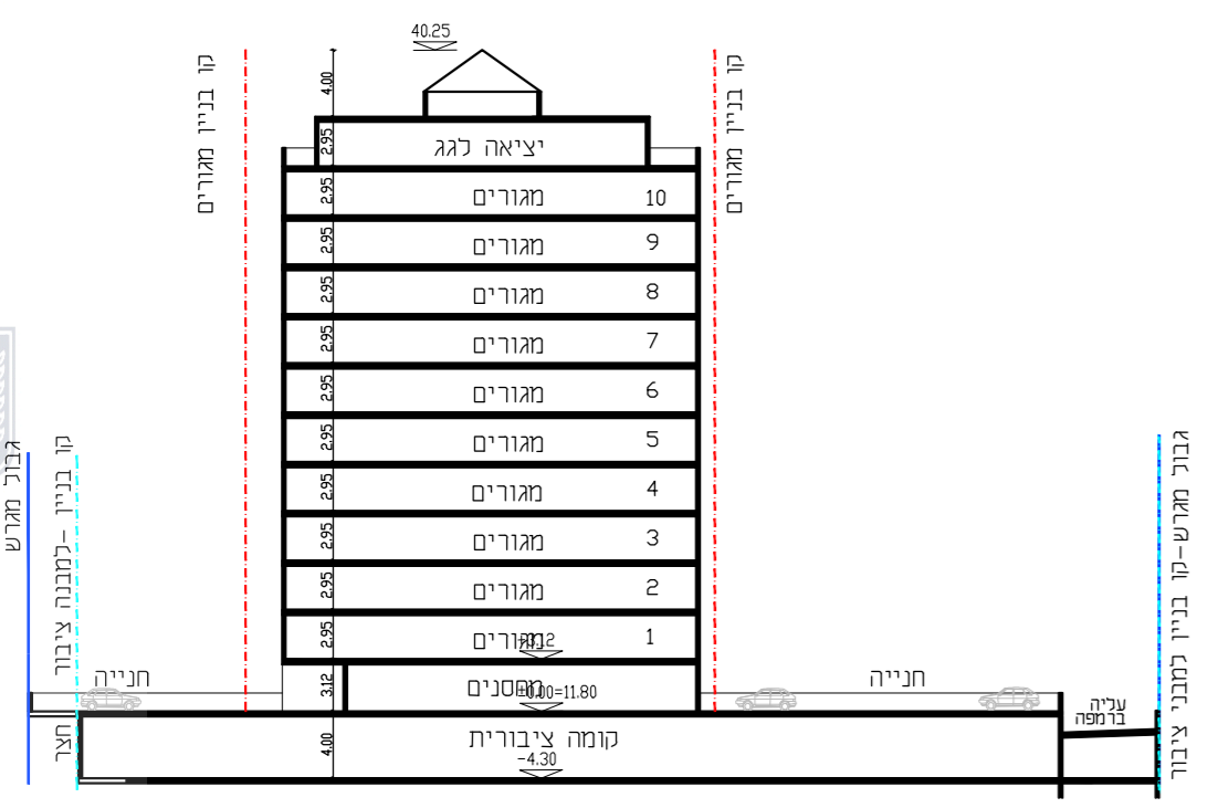
חזית 1-1 קנ"מ 1:500
