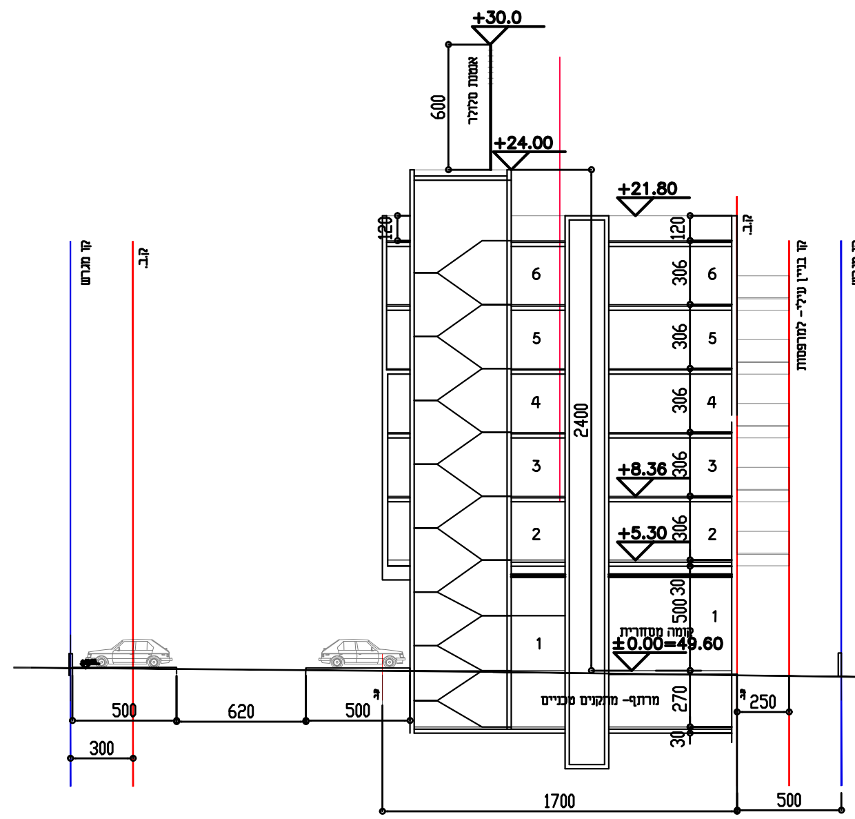
קנ"ב 1:250 חתך א-א
