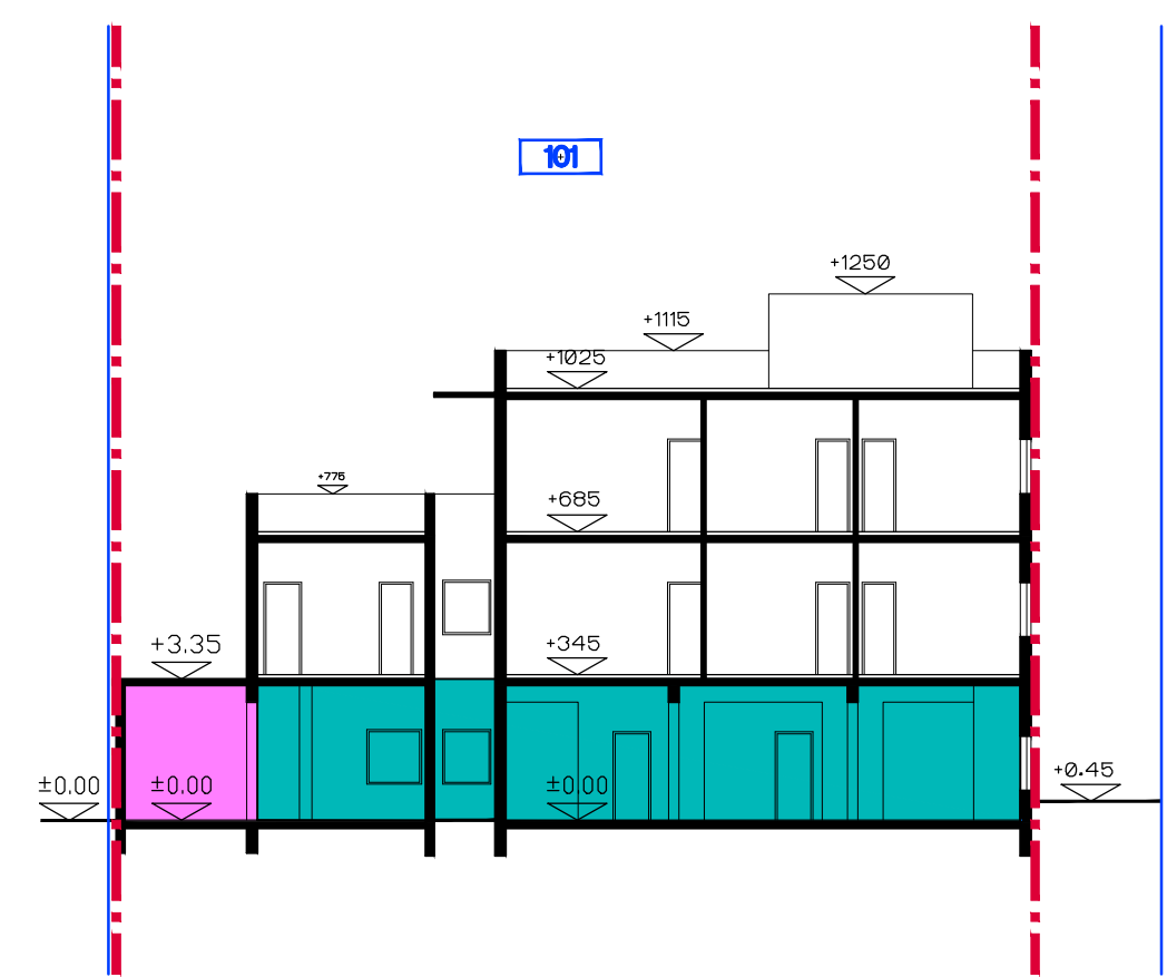
חיתך ב-ב - קנ"מ 1:200
