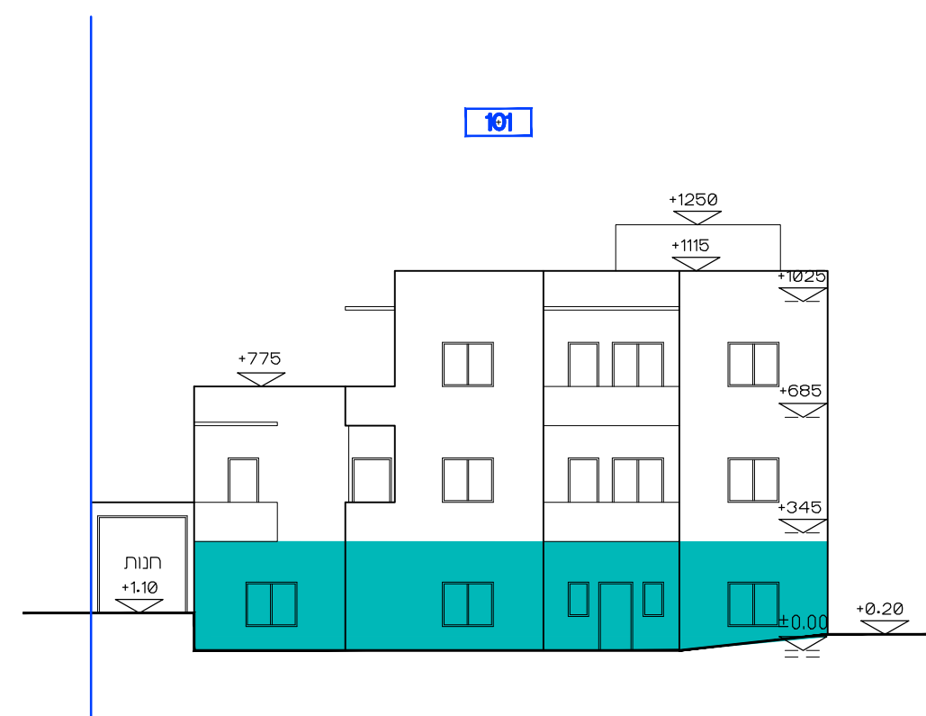
חזית דרומית - קנ"מ 1:200
