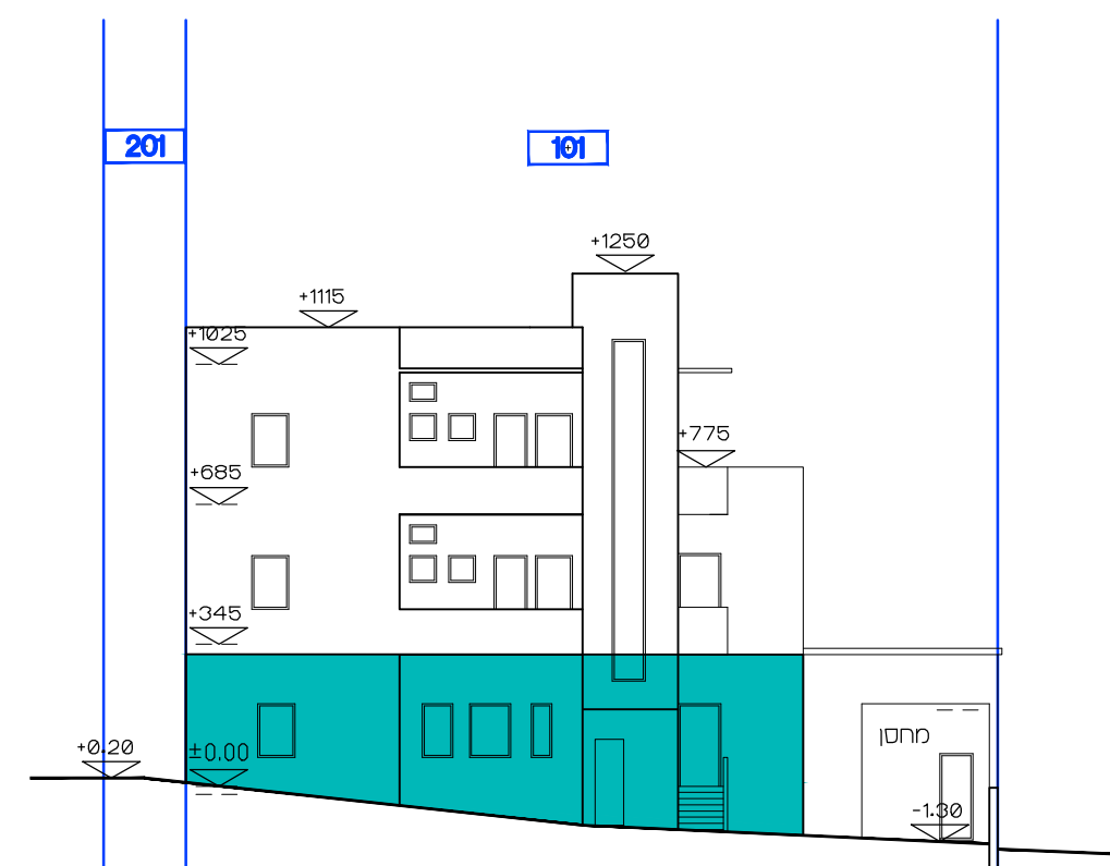
חזית מזרחית - קנ"מ 1:200
