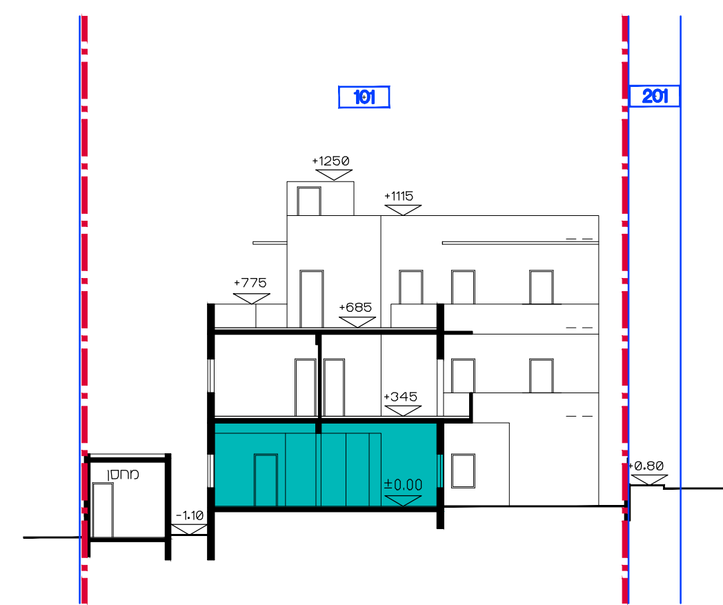
חיתך א-א - קנ"מ 1:200
