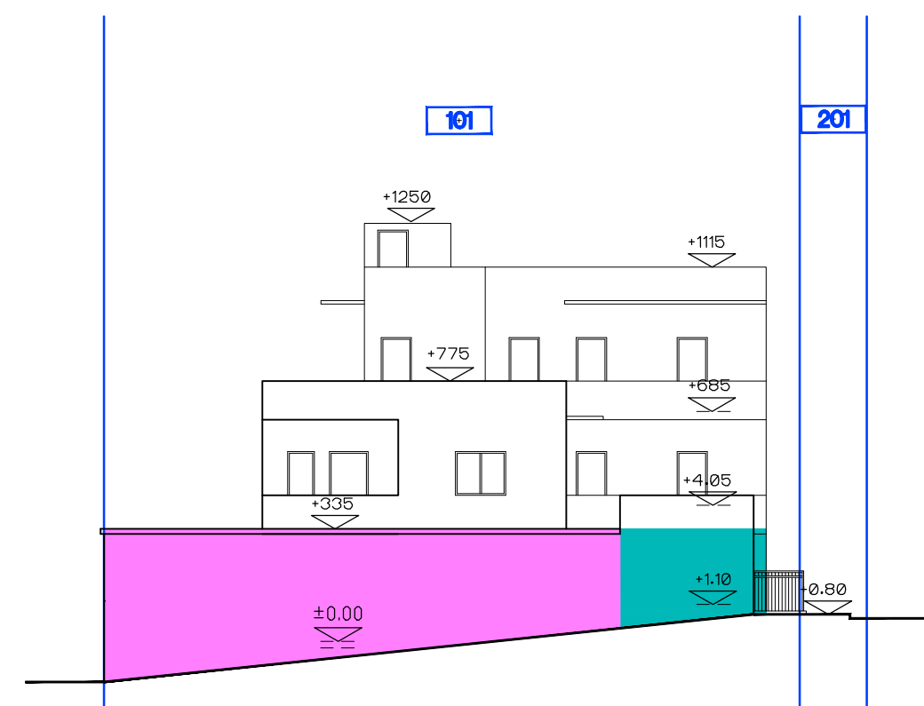
חזית מערבית - קנ"מ 1:200
