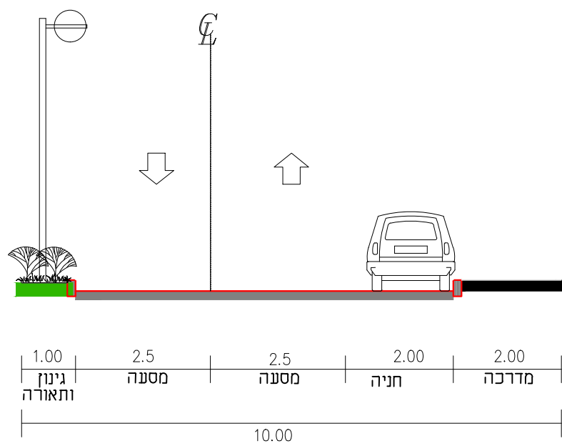
חתך 2-2 חתך טיפוסי 10 מ' קנ"מ 1:100
