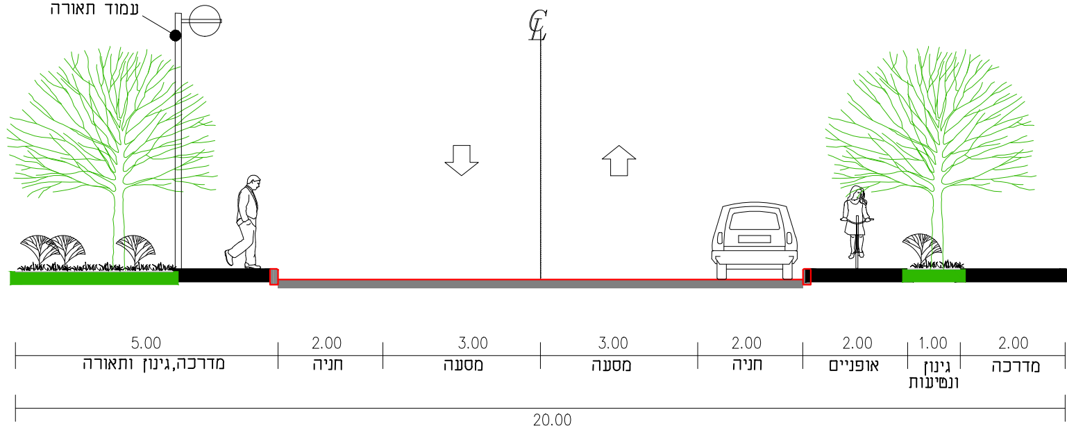
חתך 9-9 חתך טיפוסי 20 מ' קנ"מ 1:100
