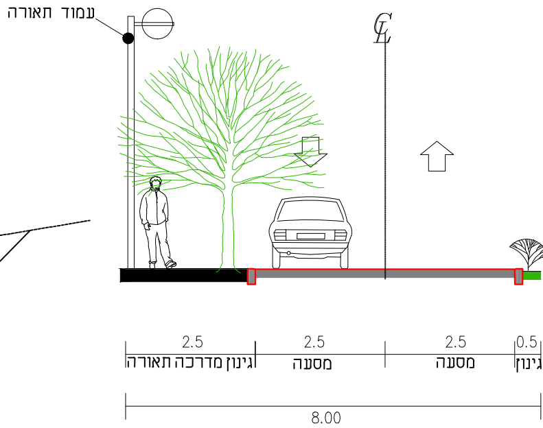
חתך 1-1 חתך טיפוסי 8 מ' קנ"מ 1:100
