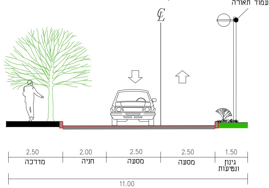
חתך 4-4 חתך טיפוסי 11 מ' קנ"מ 1:100
