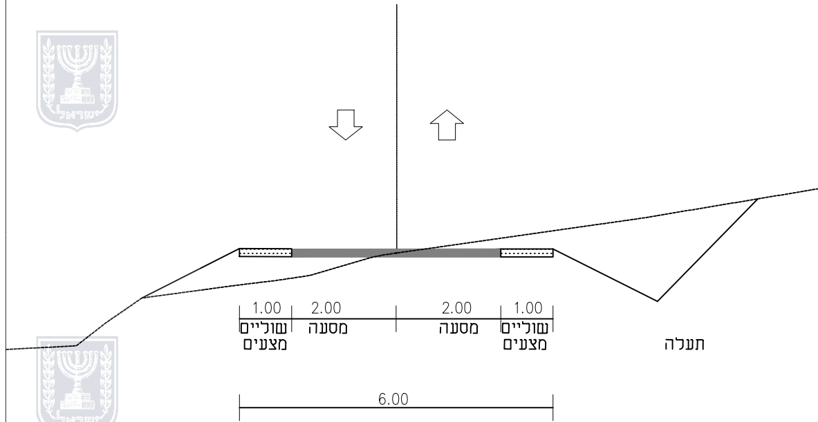
חתך טיפוסי 6 מ' דרכי גישה לת.שאיבה קנ"מ 1:100
