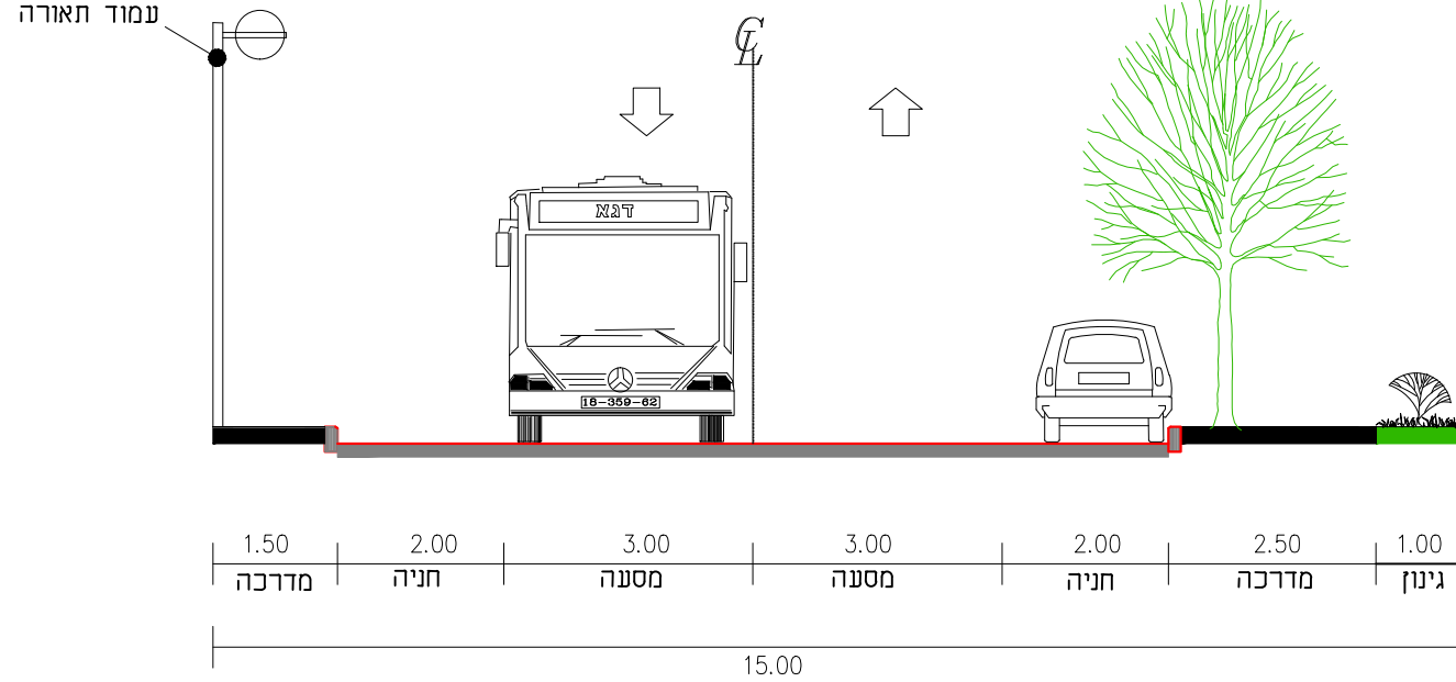
חתך 8-8 חתך טיפוסי 15 מ' קנ"מ 1:100
