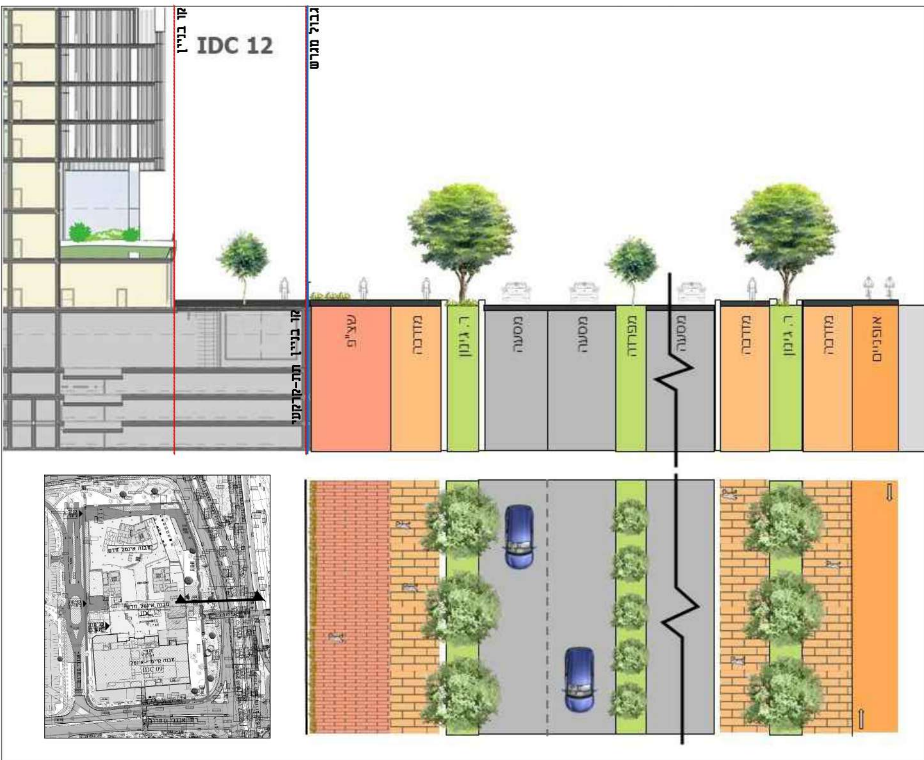
חתך רחוב- כביש 4 ממזרח למבנה מתוכנן
