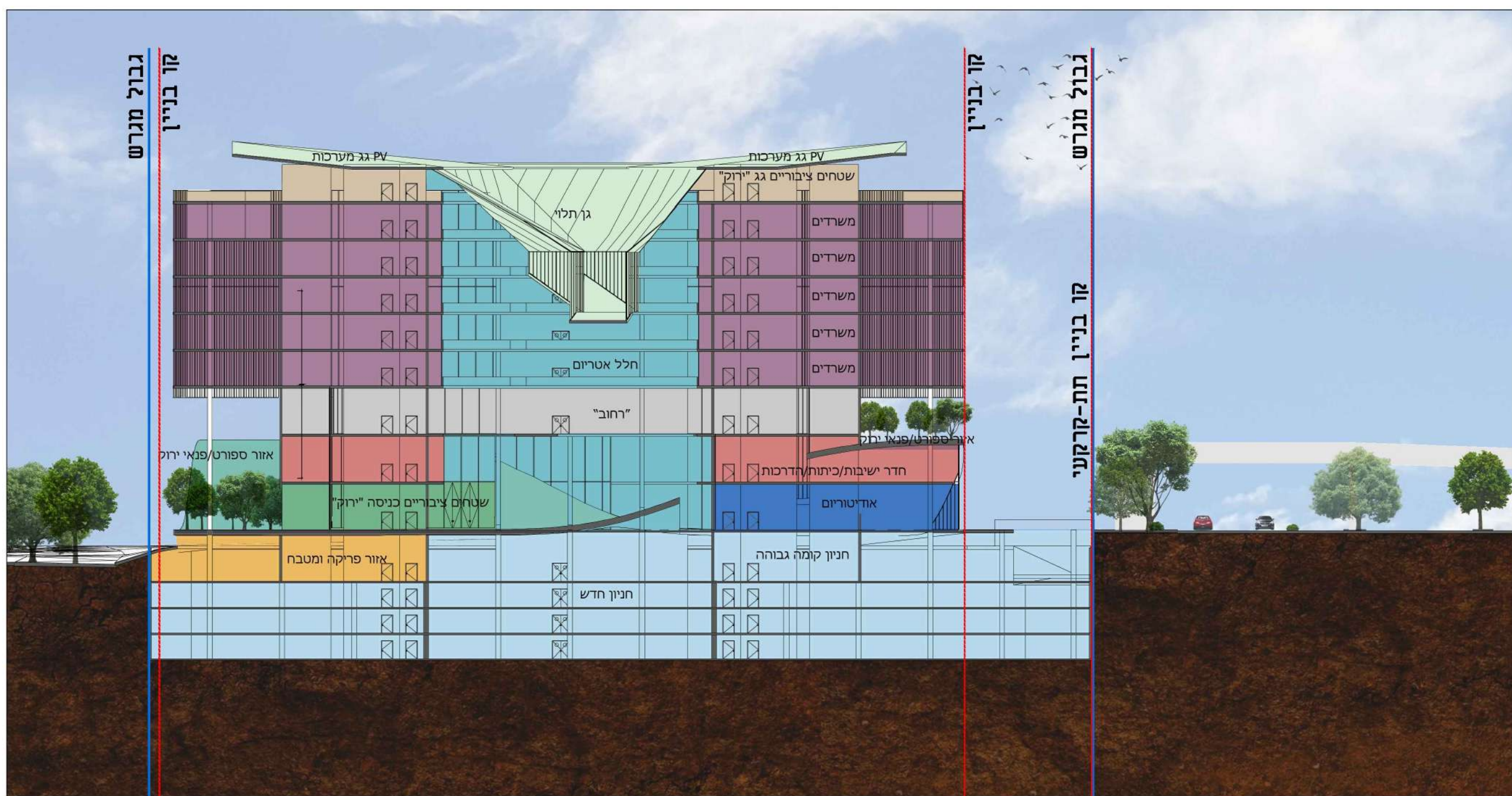
חתך א-א קנה מידה 1:500
