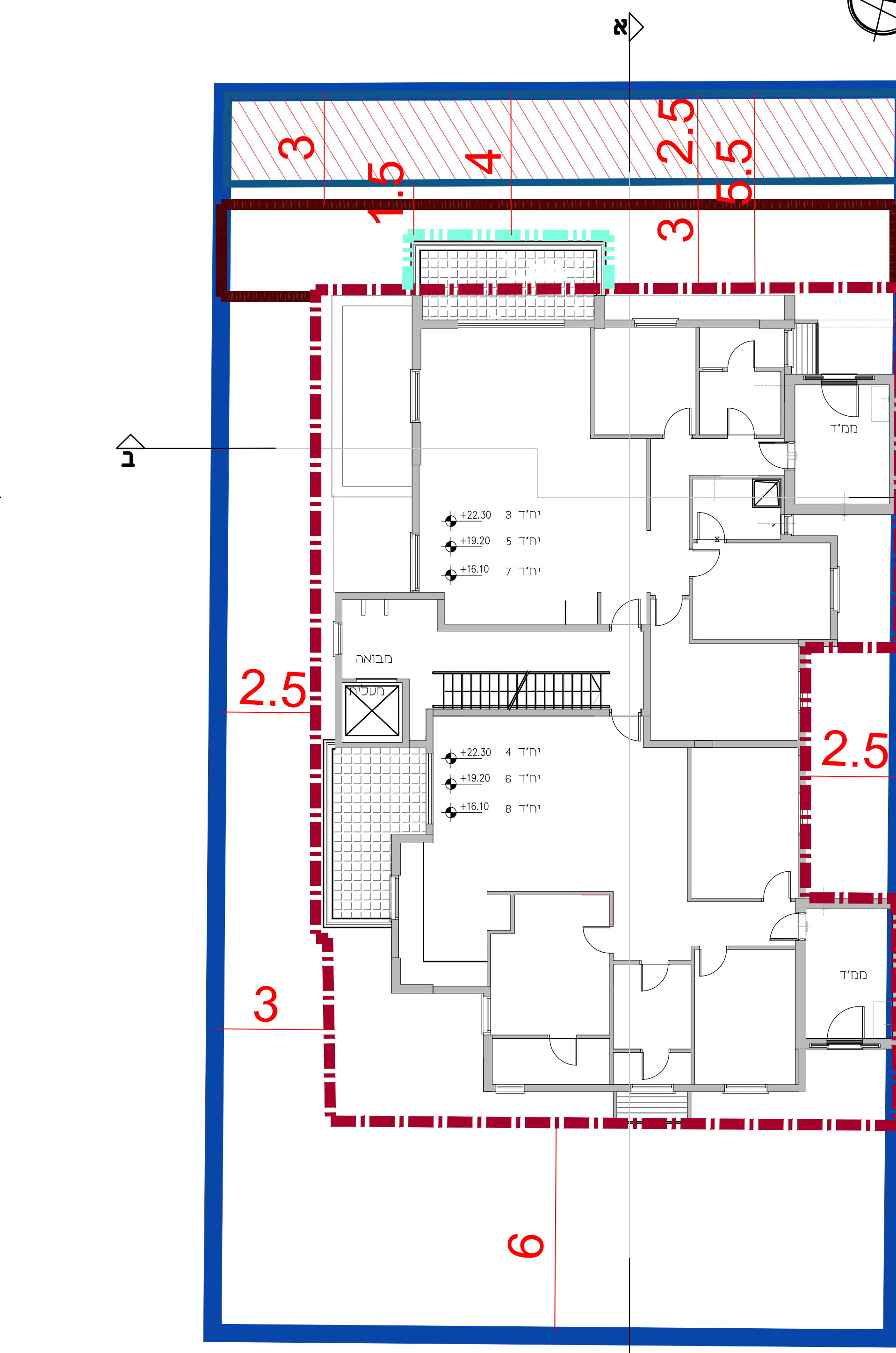
תכנית קומות 5+6+7 1:100 קני"מ
