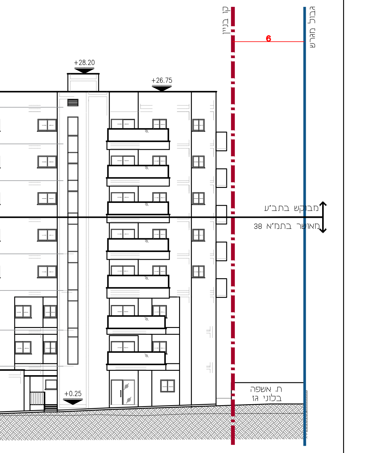
זחיתות וזחתיים 1:200 קני"מ
