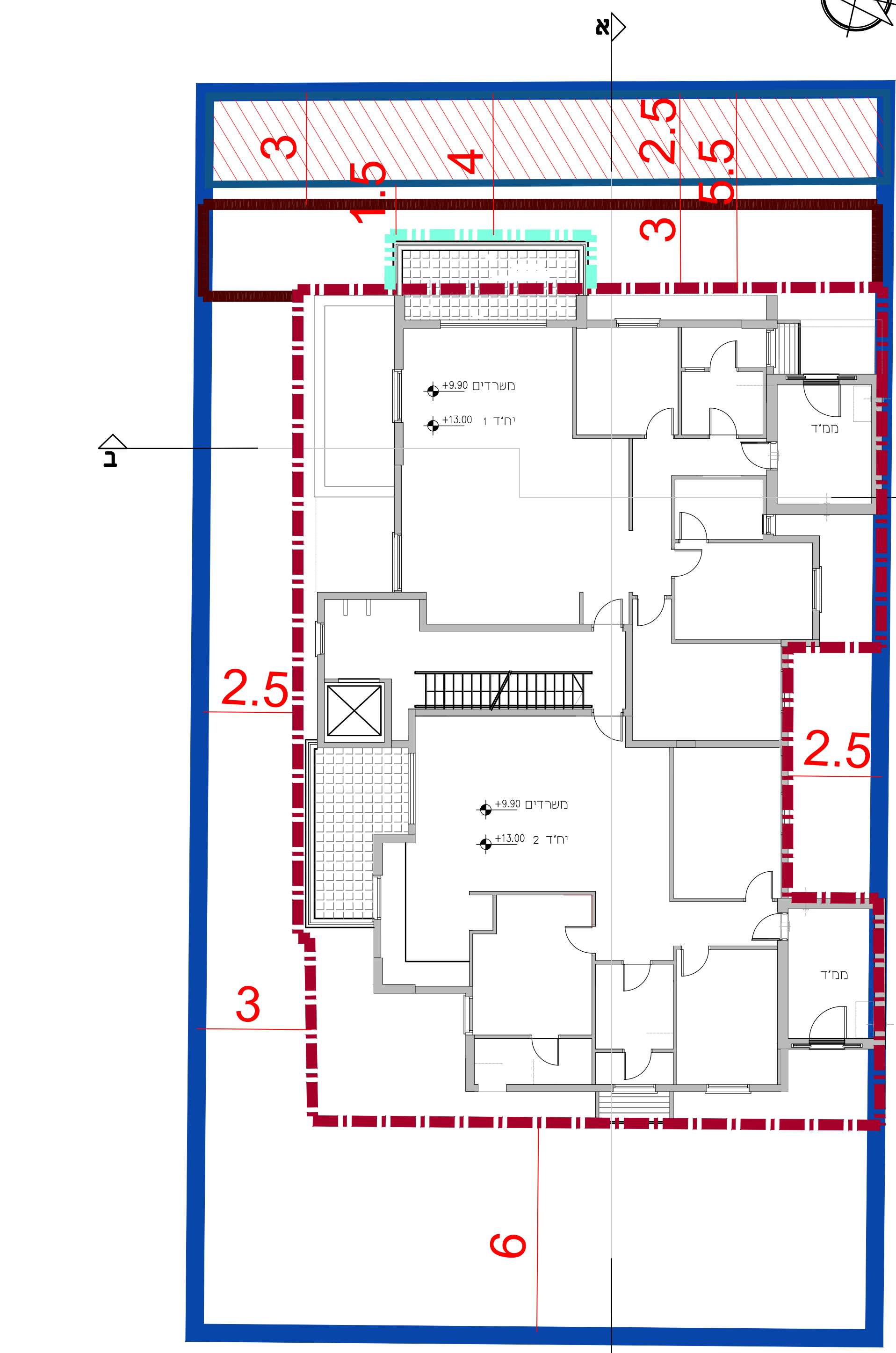
תכנית קומות 3+4 1:100 קני"מ
