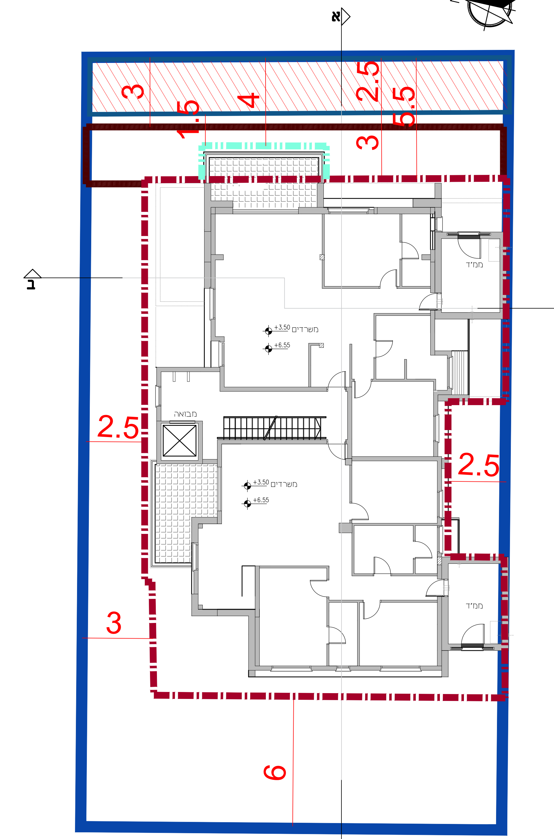
תכנית קומות 2+1 1:100 קני"מ
