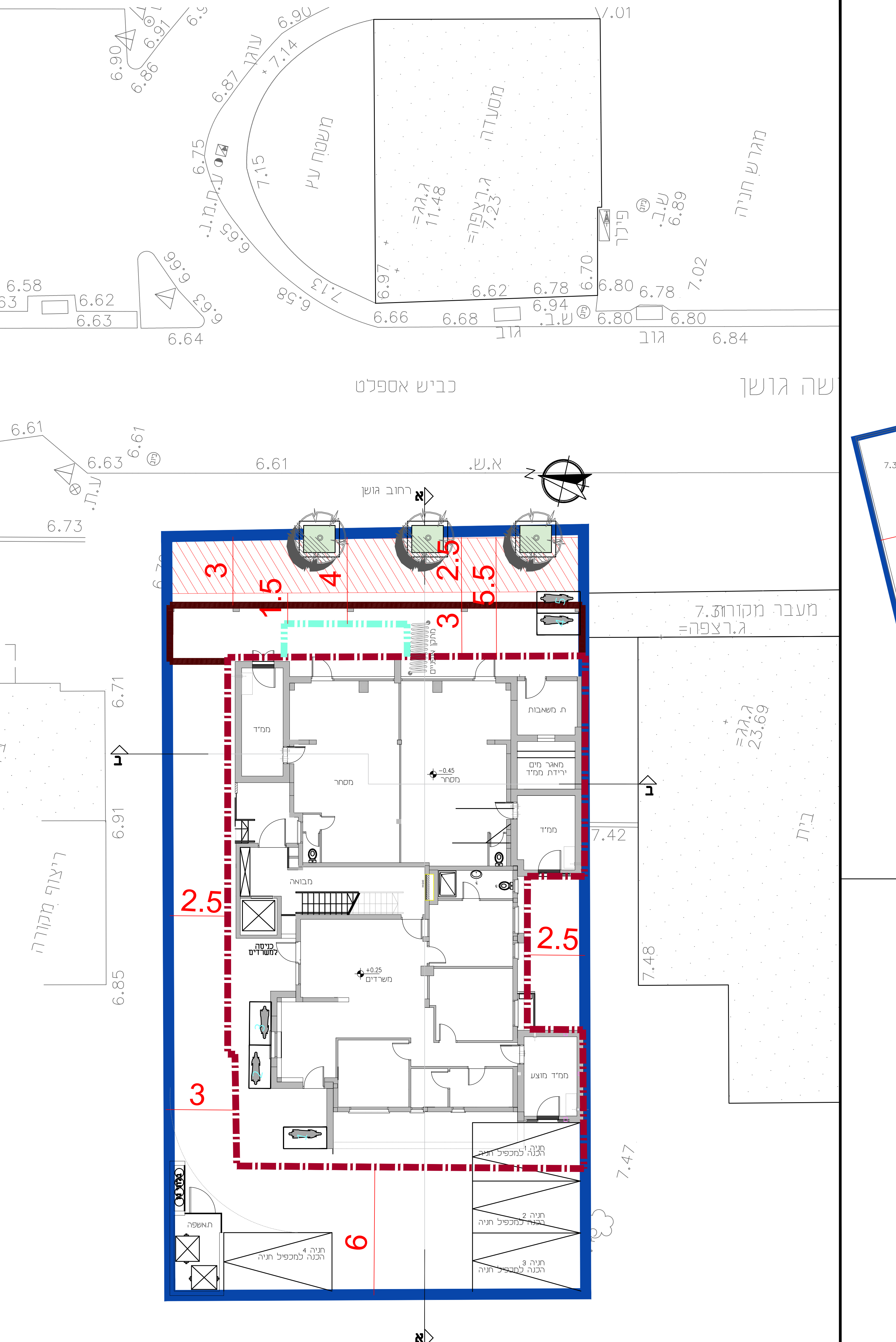
תכנית קומות קרקע 1:100 קני"מ
