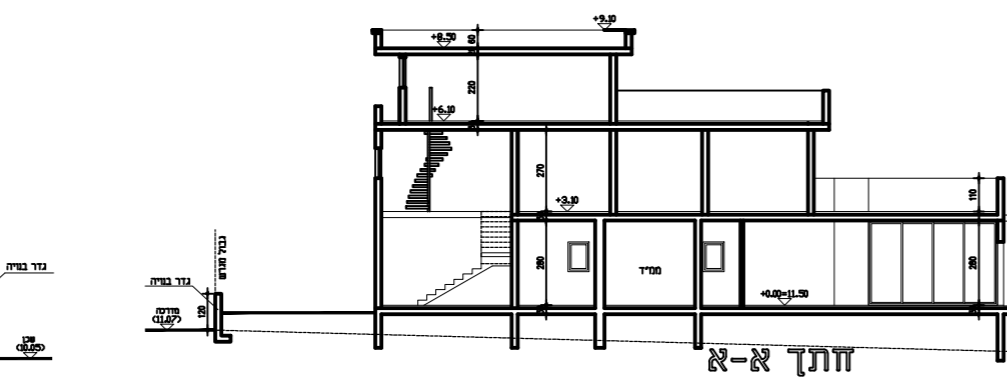
חזית א-א ק.נ.מ. 1:100
