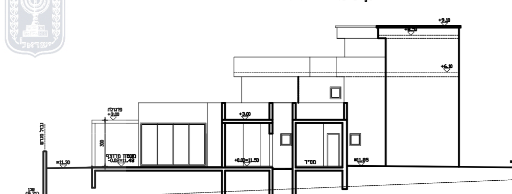
חזית מזרחית ק.נ.מ. 1:100
