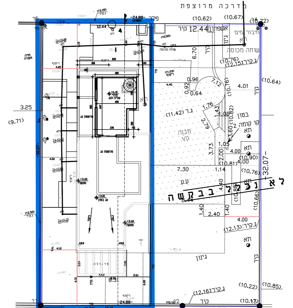
תכנית קומת עליה לגג ק.נ.מ. 1:100
