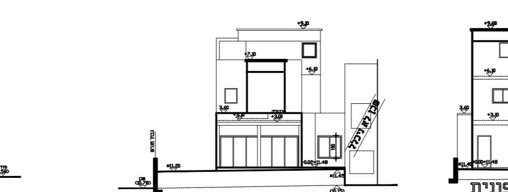
חזית דרומית ק.נ.מ. 1:100
