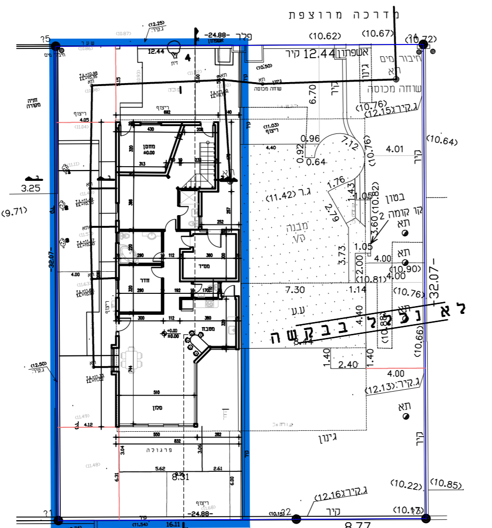
תכנית קומת קרקע ופיתוח המגרש ק.נ.מ. 1:100
