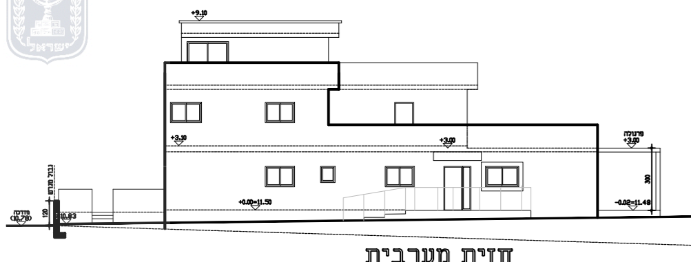
חזית מערבית ק.נ.מ. 1:100
