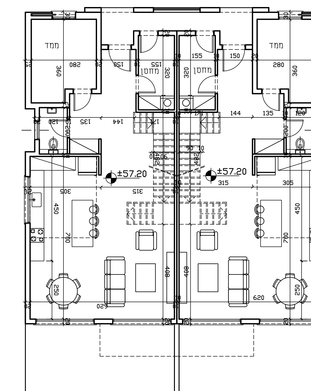
תכנית קומת כניסה ק.מ. 1:100
