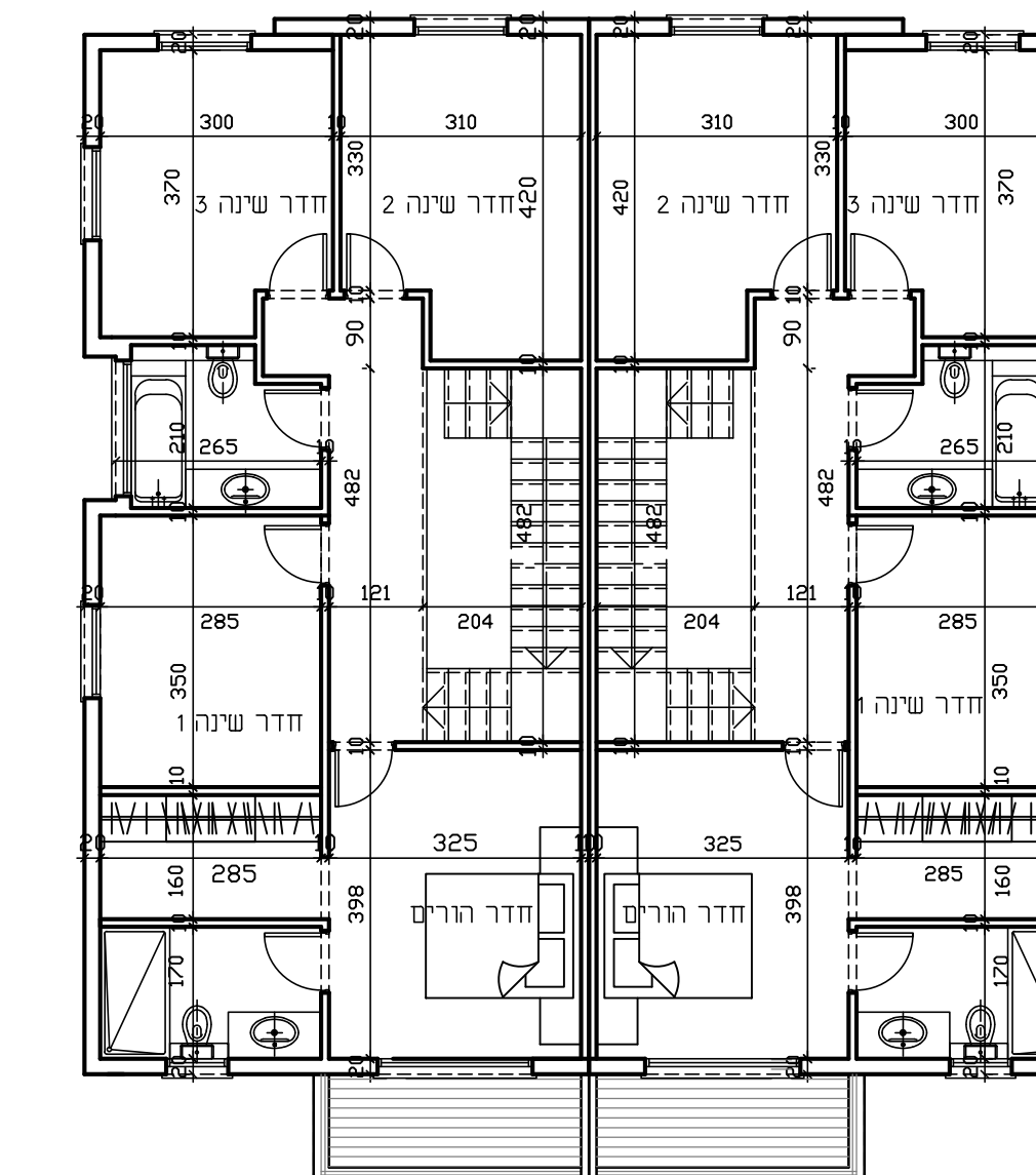
תכנית קומה אי ק.מ. 1:100
