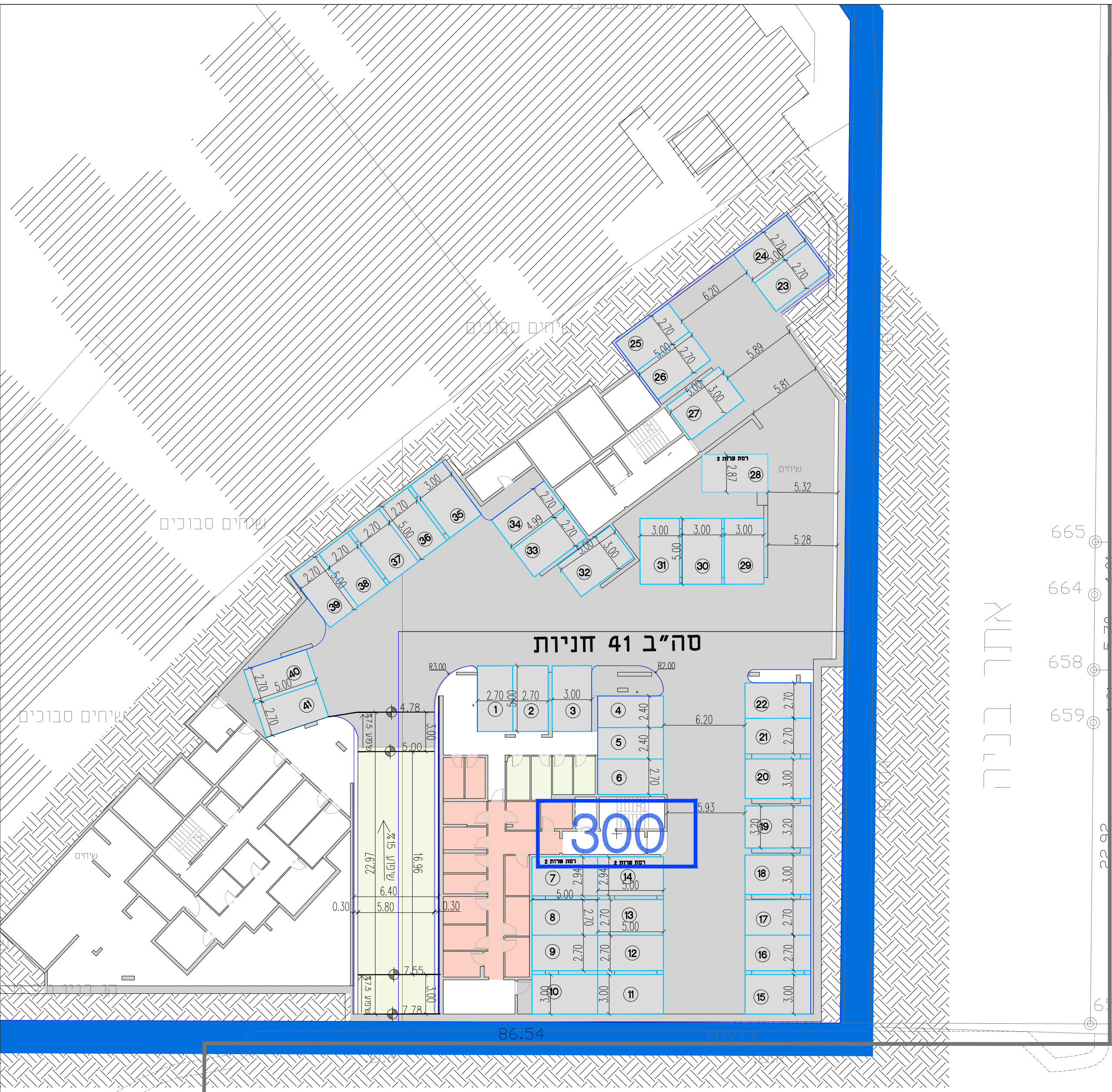
תכנית קומת מרתף קנ"מ 1:250
