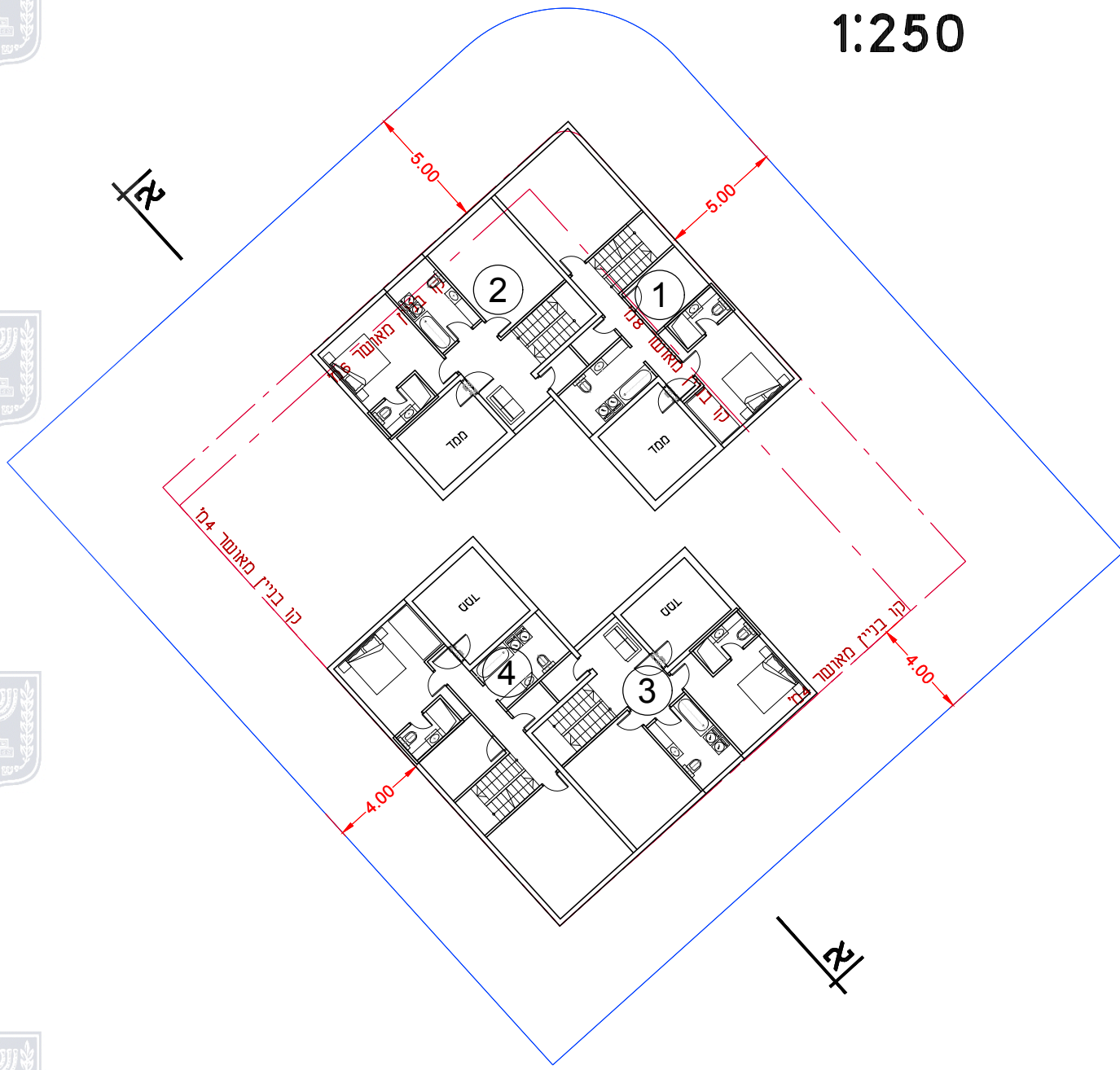
קומה 1: מפלס עליון קוטגיים
