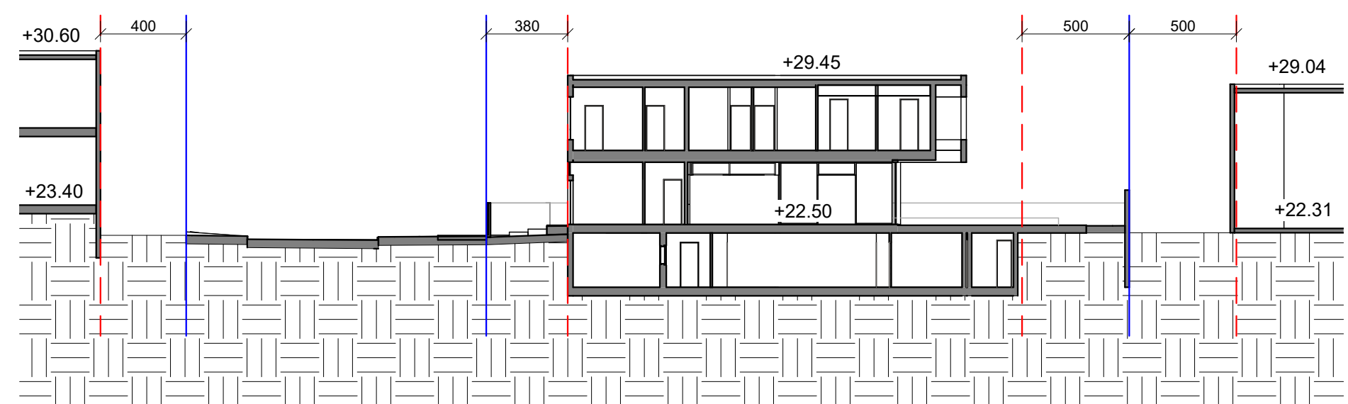
חתך א-א
