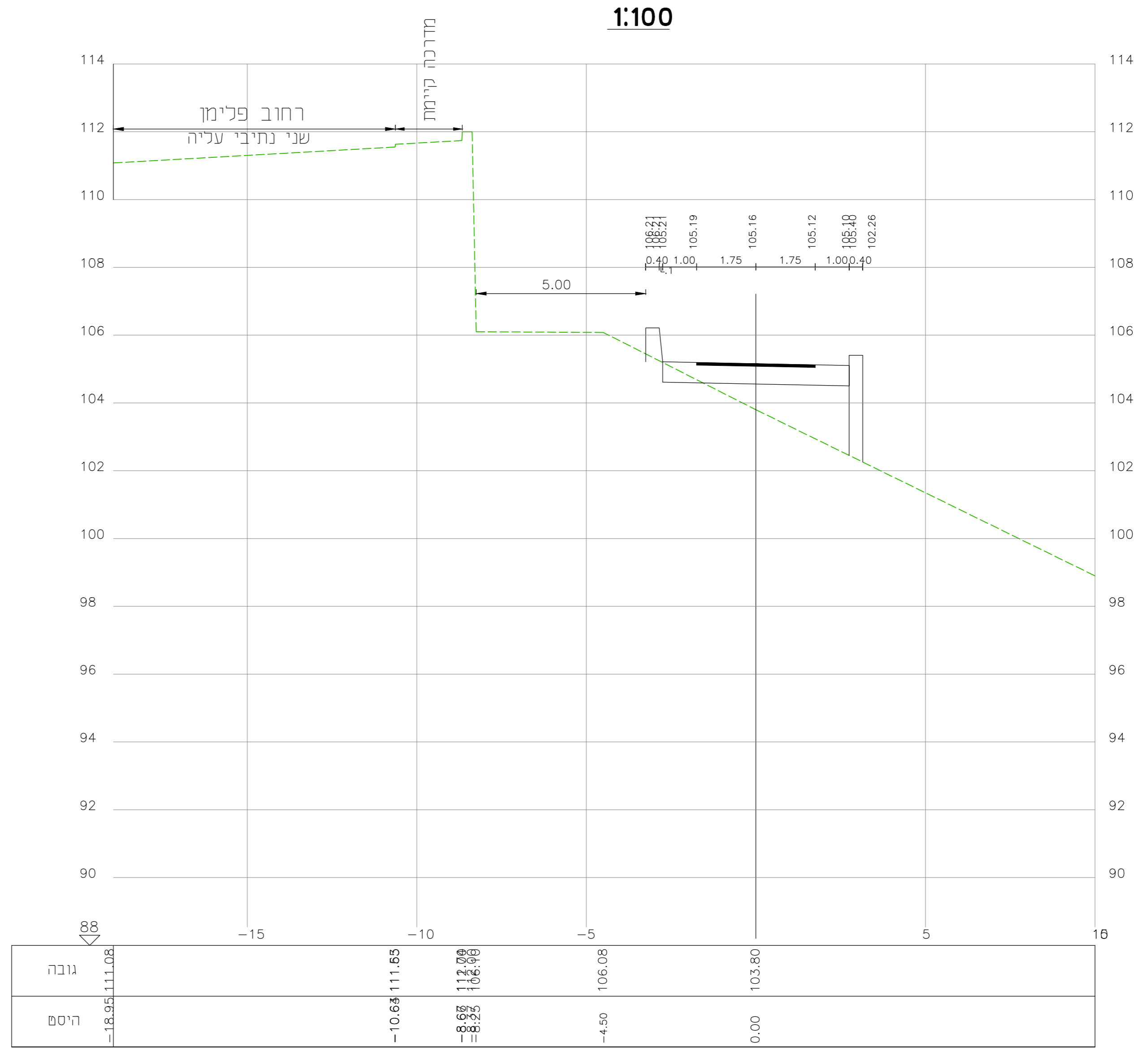
חיפה_מאגר מרחק רץ = 70 חתך A
