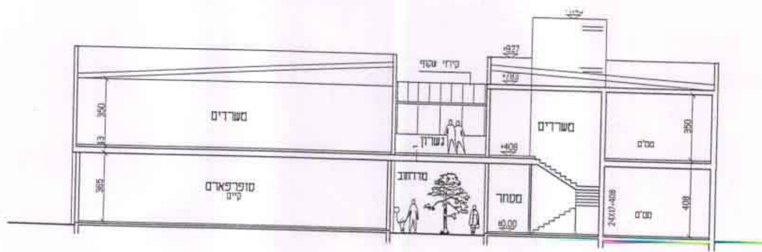
חתך א-א 1:200 SEC1
