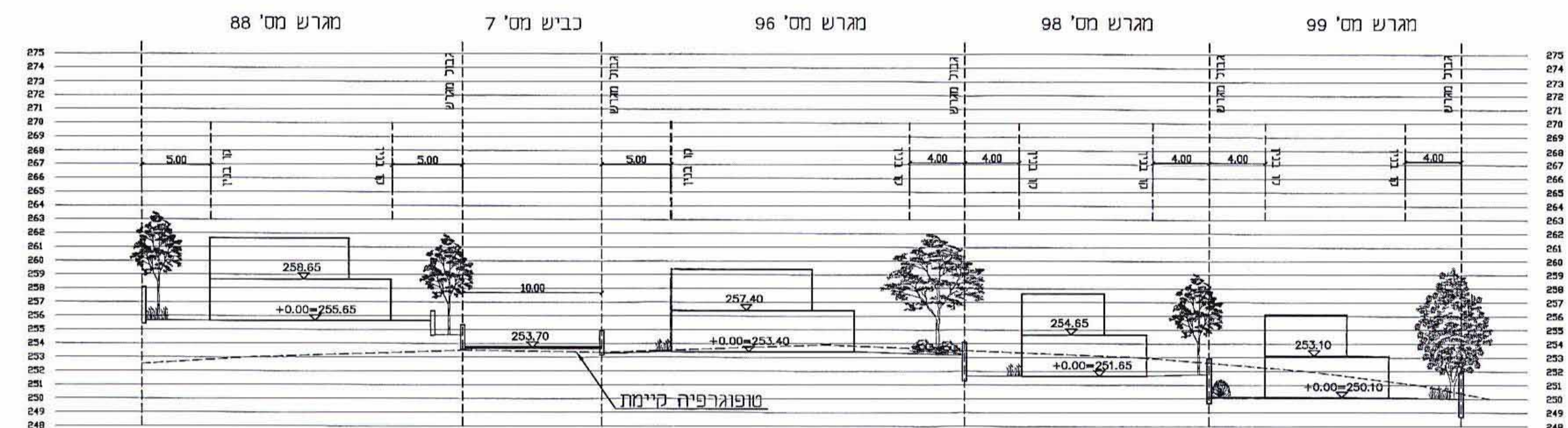
4-4 חתך
