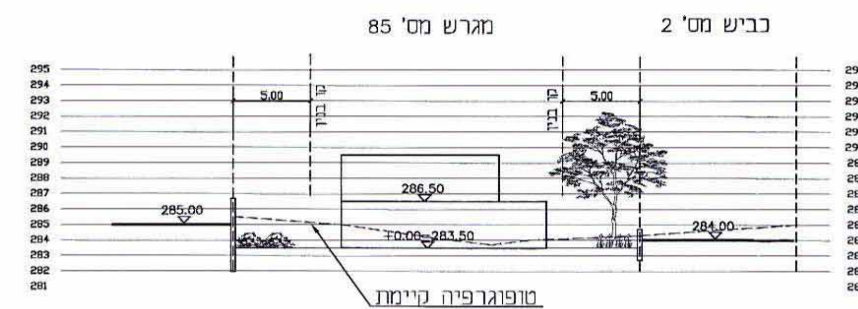
6-6 חתך
