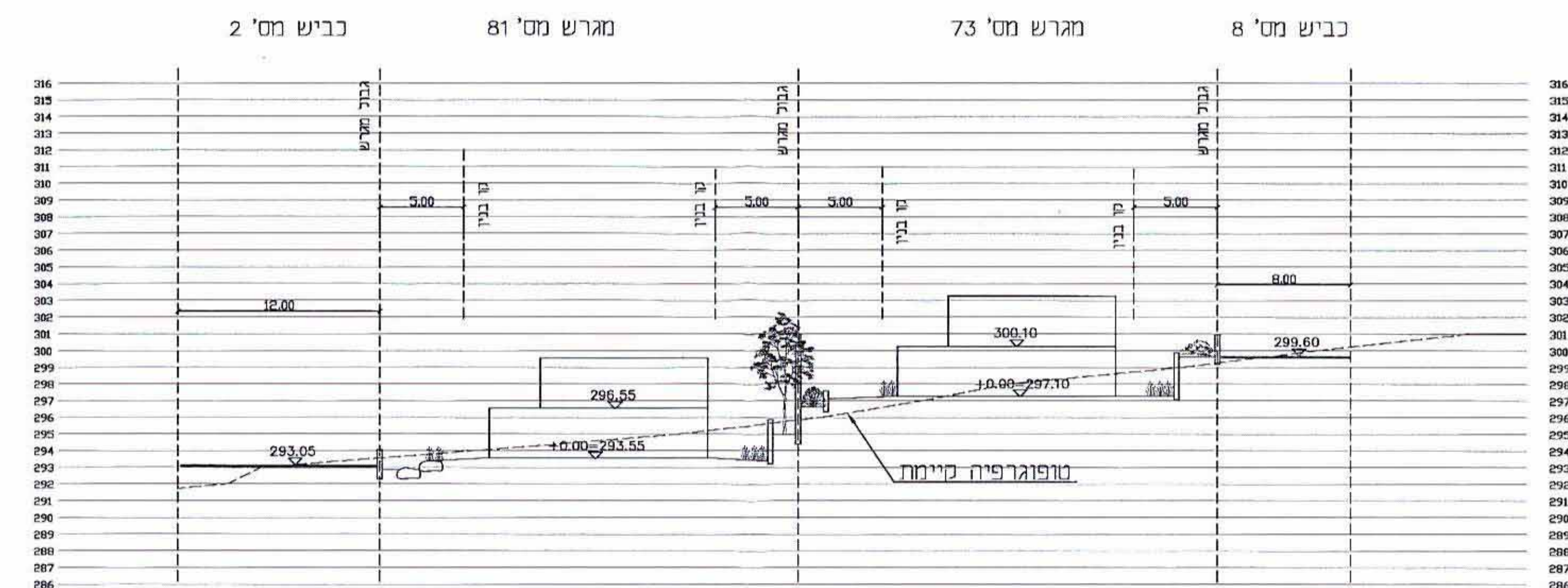
3-3 חתך
