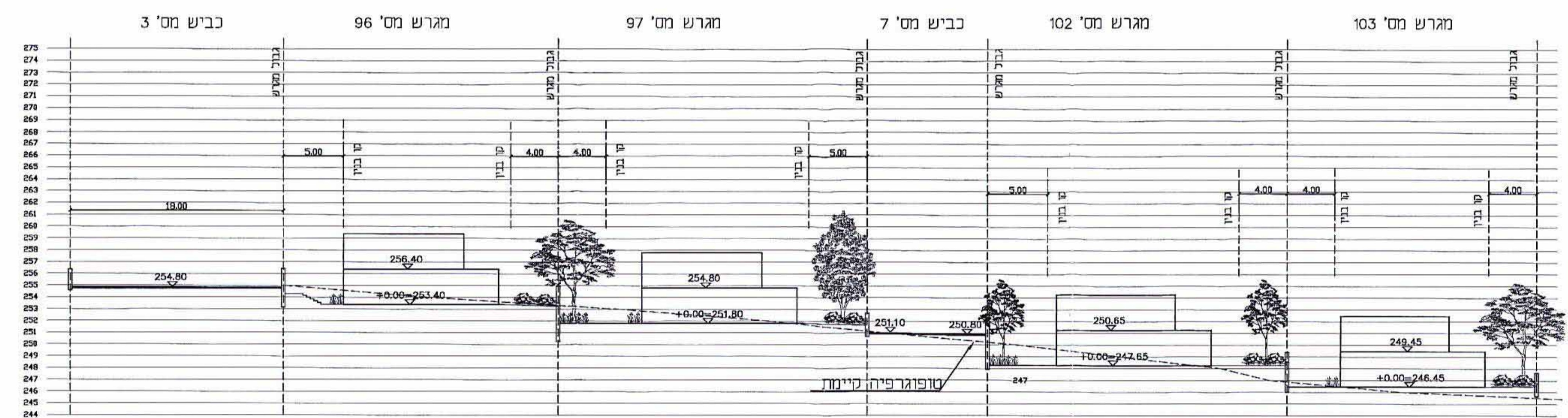
5-5 חתך
