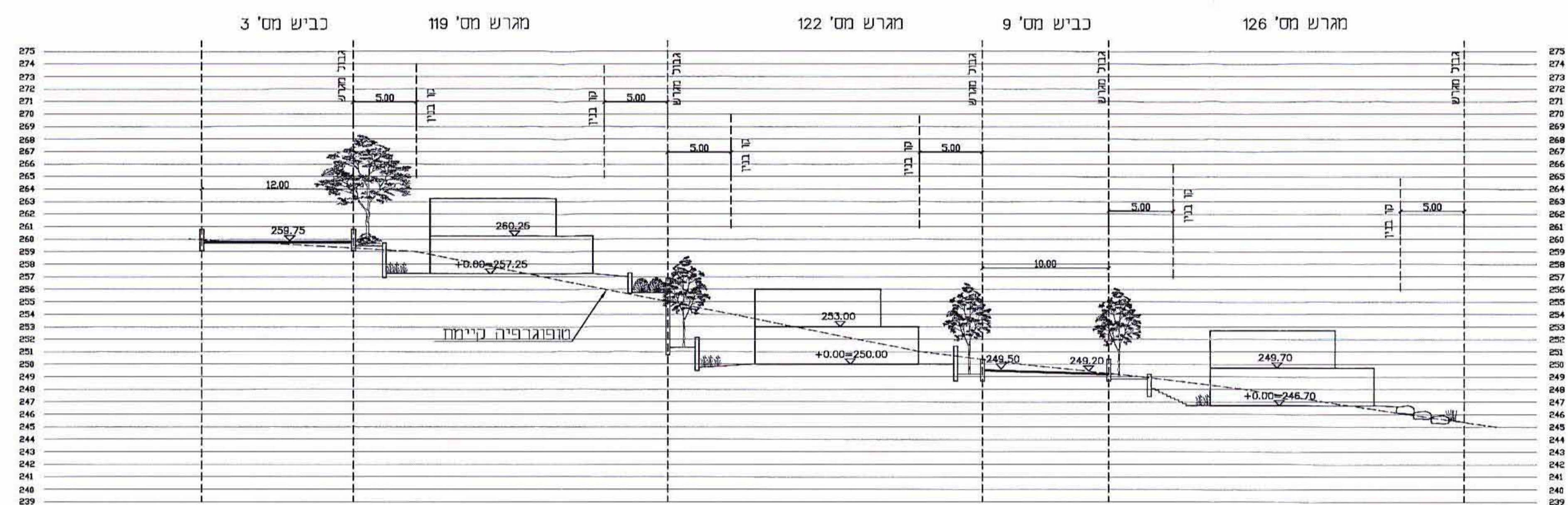
2-2 חתך
