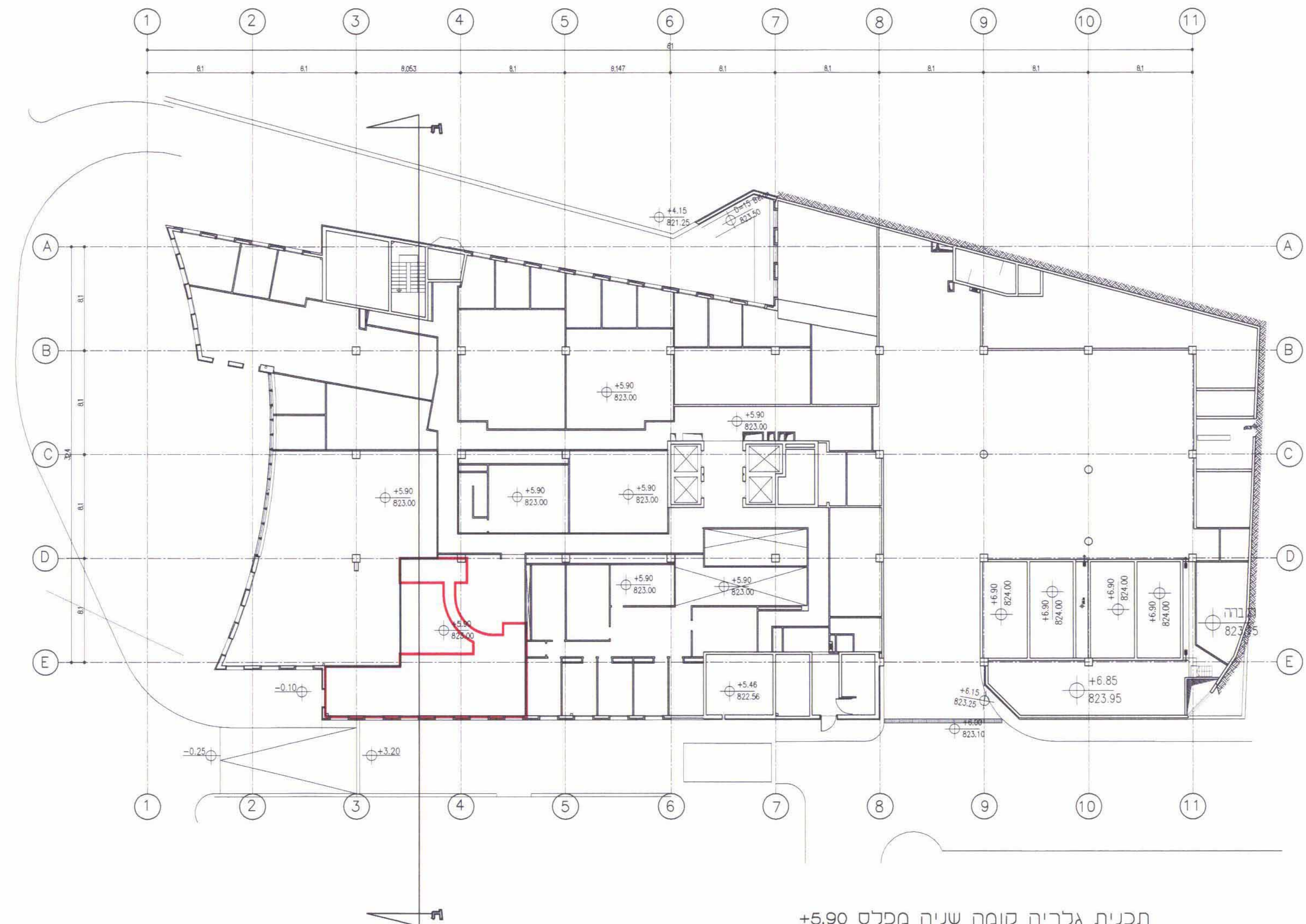
תכנית גלריה קומה שניה במפלס +5.90 ק"מ: 1:200
