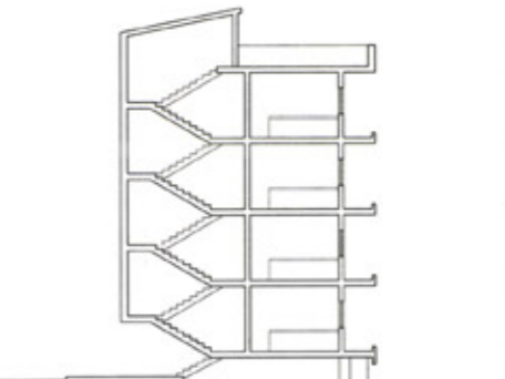
4 חזית א-א - מצב קיים
