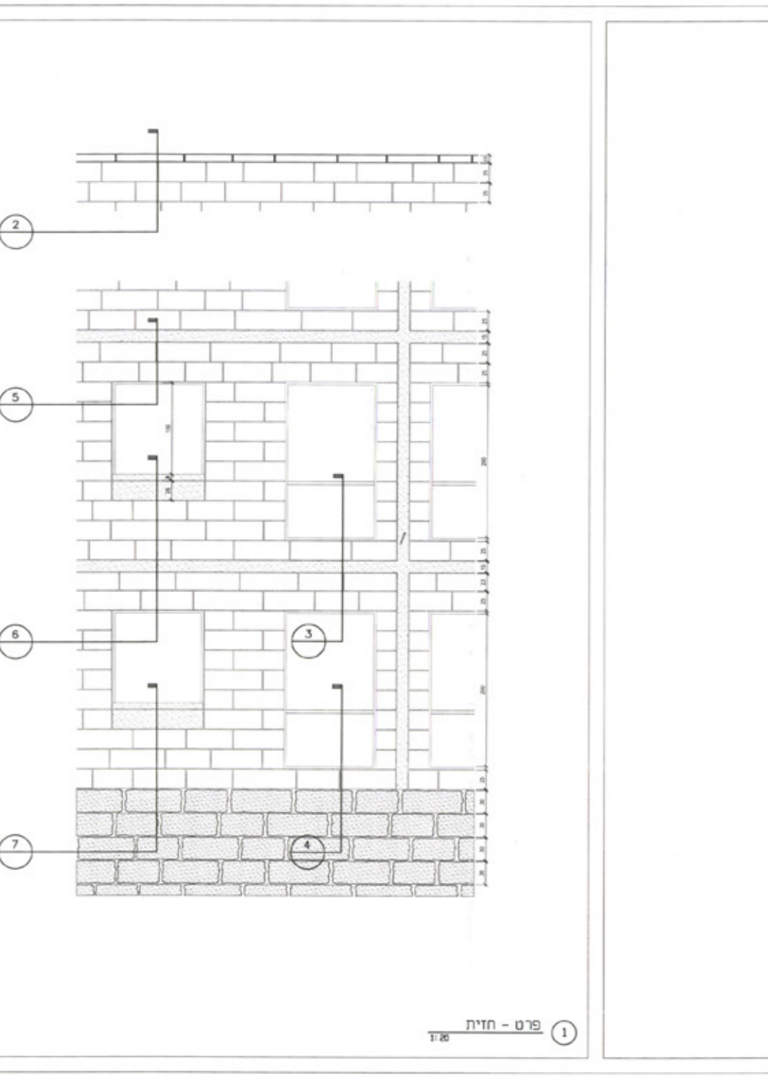
1 פרט - חזית
