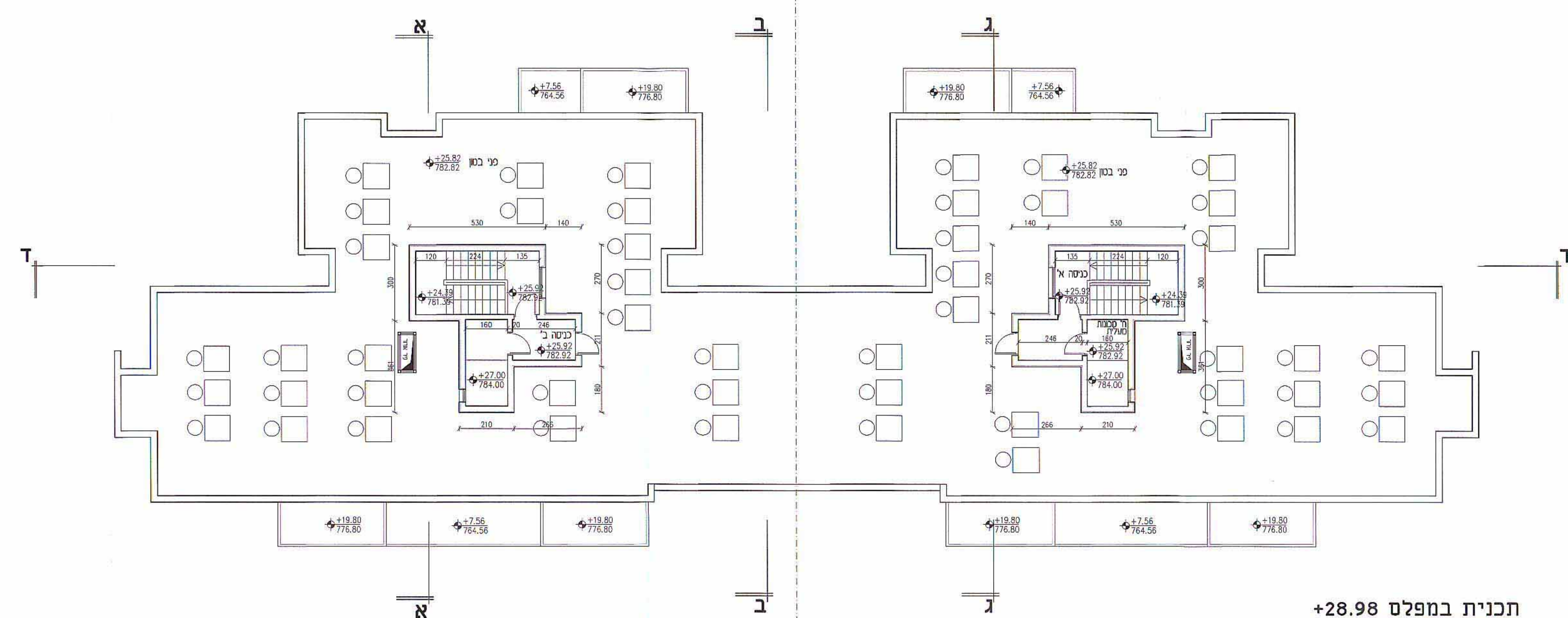
תכנית במפלס +28.98
