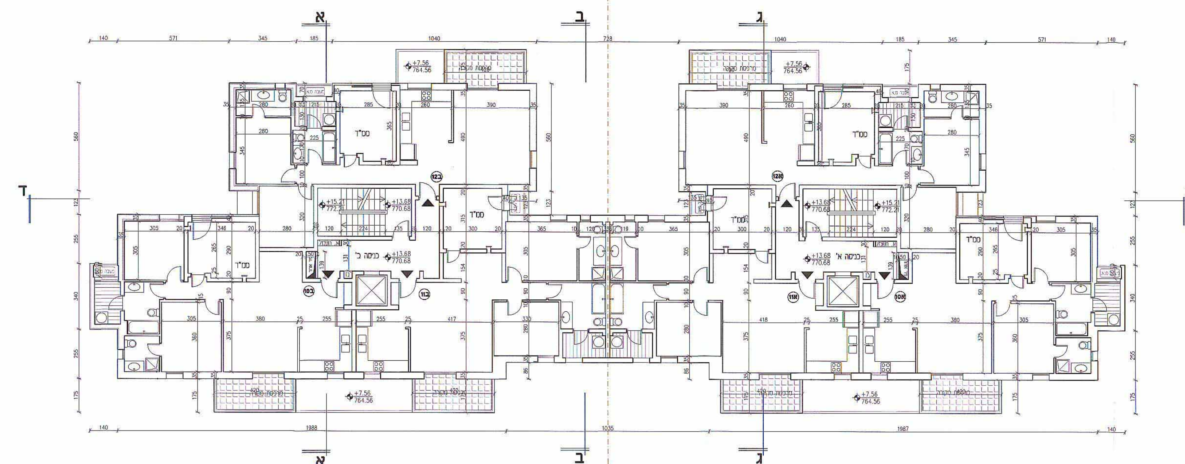
קומה 3 מפלס +13.68
