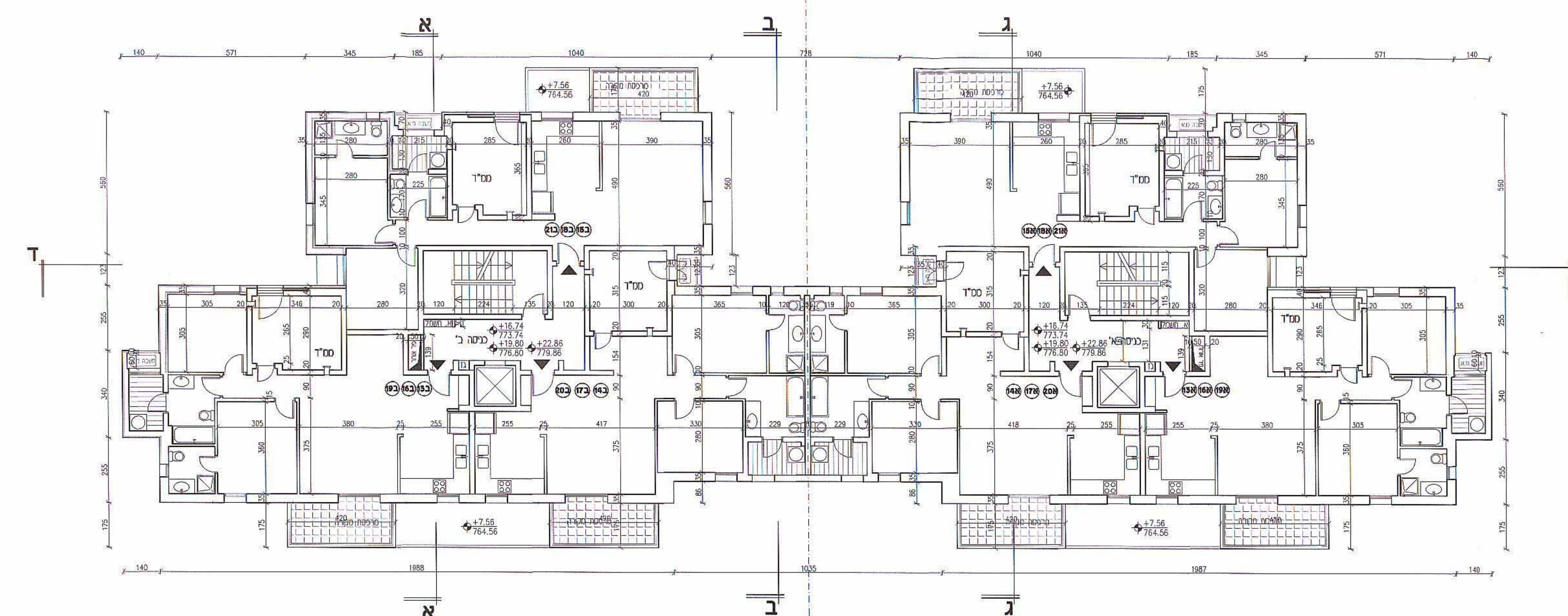
קומה טיפוסית
