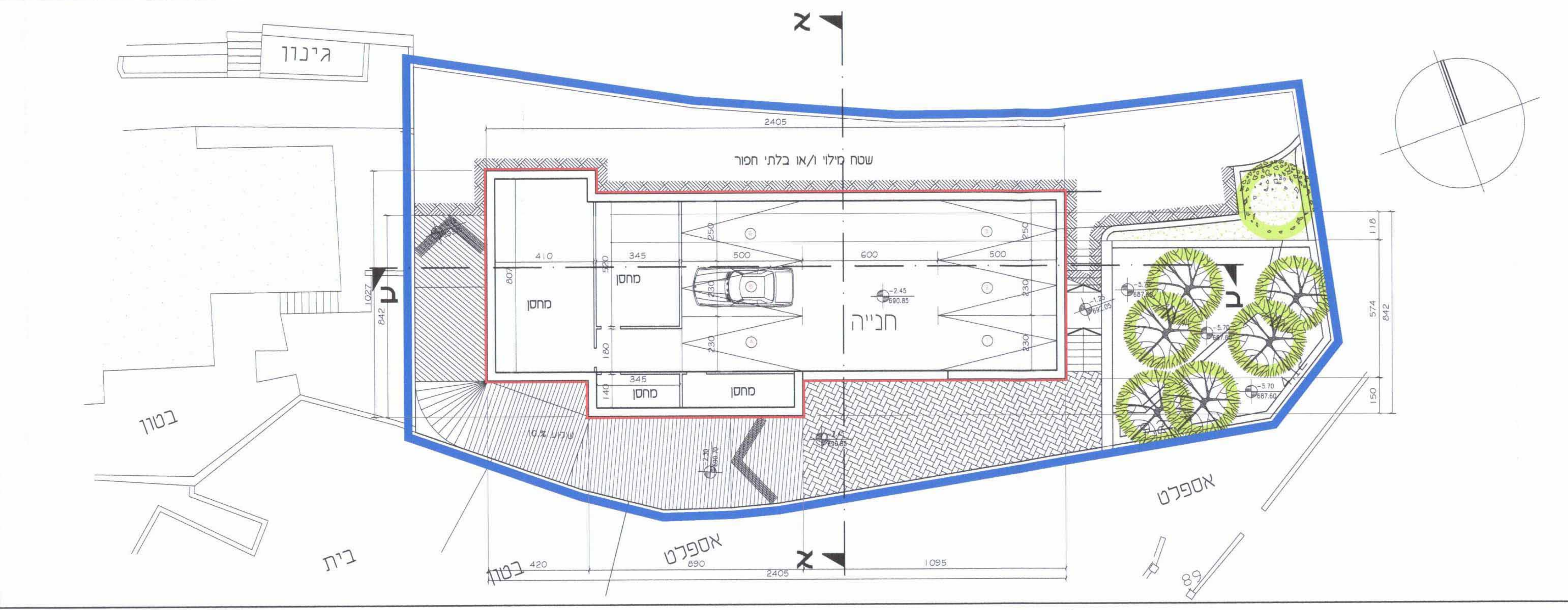
תכנית קומת חניה קנ"מ 1:100
