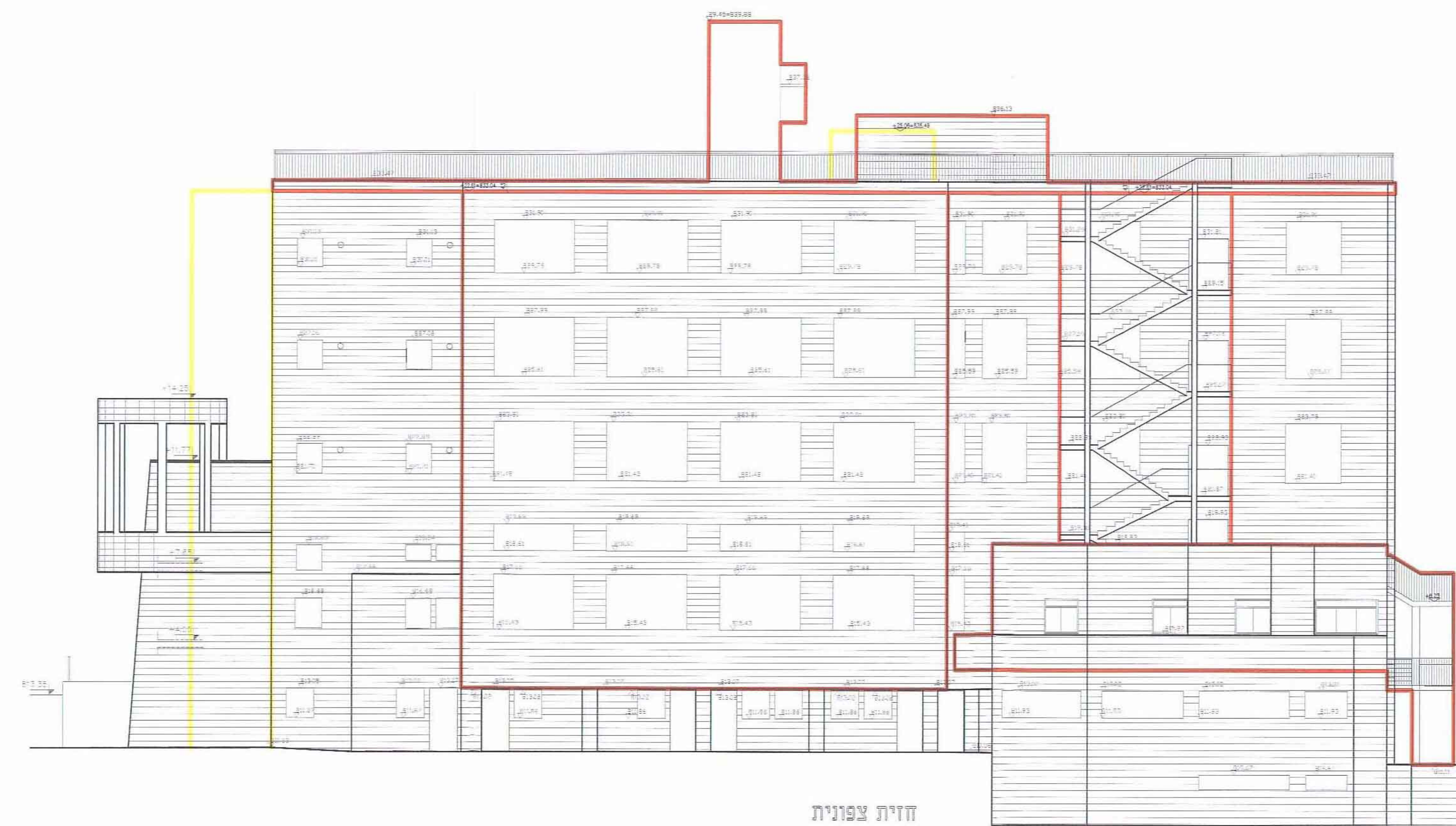
חזית צפונית קני"מ 1:100 ±0.00 = 810.43
