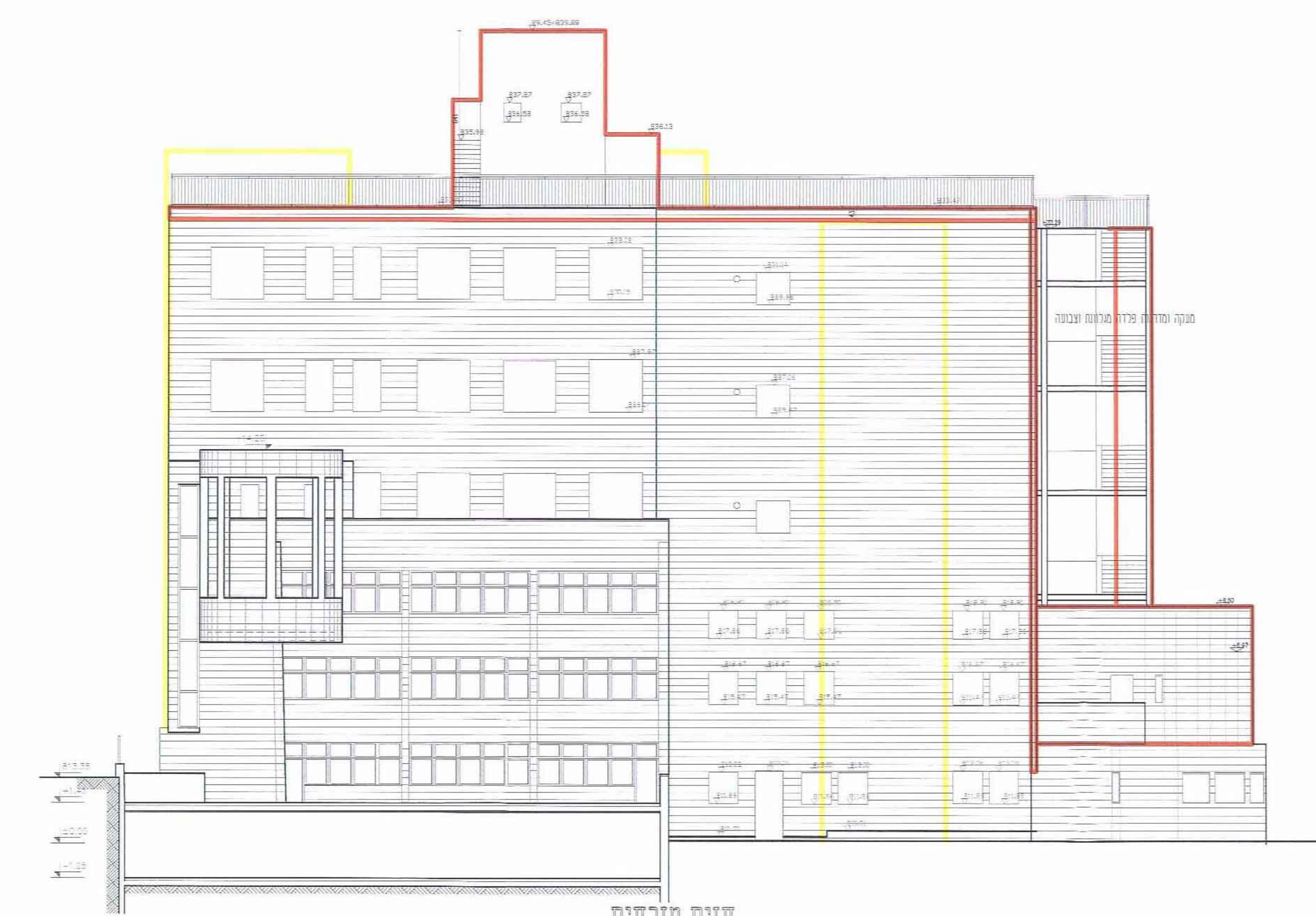
חזית מזרחית קני"מ 1:100 ±0.00 = 810.43
