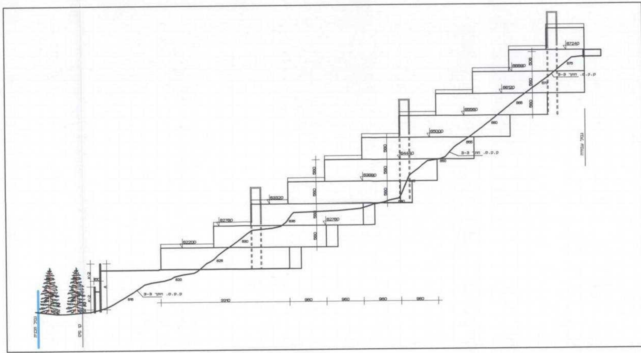
פרט חתך 2-4 עם מעליה ק.מ. 1:500
