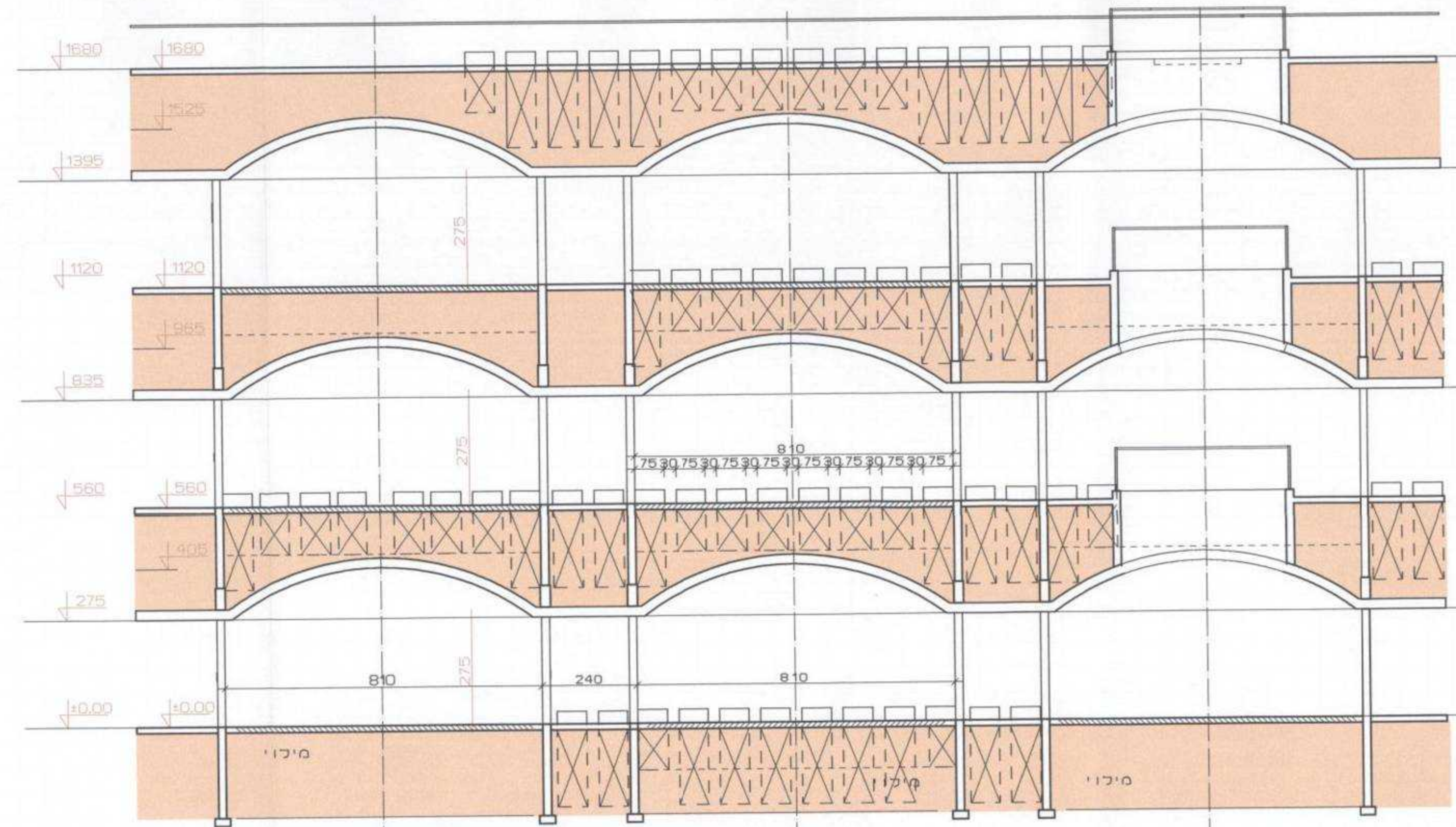
חתך אופייני לרוחב ק.מ. 1:100
