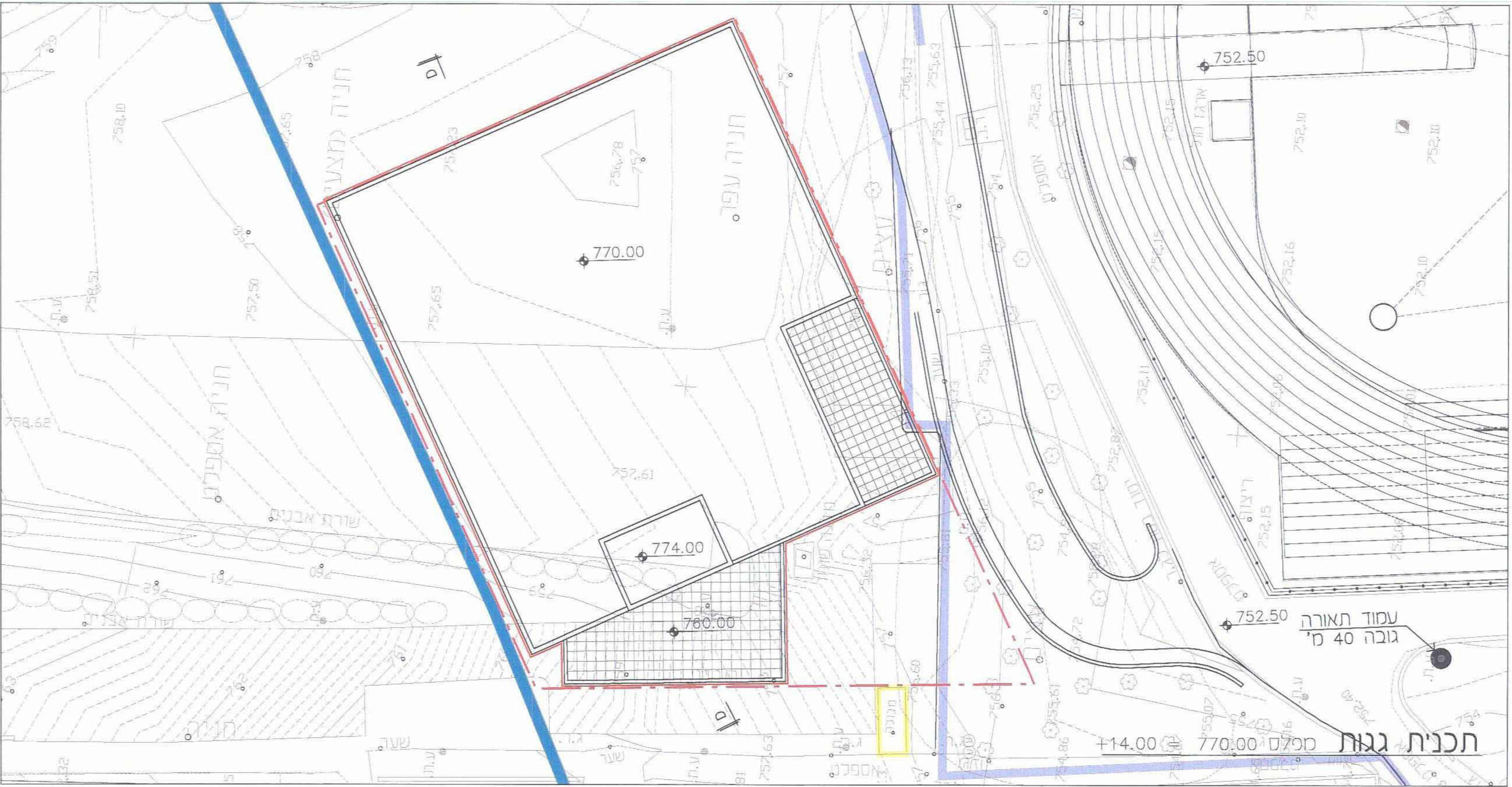
בניין מס' 4 קנ"מ 1:250
