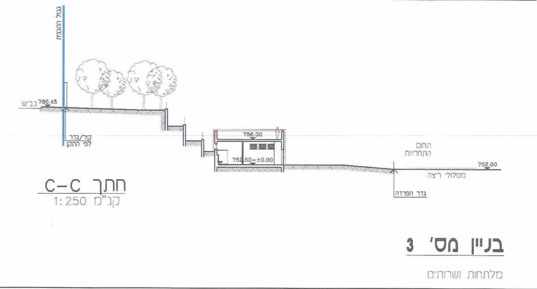
בניין מס' 3 קנ"מ 1:250
