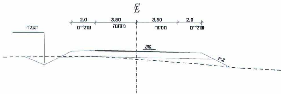
חותך טיפוס א-א לכביש מס' 5 ק.מ. - 1:50
