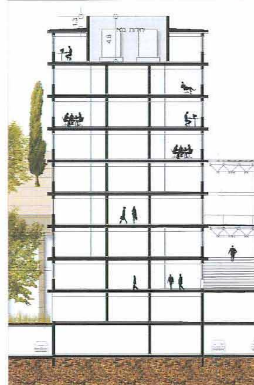
1:250 חתך מקומי מבני אטריום מיקום מערכת טכנית
