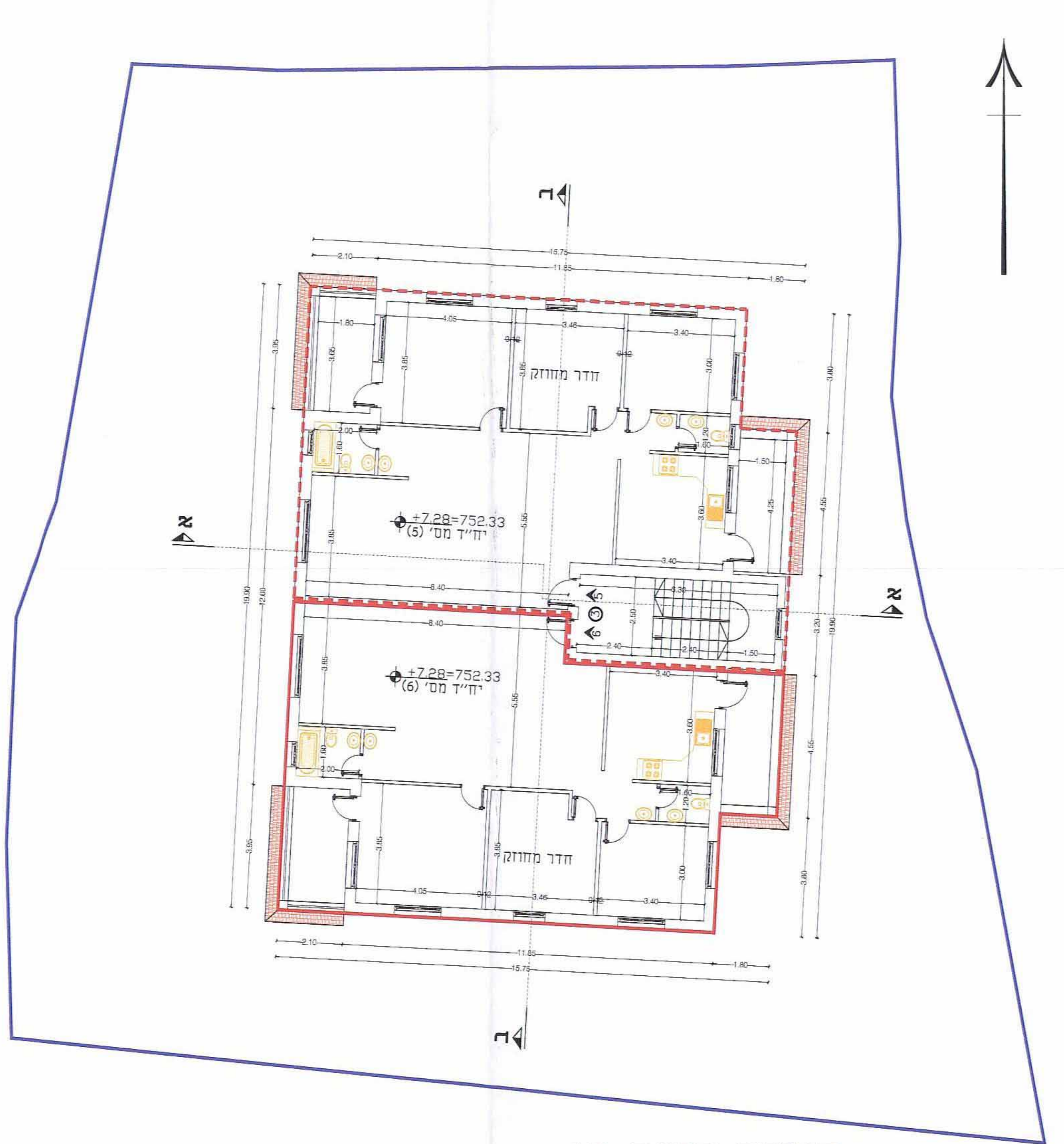
תכנית קומה ב' ק.מ. : 1:100
