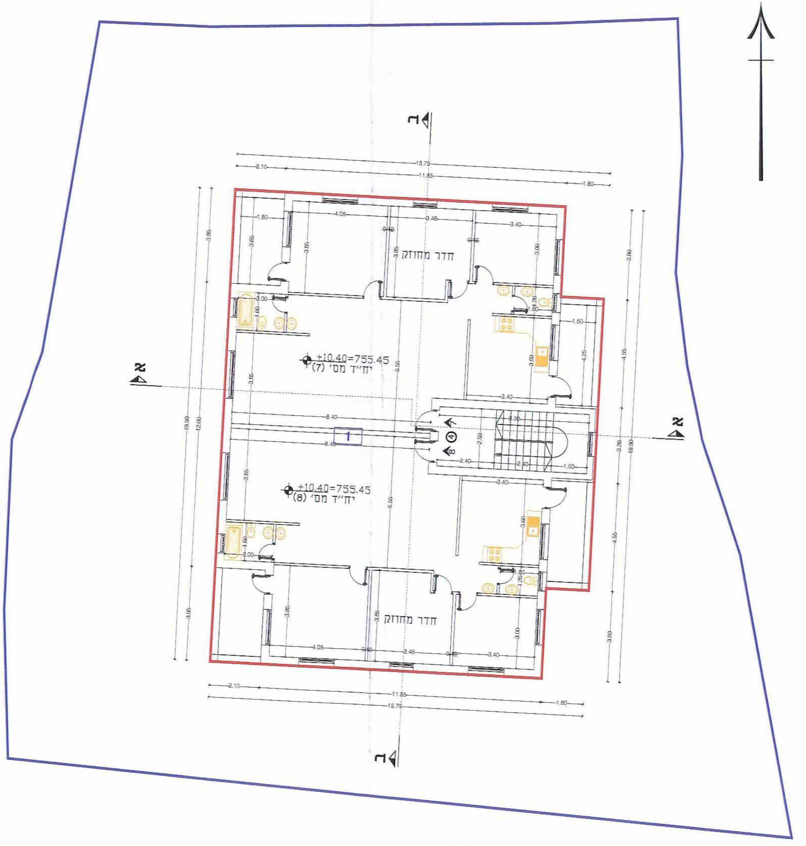
תכנית קומה ג' ק.מ. : 1:100
