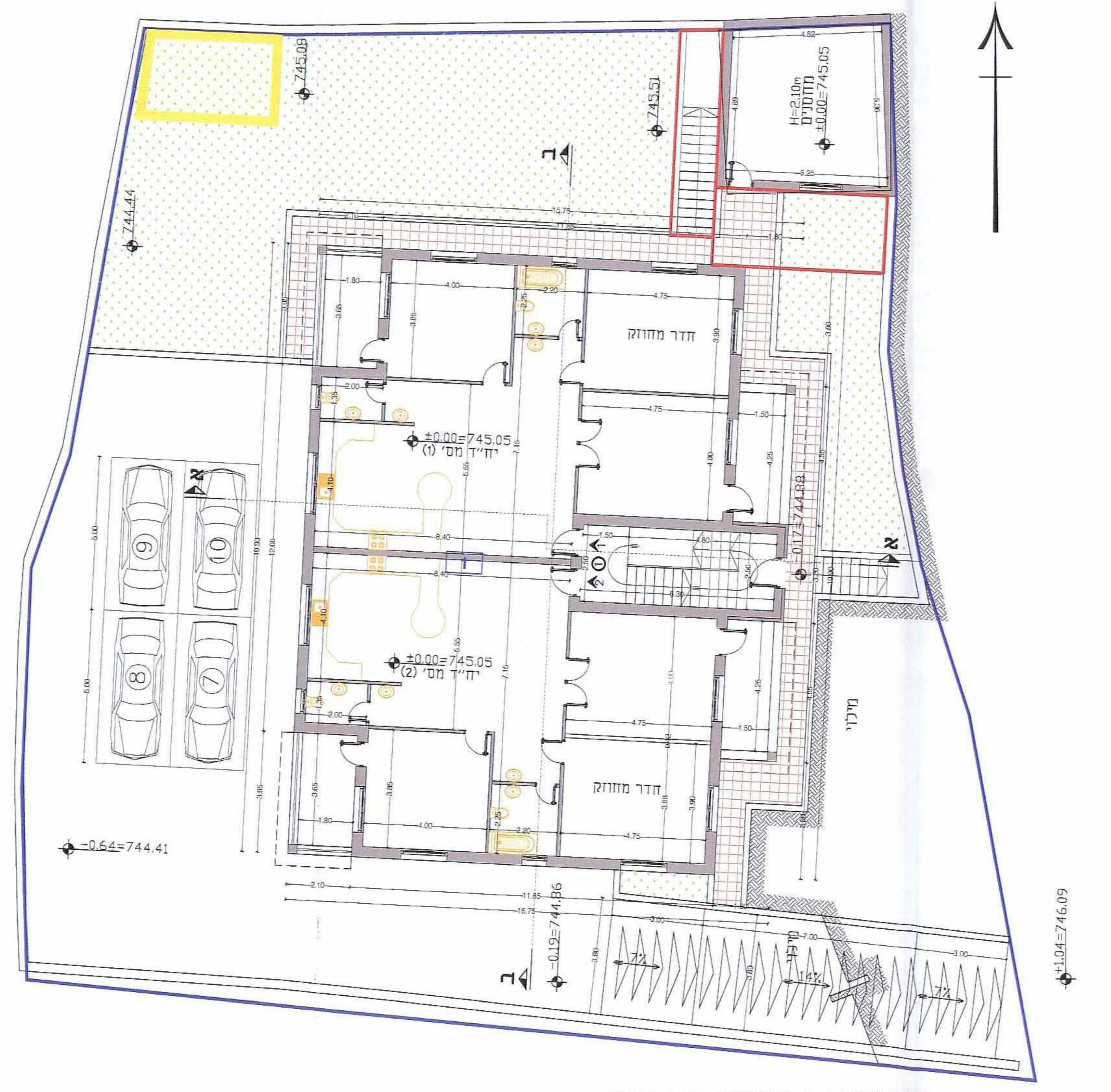
תכנית קומת קרקע ק.מ. : 1:100
