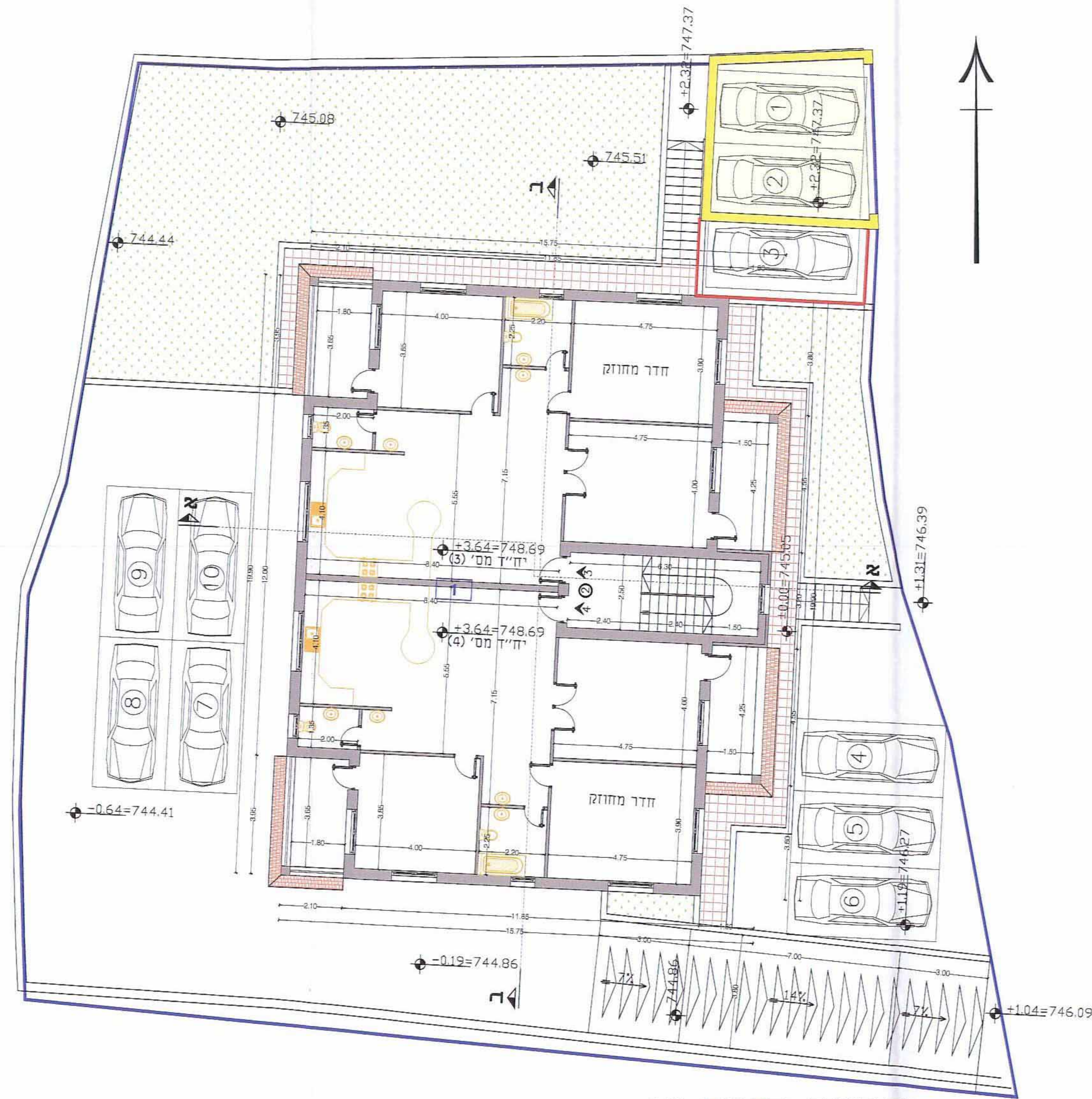
תכנית קומה א' ק.מ. : 1:100
